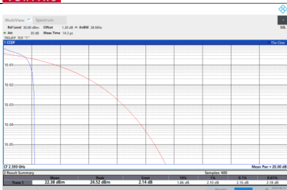
Band41-20MHz-QPSK-41490-1RB#0
