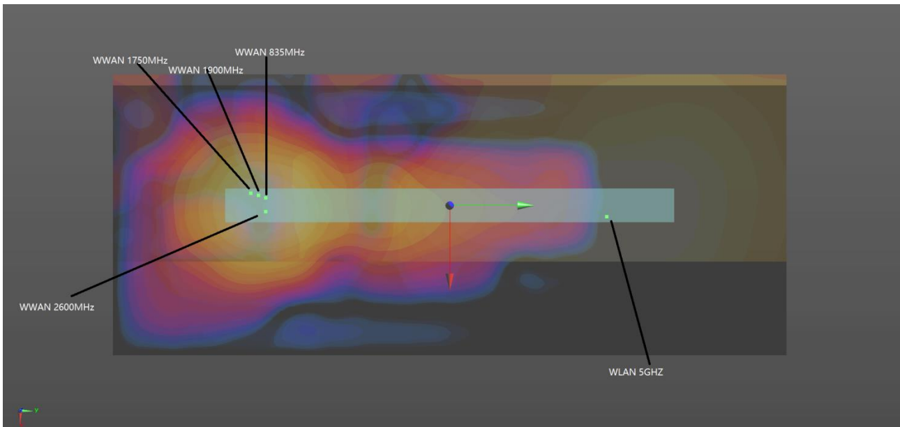
WWAN+WLAN5G _ Edge 1 0mm
