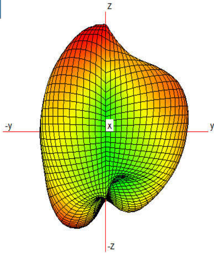
WIFI 5500MHz
