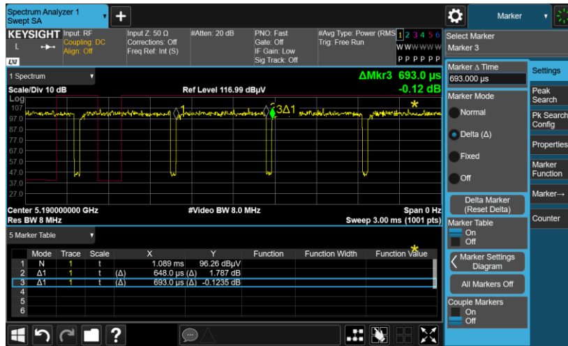
802.11n HT40
