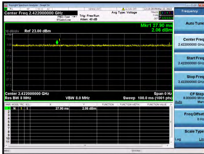
11AX40MIMO_Ant0+1_2422
