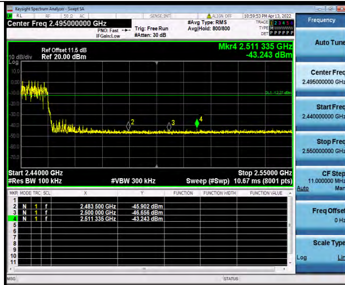
11AX40MIMO_Ant1_High_2452_26Tone_RU8
