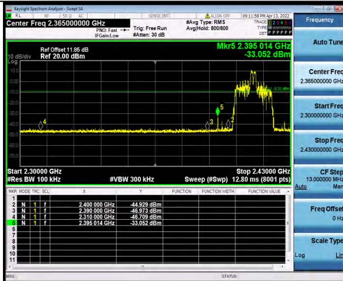
11AX20MIMO_Ant1_Low_2412_26Tone_RU8
