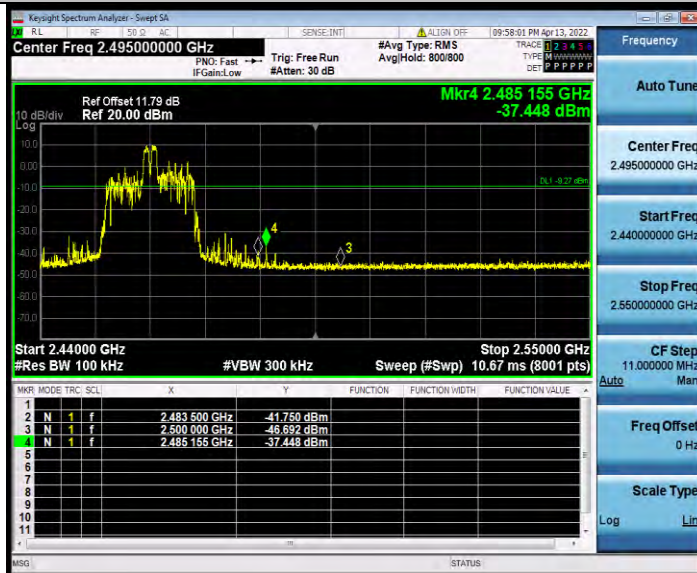
11AX20MIMO_Ant1_High_2462_26Tone_RU8
