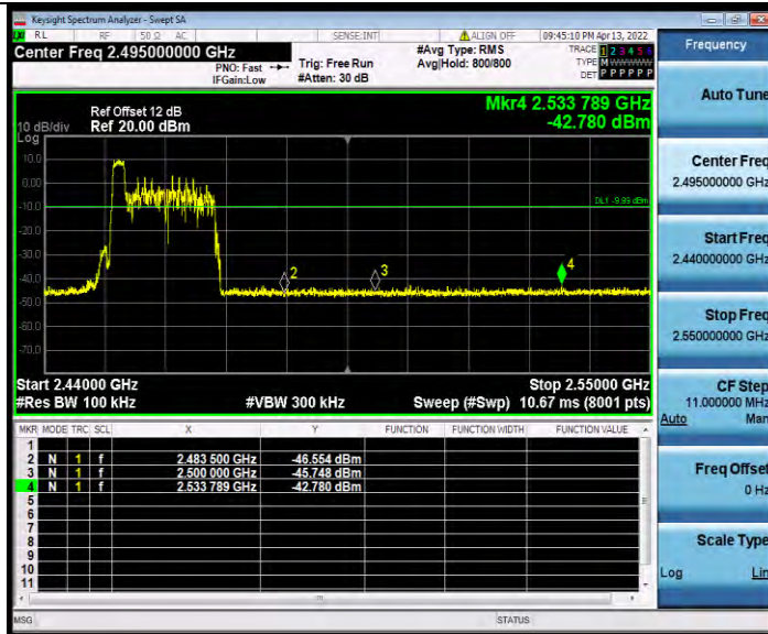
11AX20MIMO_Ant0_High_2462_26Tone_RU4
