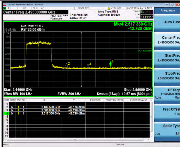
11AX20MIMO_Ant1_High_2462_26Tone_RU0
