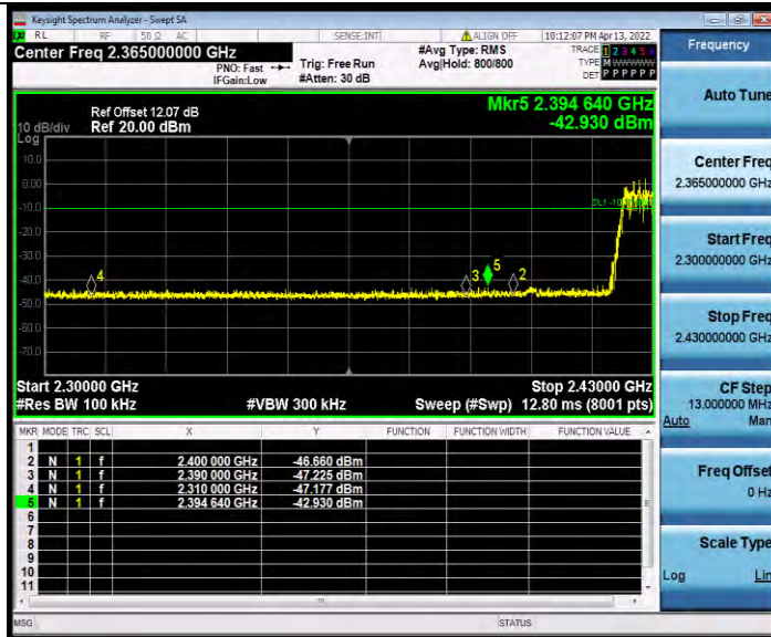
11AX40MIMO_Ant0_Low_2422_484Tone_RU65
