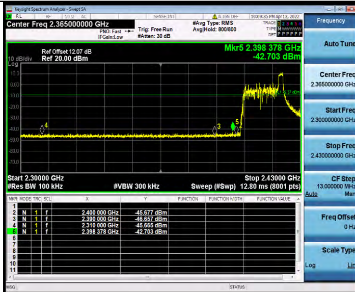
11AX40MIMO_Ant0_Low_2422_26Tone_RU17
