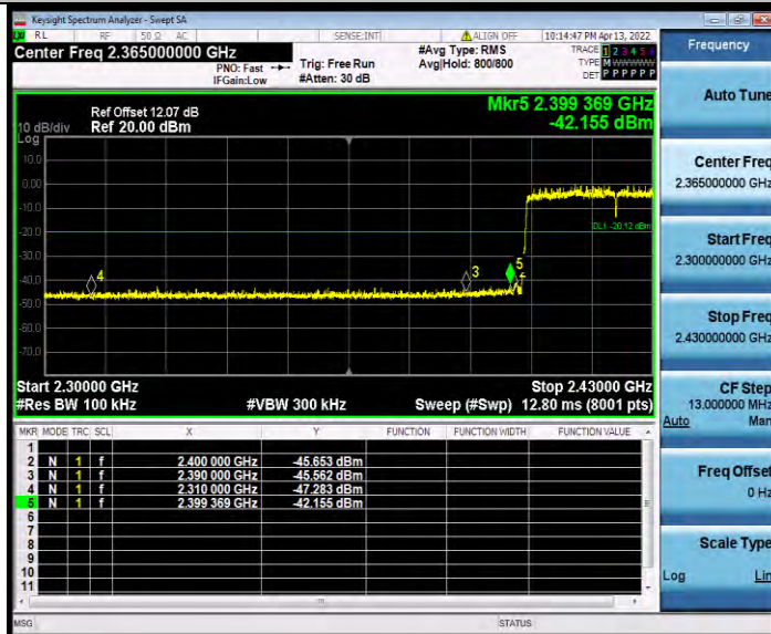
11AX40MIMO_Ant1_Low_2422_26Tone_RU0
