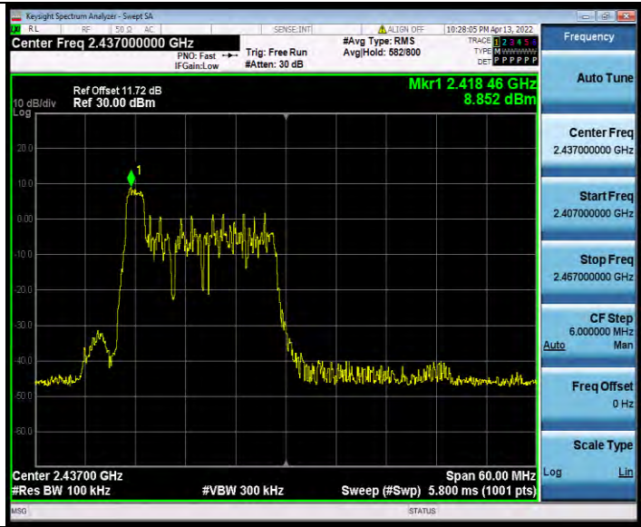
11AX40MIMO_Ant0_2437_26Tone_RU8
