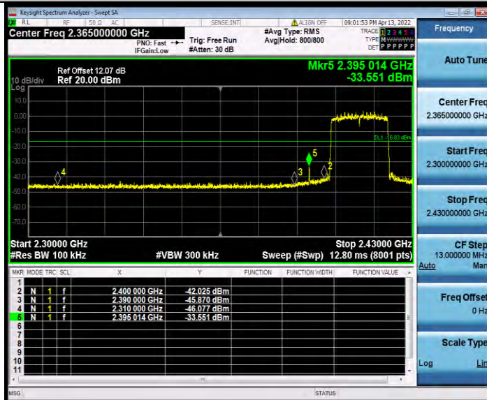
11AX20MIMO_Ant1_Low_2412_26Tone_RU0
