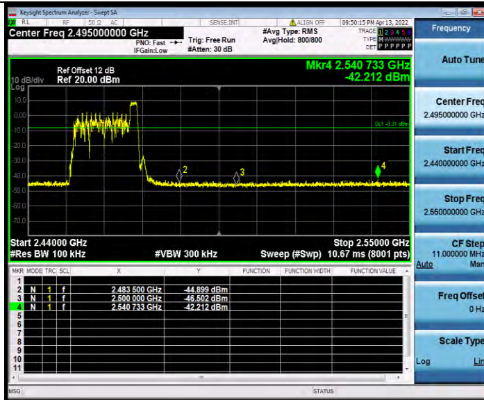
11AX20MIMO_Ant0_High_2462_242Tone_RU61
