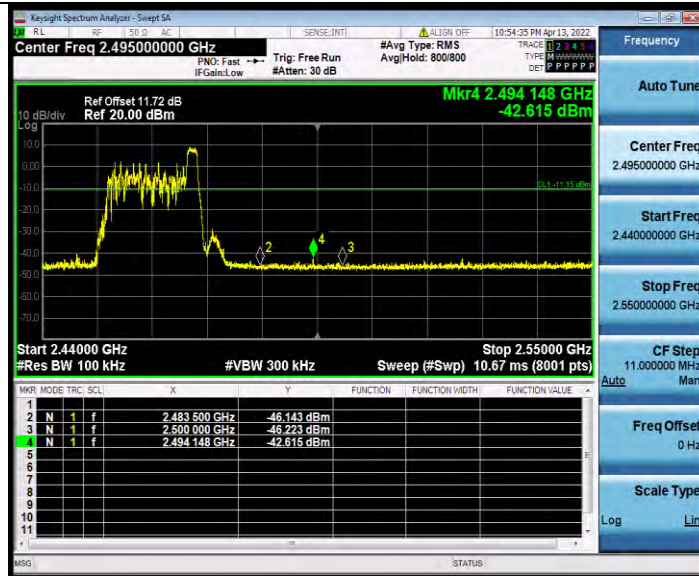
11AX40MIMO_Ant0_High_2452_484Tone_RU65
