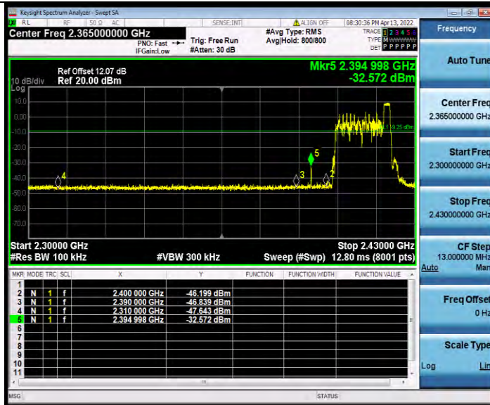
11AX20MIMO_Ant0_Low_2412_242Tone_RU61
