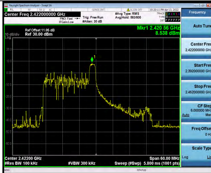
11AX40MIMO_Ant1_2422_26Tone_RU17
