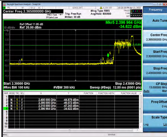
11AX40MIMO_Ant1_Low_2422_26Tone_RU17
