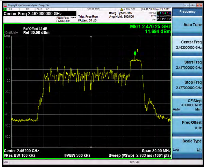
11AX20MIMO_Ant0_2462_242Tone_RU61
