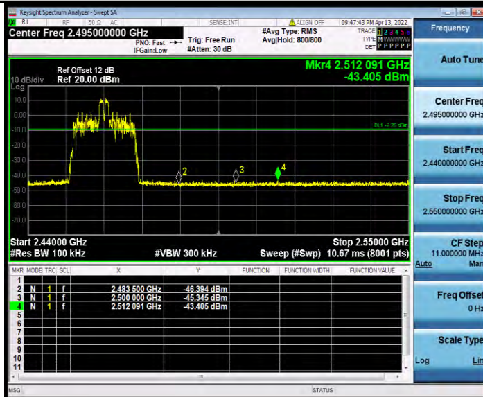
11AX20MIMO_Ant0_High_2462_26Tone_RU8
