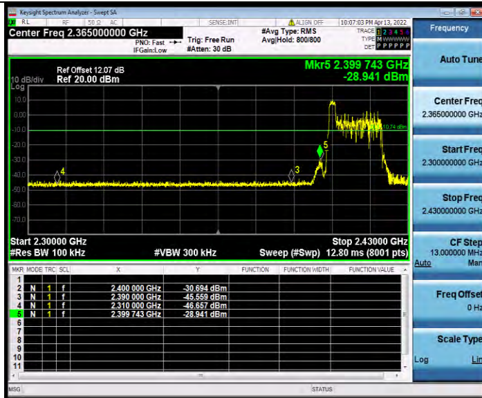
11AX40MIMO_Ant0_Low_2422_26Tone_RU8
