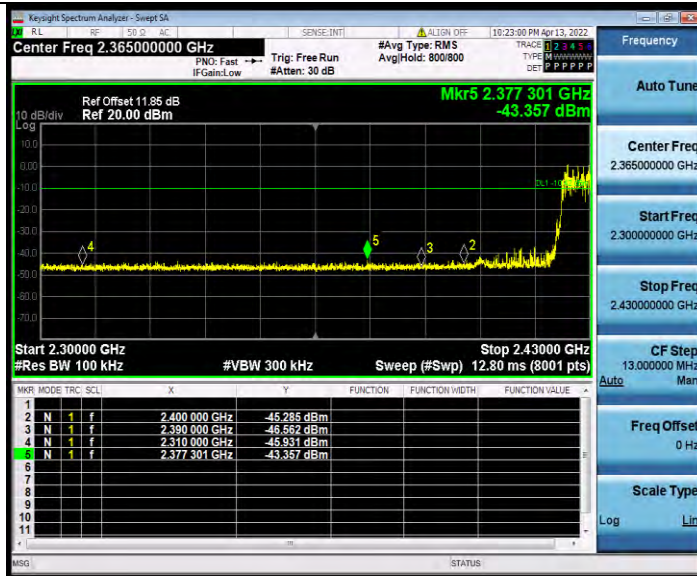
11AX40MIMO_Ant1_Low_2422_484Tone_RU65
