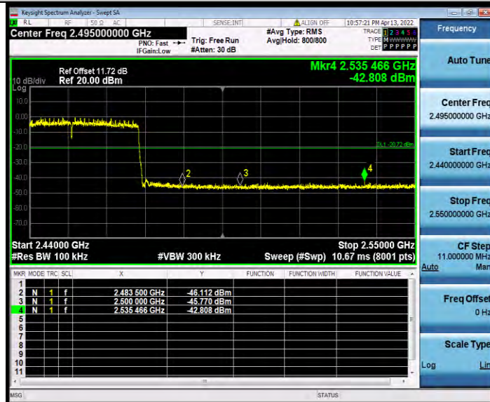
11AX40MIMO_Ant1_High_2452_26Tone_RU0
