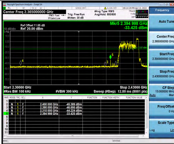
11AX20MIMO_Ant1_Low_2412_242Tone_RU61
