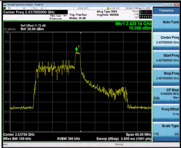
11AX40MIMO_Ant0_2437_26Tone_RU17
