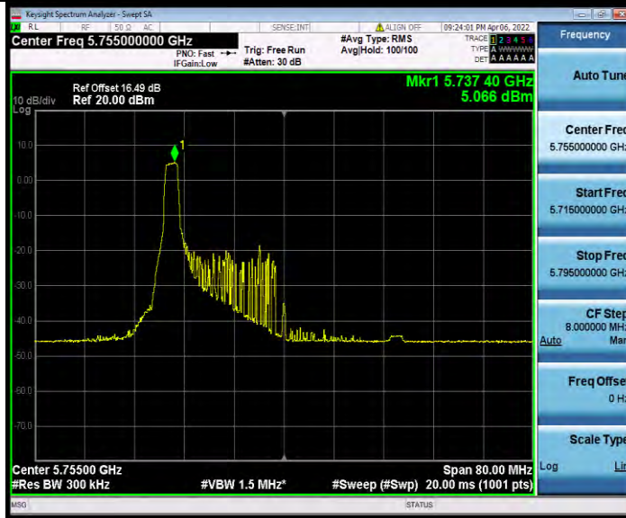
11AX40MIMO_Ant1_5755_26Tone_RU8
