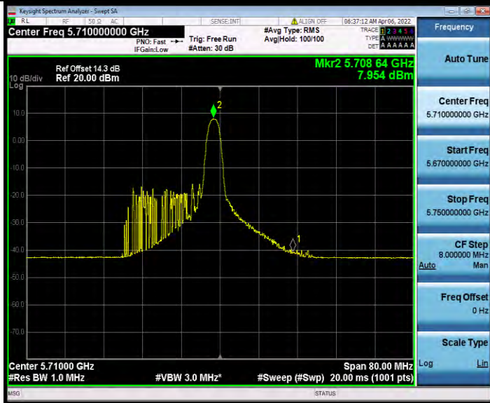
11AX40MIMO_Ant0_5710_UNII-2C_26Tone_RU17
