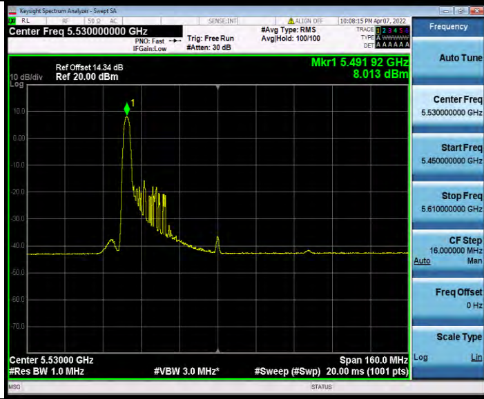
11AX80MIMO_Ant0_5530_26Tone_RU18
