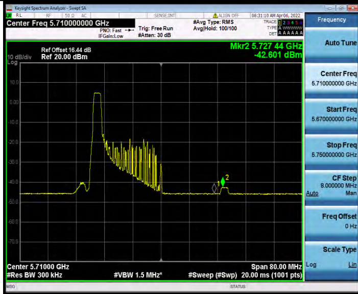
11AX40MIMO_Ant0_5710_UNII-3_26Tone_RU8
