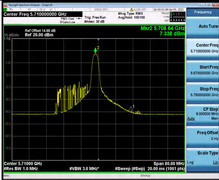
11AX40MIMO_Ant1_5710_UNII-2C_26Tone_RU17
