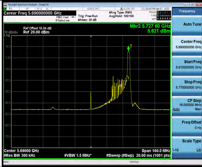
11AX80MIMO_Ant1_5690_UNII-3_996Tone_RU67
