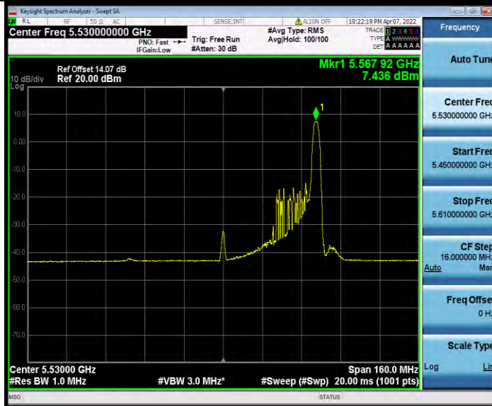
11AX80MIMO_Ant1_5530_996Tone_RU67
