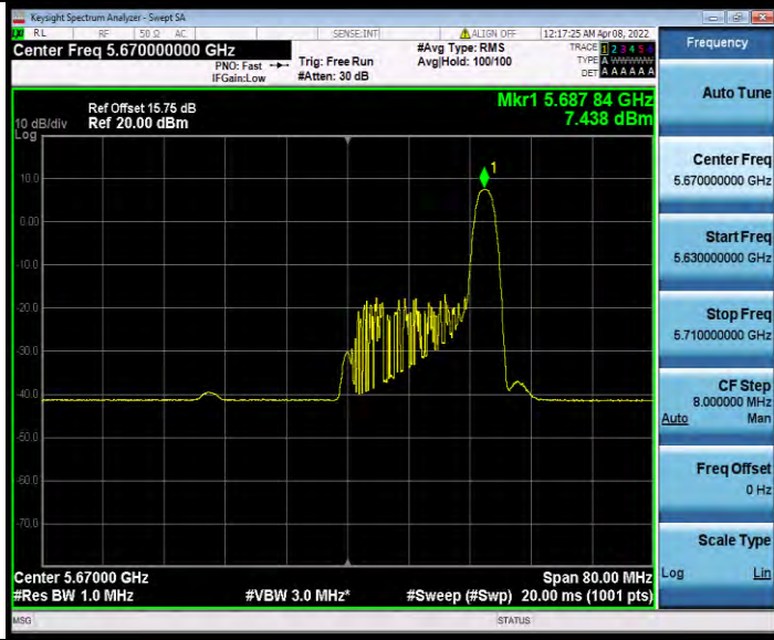
11AX40MIMO_Ant1_5670_484Tone_RU65
