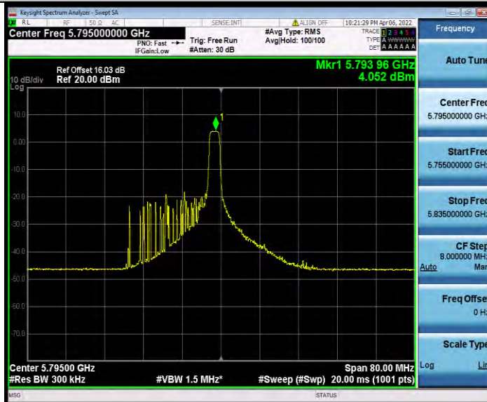
11AX40MIMO_Ant0_5795_26Tone_RU17
