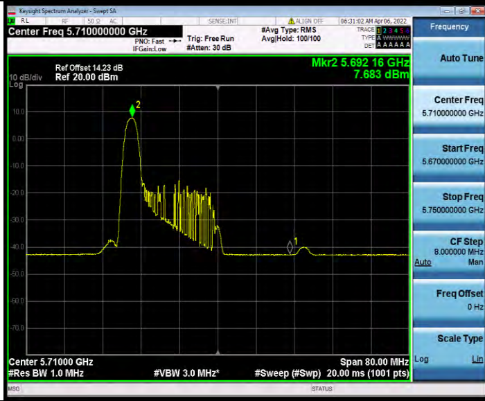
11AX40MIMO_Ant0_5710_UNII-2C_26Tone_RU8
