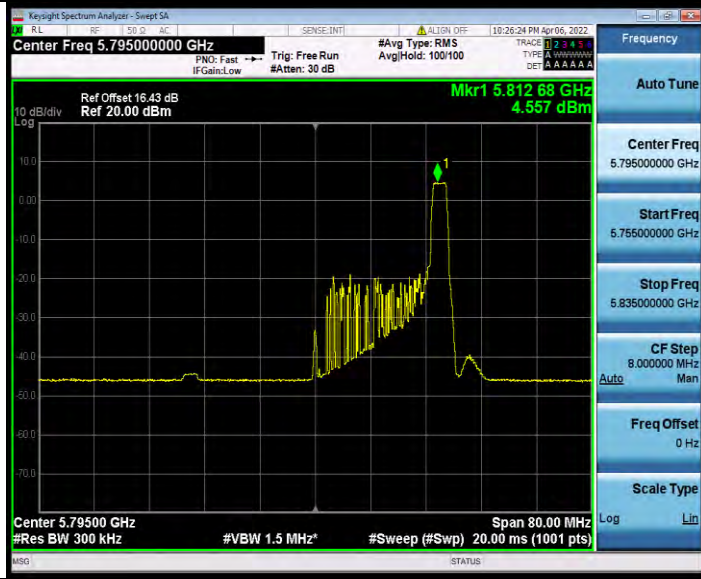
11AX40MIMO_Ant0_5795_484Tone_RU65
