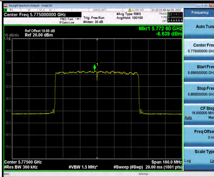
11AX80MIMO_Ant1_5775_996Tone_RU67
