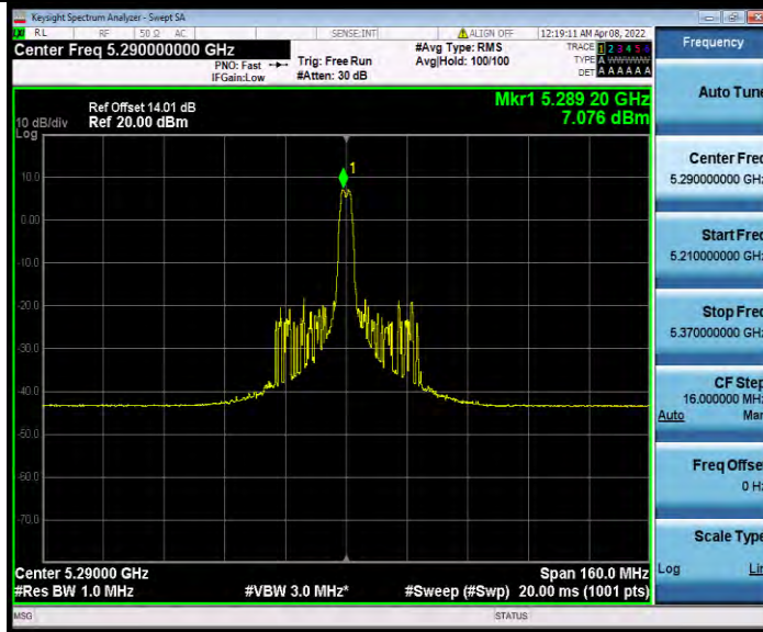
11AX80MIMO_Ant0_5290_996Tone_RU67
