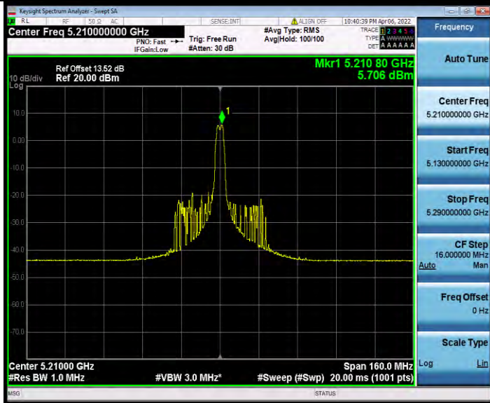
11AX80MIMO_Ant0_5210_26Tone_RU36
