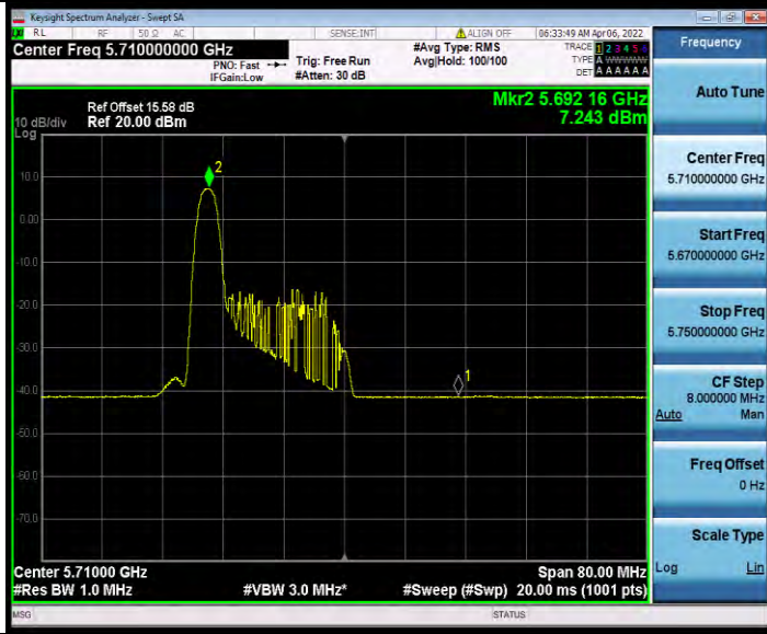
11AX40MIMO_Ant1_5710_UNII-2C_26Tone_RU8
