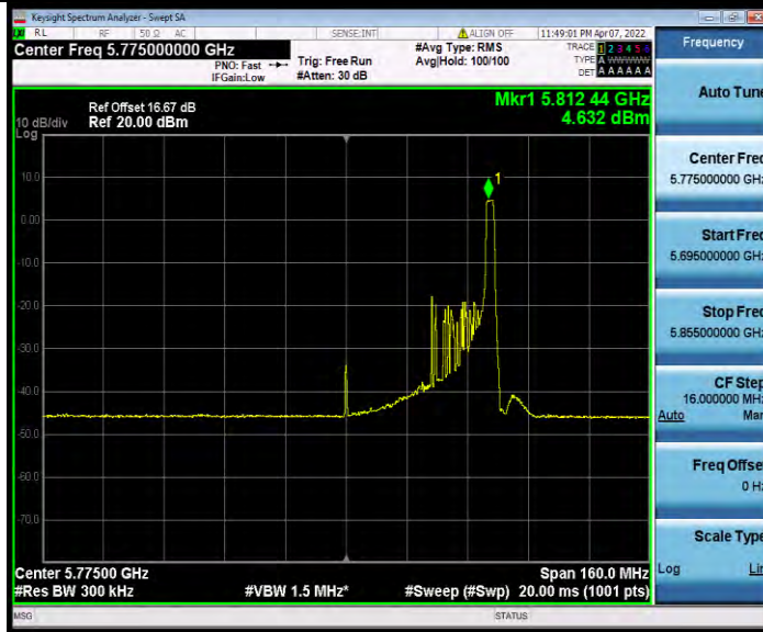
11AX80MIMO_Ant0_5775_996Tone_RU67
