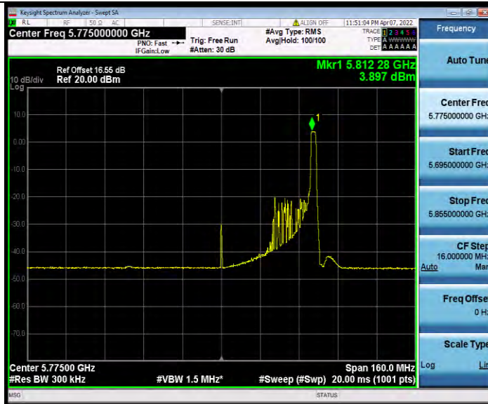
11AX80MIMO_Ant1_5775_996Tone_RU67
