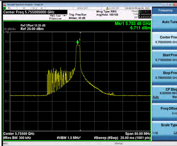
11AX40MIMO_Ant0_5755_26Tone_RU17
