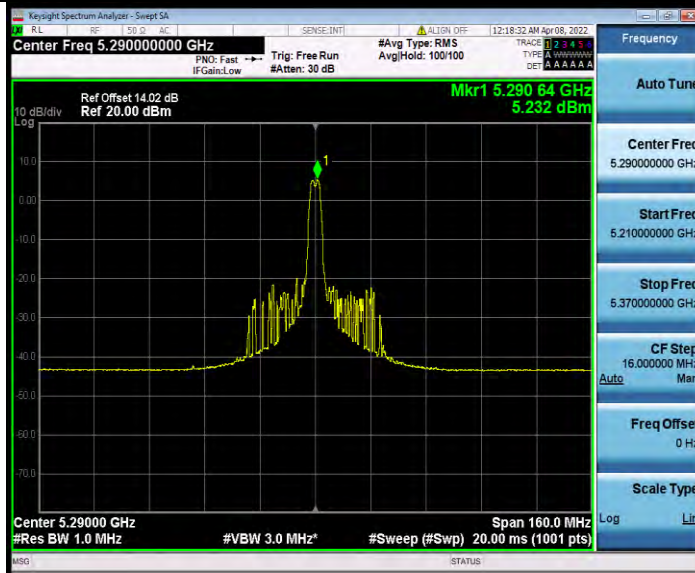
11AX80MIMO_Ant0_5290_26Tone_RU36
