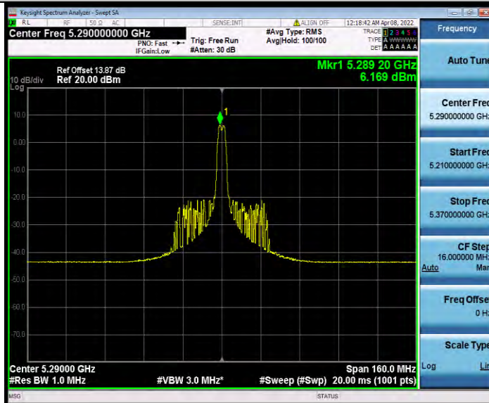
11AX80MIMO_Ant1_5290_26Tone_RU36
