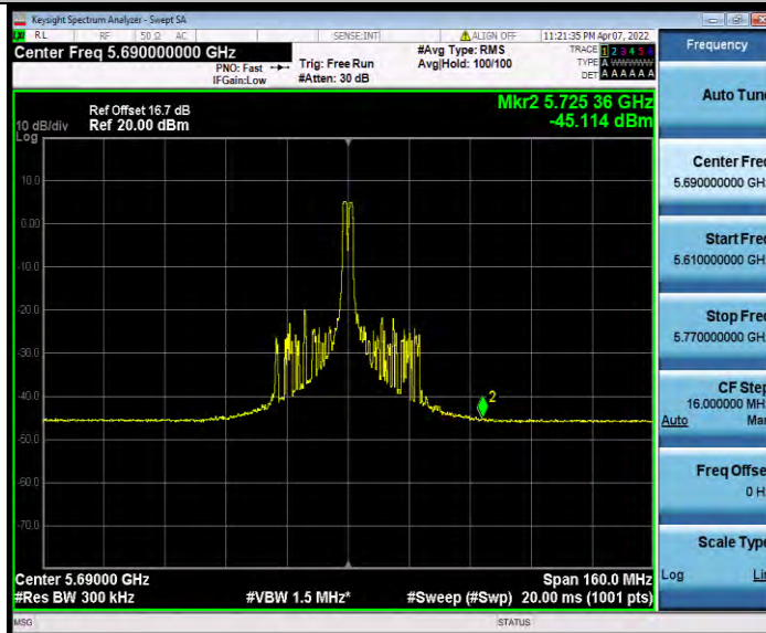
11AX80MIMO_Ant0_5690_UNII-3_26Tone_RU36
