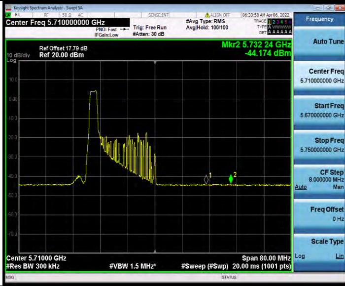
11AX40MIMO_Ant1_5710_UNII-3_26Tone_RU8
