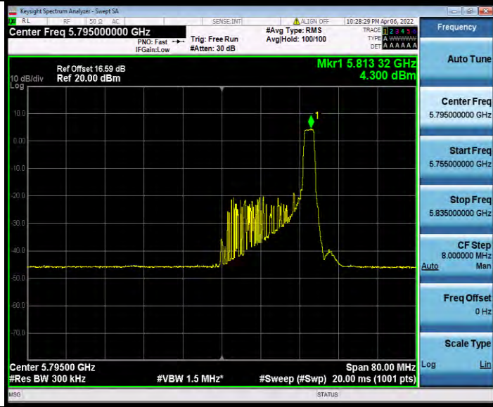
11AX40MIMO_Ant1_5795_484Tone_RU65
