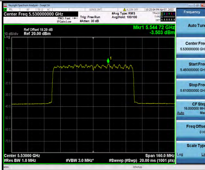
11AX80MIMO_Ant1_5530_26Tone_RU0
