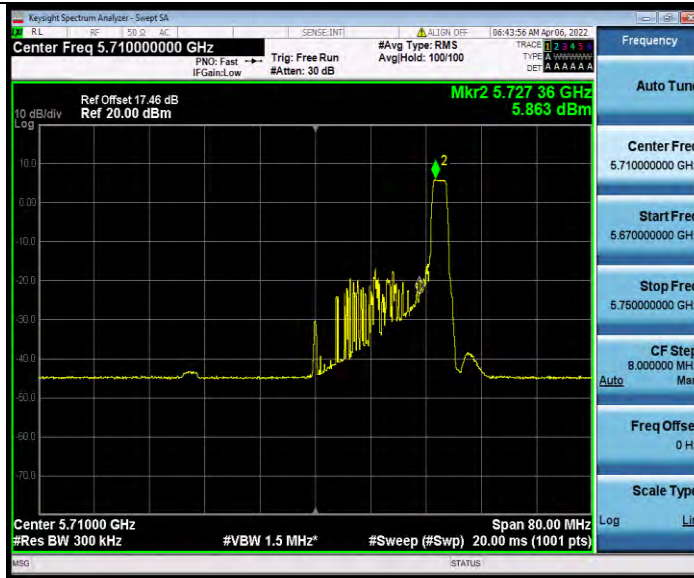
11AX40MIMO_Ant0_5710_UNII-3_484Tone_RU65
