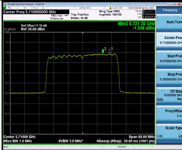
11AX40MIMO_Ant0_5710_UNII-3_26Tone_RU0
