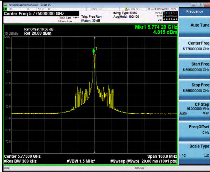
11AX80MIMO_Ant1_5775_26Tone_RU36
