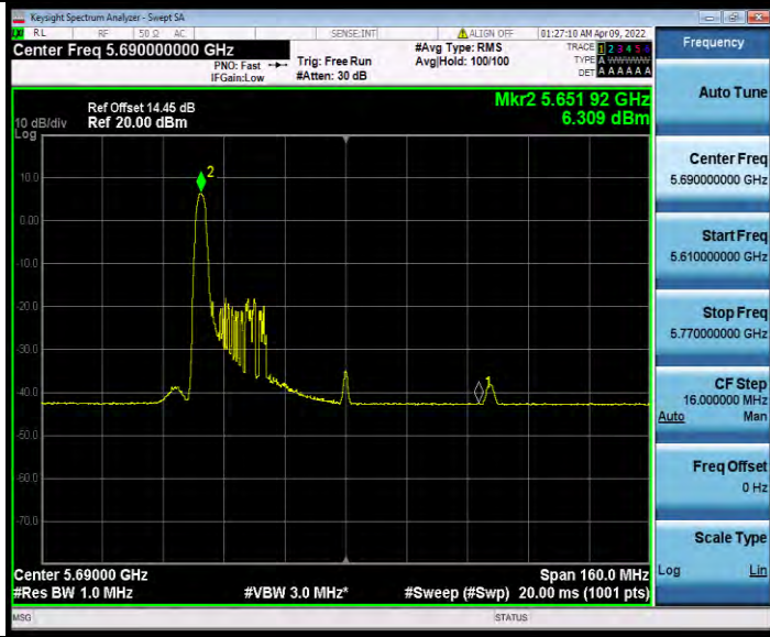
11AX80MIMO_Ant0_5690_UNII-2C_26Tone_RU18
