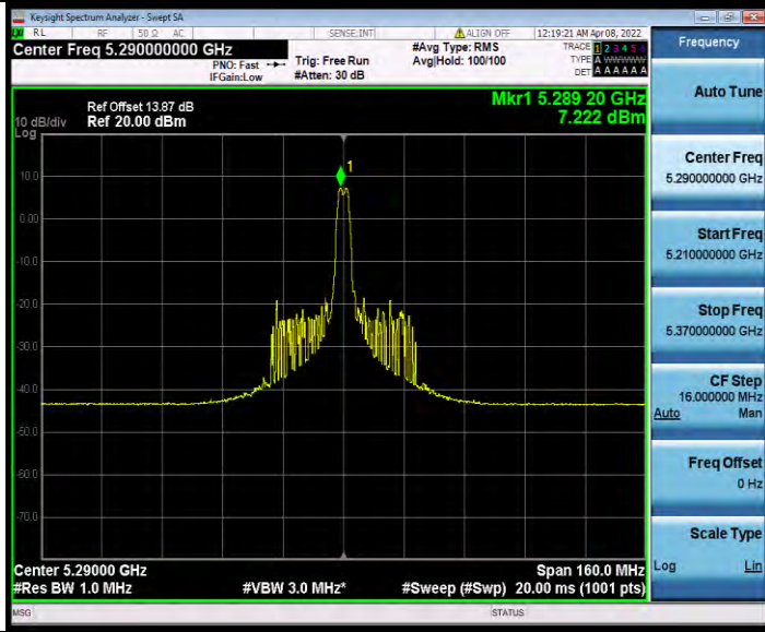
11AX80MIMO_Ant1_5290_996Tone_RU67
