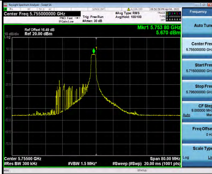
11AX40MIMO_Ant1_5755_26Tone_RU17
