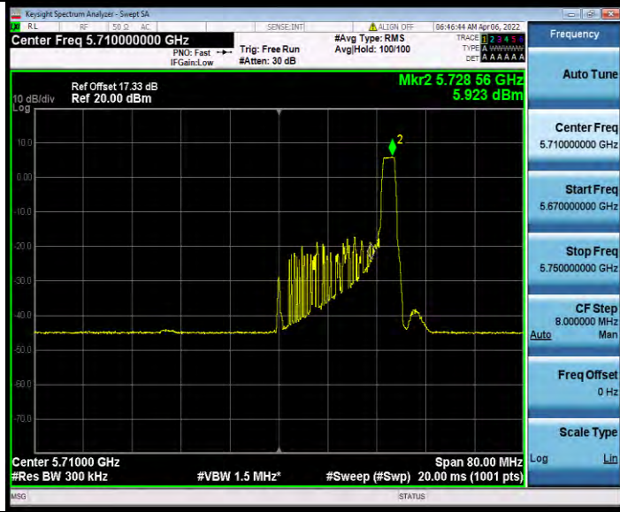
11AX40MIMO_Ant1_5710_UNII-3_484Tone_RU65
