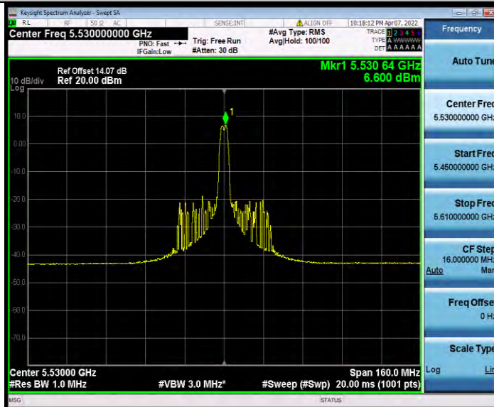
11AX80MIMO_Ant1_5530_26Tone_RU36
