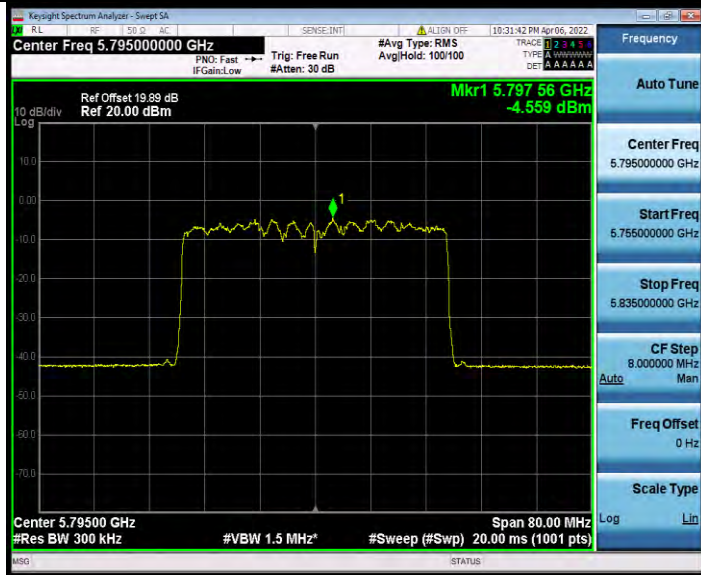
11AX40MIMO_Ant1_5795_26Tone_RU0
