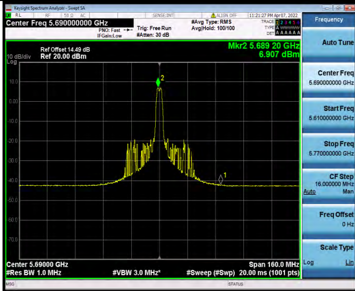
11AX80MIMO_Ant0_5690_UNII-2C_26Tone_RU36
