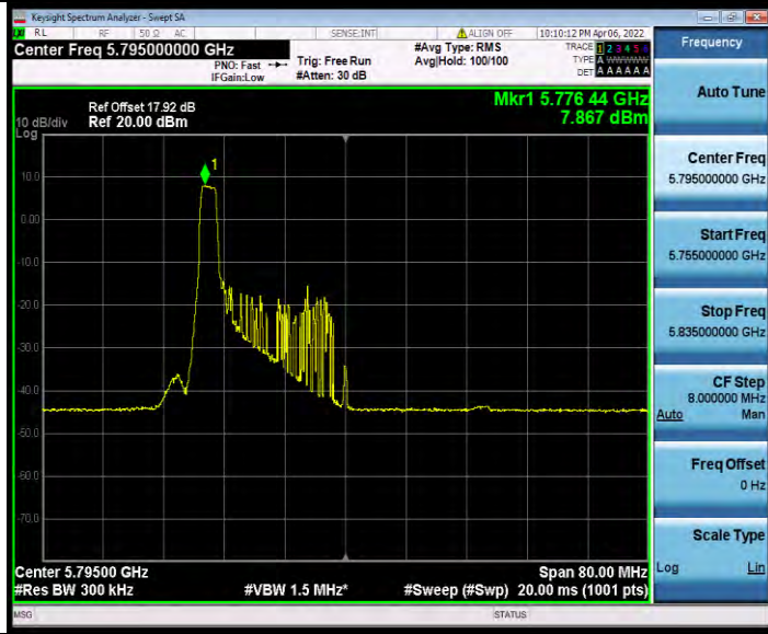
11AX40MIMO_Ant1_5795_26Tone_RU8
