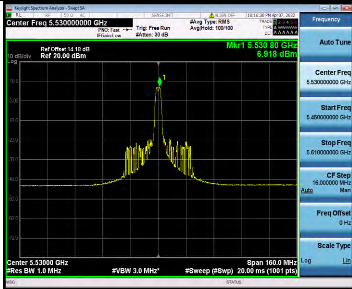
11AX80MIMO_Ant0_5530_26Tone_RU36
