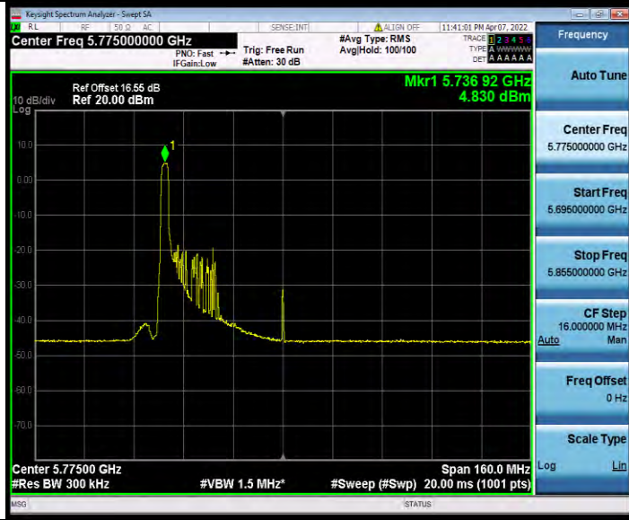
11AX80MIMO_Ant1_5775_26Tone_RU18
