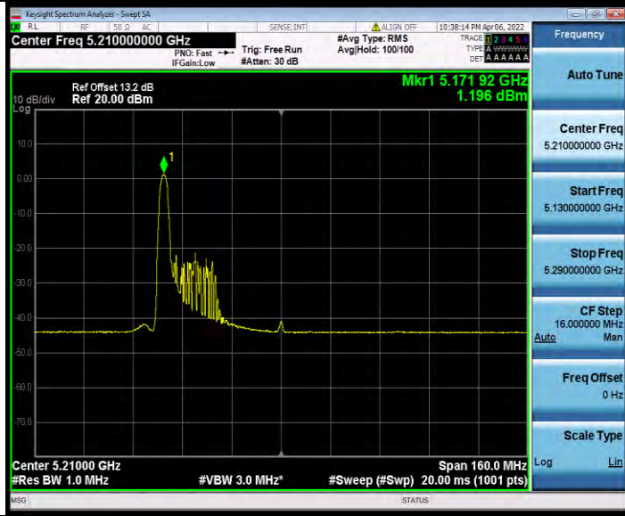
11AX80MIMO_Ant1_5210_26Tone_RU18
