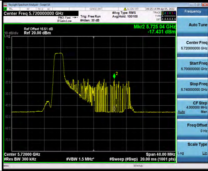
11AX20MIMO_Ant0_5720_UNII-3_26Tone_RU4
