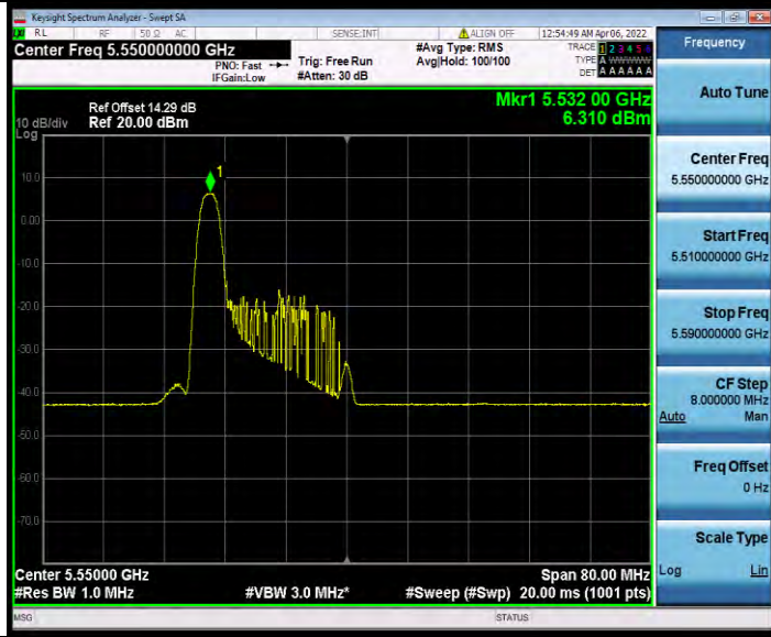
11AX40MIMO_Ant0_5550_26Tone_RU8
