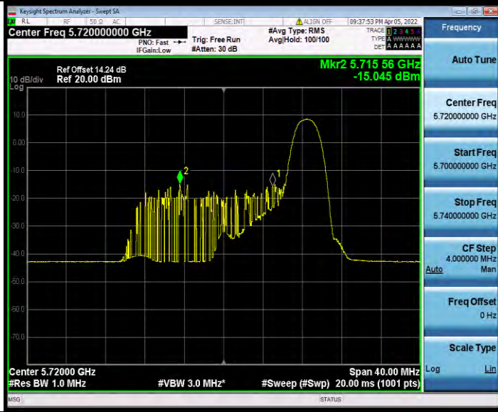
11AX20MIMO_Ant0_5720_UNII-2C_242Tone_RU61
