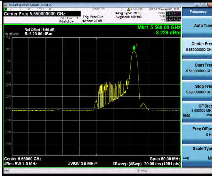
11AX40MIMO_Ant1_5550_484Tone_RU65
