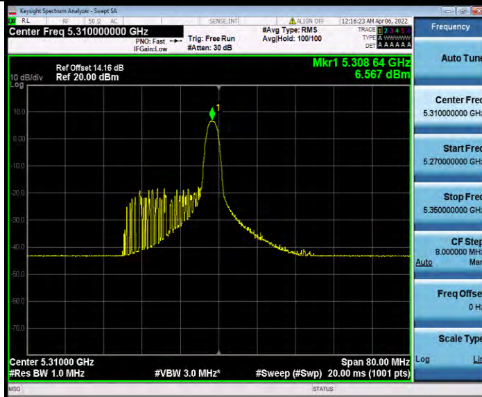
11AX40MIMO_Ant0_5310_26Tone_RU17
