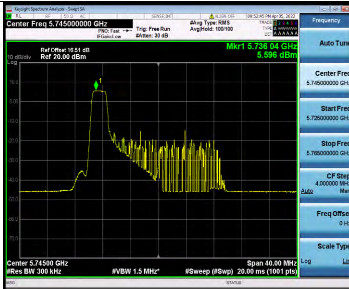
11AX20MIMO_Ant1_5745_26Tone_RU4
