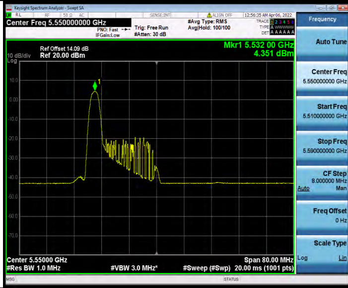
11AX40MIMO_Ant1_5550_26Tone_RU8
