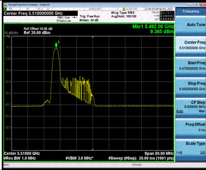
11AX40MIMO_Ant0_5510_26Tone_RU8
