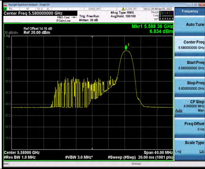
11AX20MIMO_Ant1_5580_242Tone_RU61
