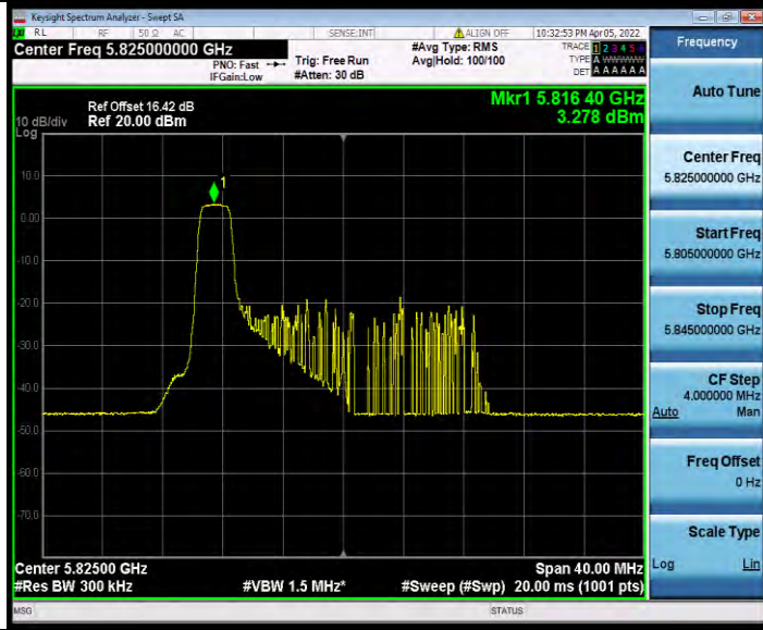
11AX20MIMO_Ant1_5825_26Tone_RU4
