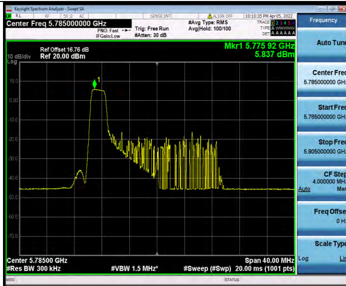
11AX20MIMO_Ant0_5785_26Tone_RU4
