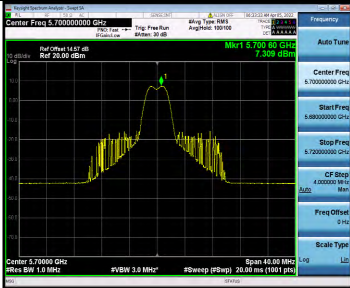
11AX20MIMO_Ant0_5700_26Tone_RU8
