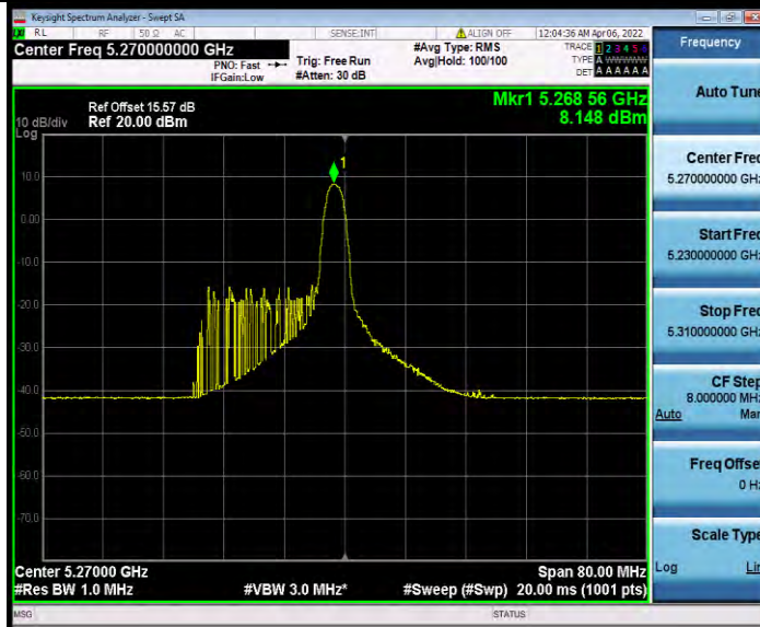
11AX40MIMO_Ant1_5270_26Tone_RU17
