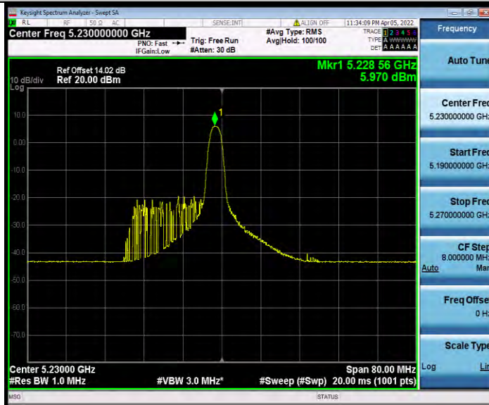
11AX40MIMO_Ant1_5230_26Tone_RU17
