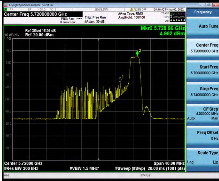
11AX20MIMO_Ant1_5720_UNII-3_242Tone_RU61
