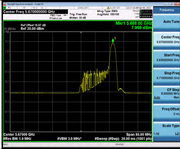
11AX40MIMO_Ant0_5670_484Tone_RU65
