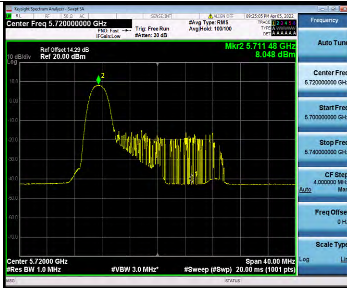
11AX20MIMO_Ant0_5720_UNII-2C_26Tone_RU4
