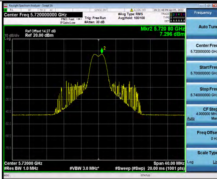
11AX20MIMO_Ant0_5720_UNII-2C_26Tone_RU8
