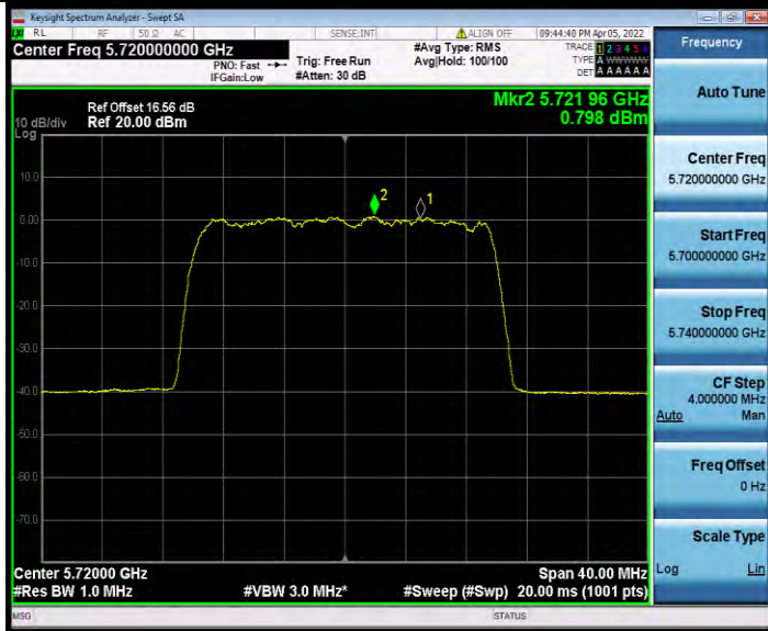
11AX20MIMO_Ant1_5720_UNII-2C_26Tone_RU0
