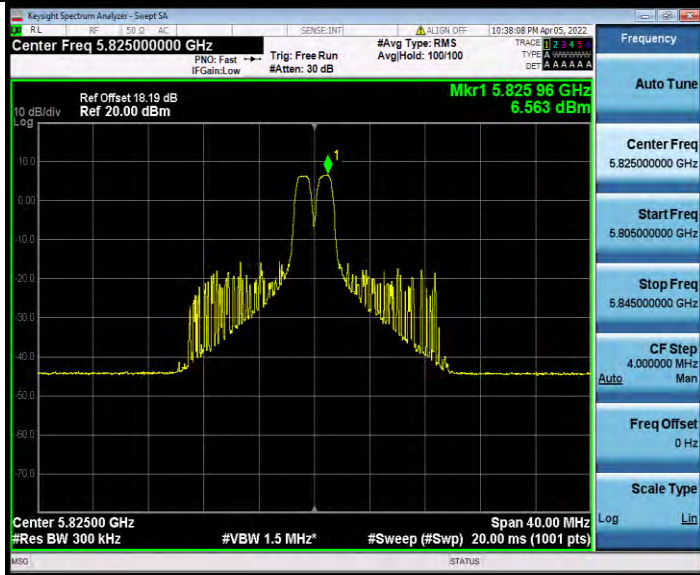
11AX20MIMO_Ant0_5825_26Tone_RU8
