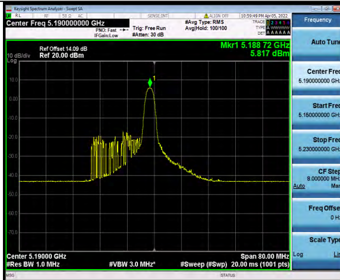
11AX40MIMO_Ant0_5190_26Tone_RU17
