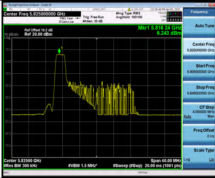
11AX20MIMO_Ant0_5825_26Tone_RU4
