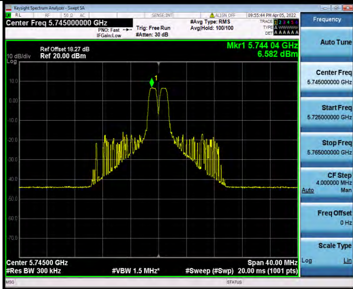
11AX20MIMO_Ant0_5745_26Tone_RU8
