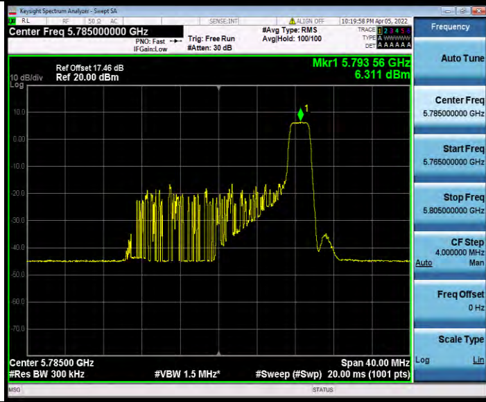
11AX20MIMO_Ant0_5785_242Tone_RU61
