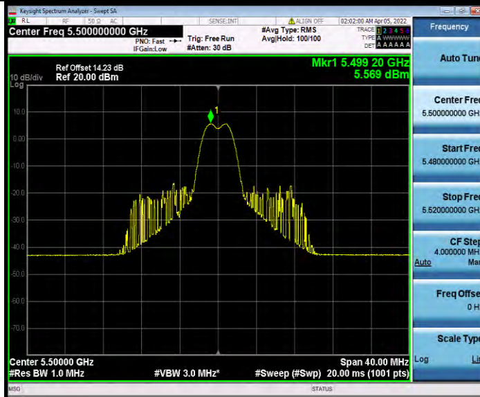
11AX20MIMO_Ant1_5500_26Tone_RU8
