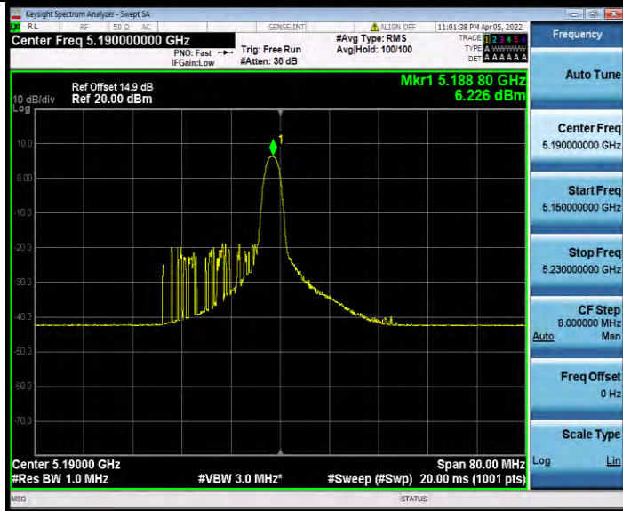
11AX40MIMO_Ant1_5190_26Tone_RU17
