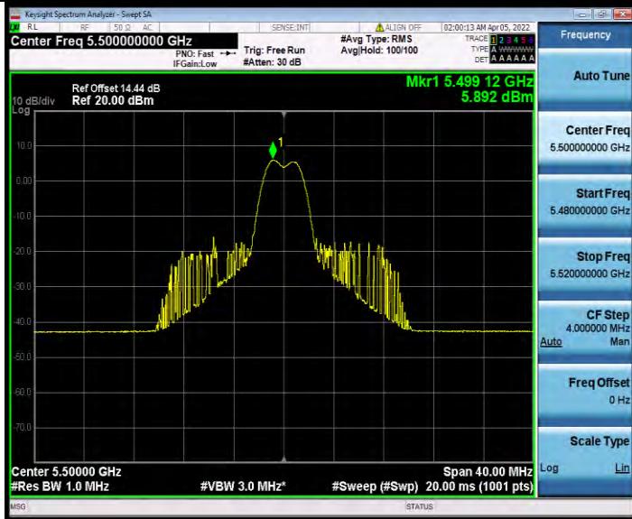
11AX20MIMO_Ant0_5500_26Tone_RU8
