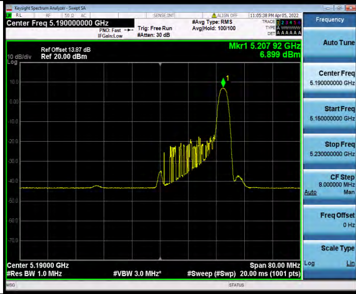
11AX40MIMO_Ant1_5190_484Tone_RU65
