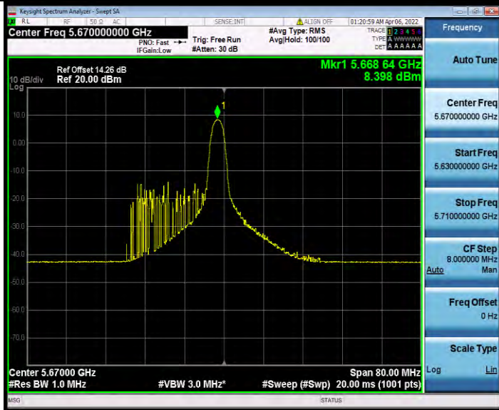
11AX40MIMO_Ant0_5670_26Tone_RU17
