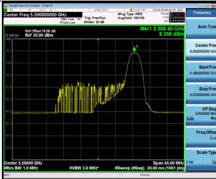
11AX20MIMO_Ant0_5500_242Tone_RU61
