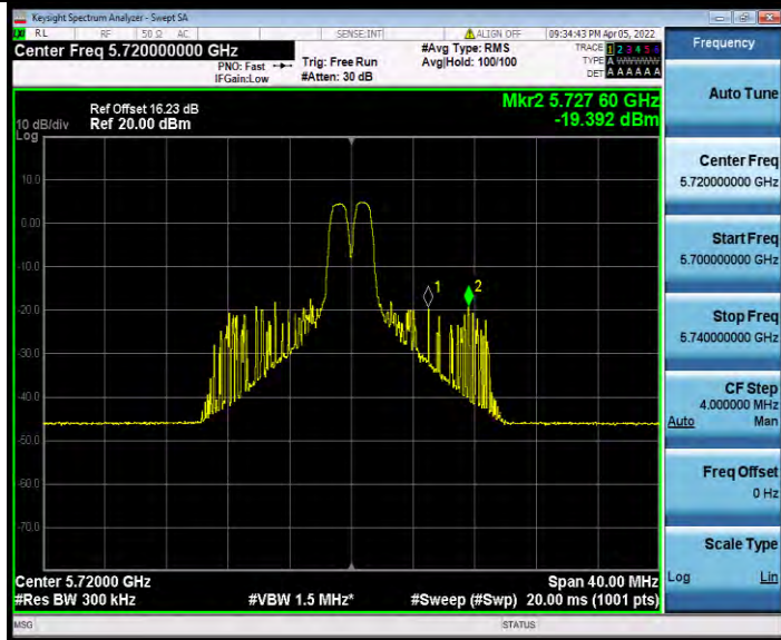
11AX20MIMO_Ant1_5720_UNII-3_26Tone_RU8
