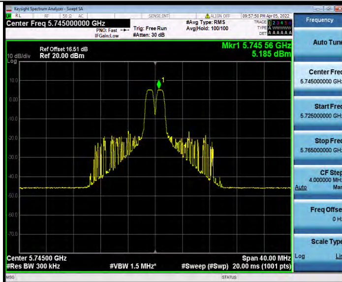
11AX20MIMO_Ant1_5745_26Tone_RU8
