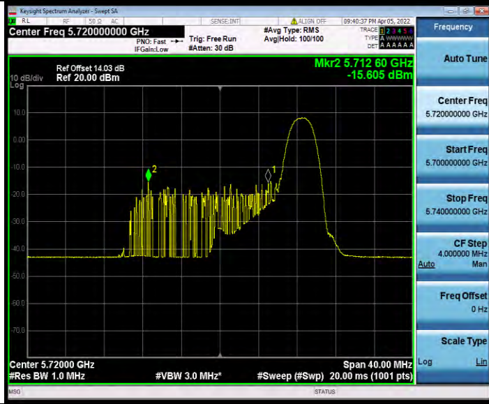
11AX20MIMO_Ant1_5720_UNII-2C_242Tone_RU61
