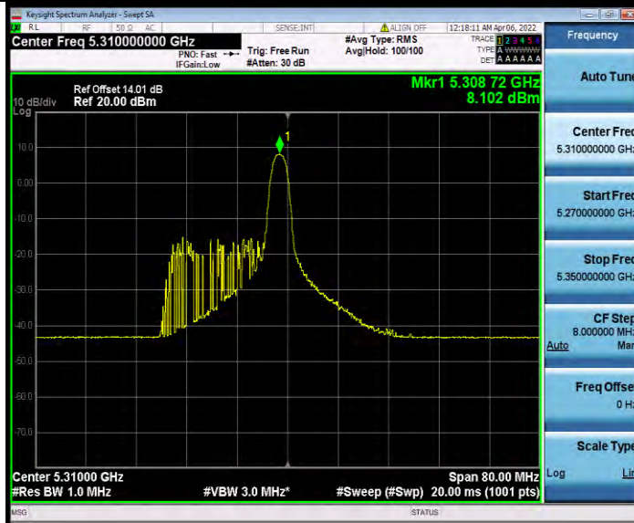
11AX40MIMO_Ant1_5310_26Tone_RU17
