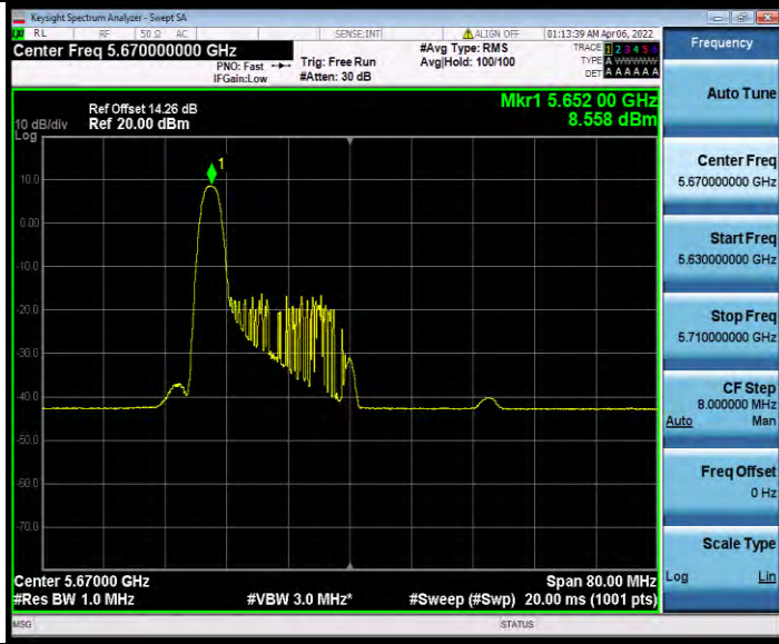
11AX40MIMO_Ant0_5670_26Tone_RU8
