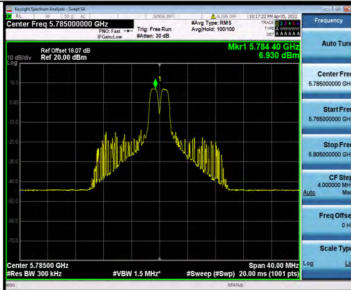
11AX20MIMO_Ant1_5785_26Tone_RU8
