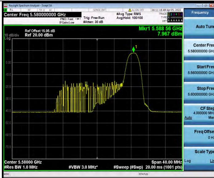
11AX20MIMO_Ant0_5580_242Tone_RU61
