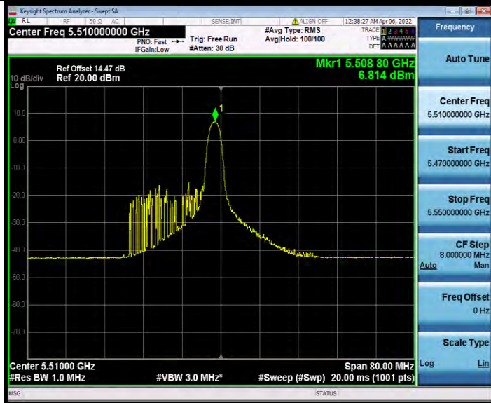
11AX40MIMO_Ant0_5510_26Tone_RU17
