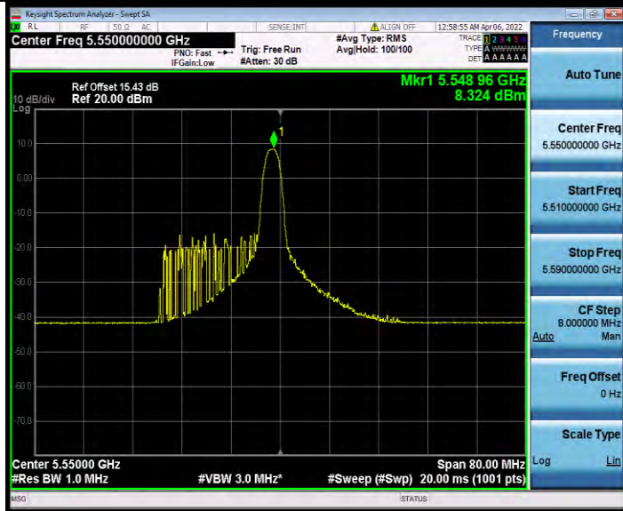
11AX40MIMO_Ant0_5550_26Tone_RU17
