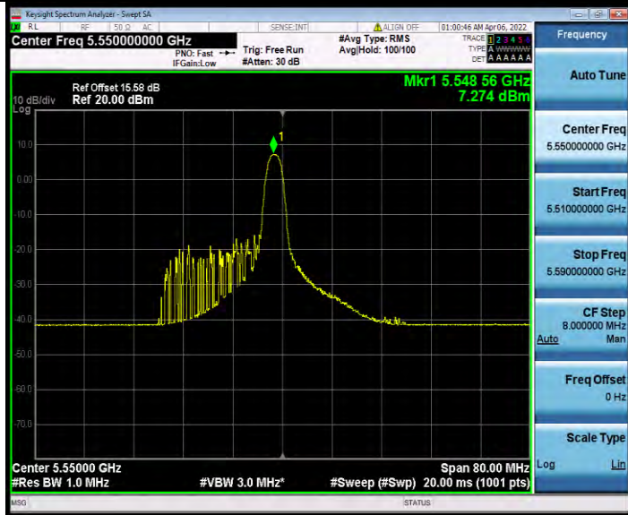
11AX40MIMO_Ant1_5550_26Tone_RU17
