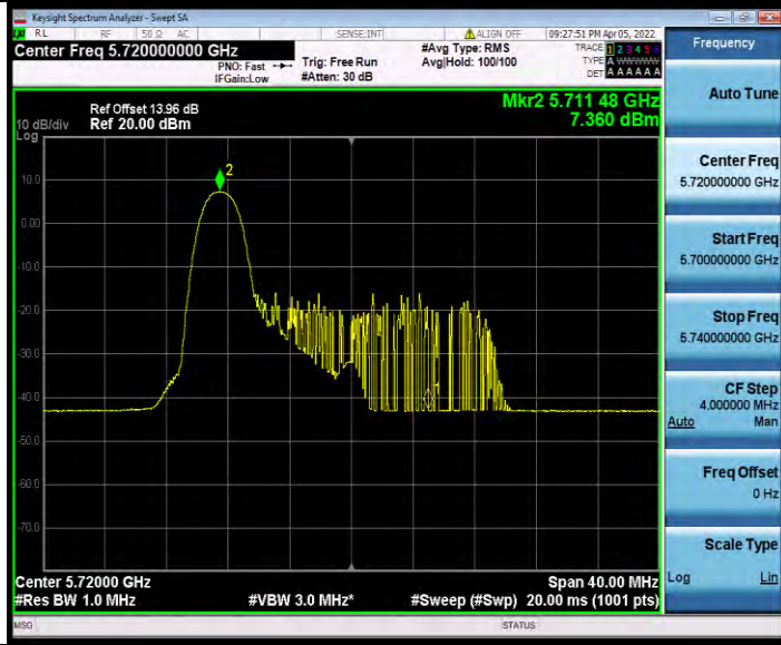
11AX20MIMO_Ant1_5720_UNII-2C_26Tone_RU4
