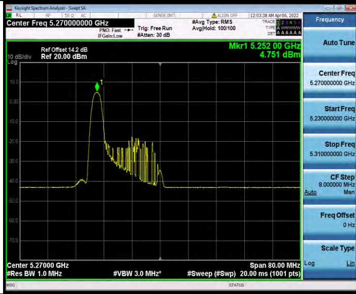
11AX40MIMO_Ant0_5270_26Tone_RU8
