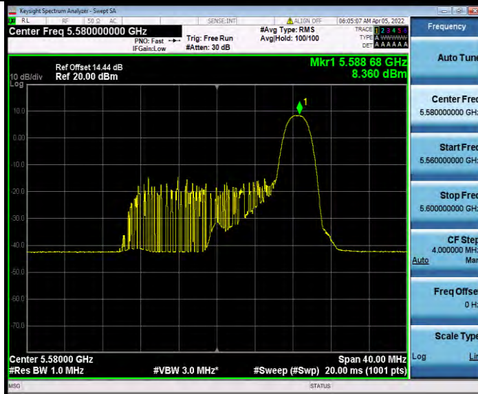
11AX20MIMO_Ant0_5580_26Tone_RU8
