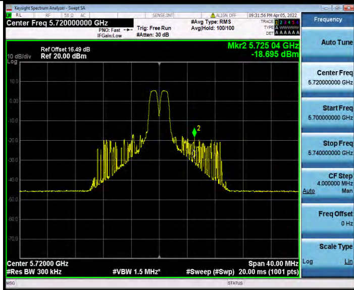
11AX20MIMO_Ant0_5720_UNII-3_26Tone_RU8
