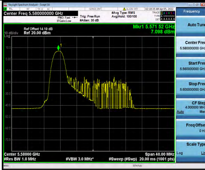
11AX20MIMO_Ant1_5580_26Tone_RU4
