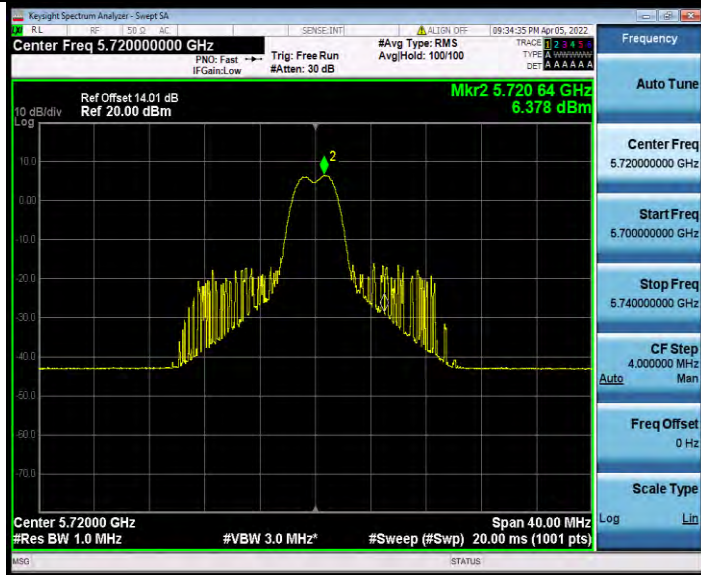
11AX20MIMO_Ant1_5720_UNII-2C_26Tone_RU8
