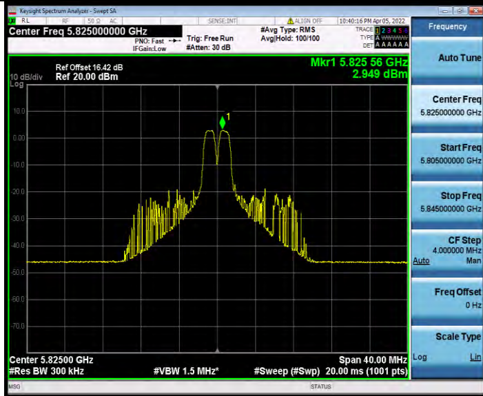
11AX20MIMO_Ant1_5825_26Tone_RU8
