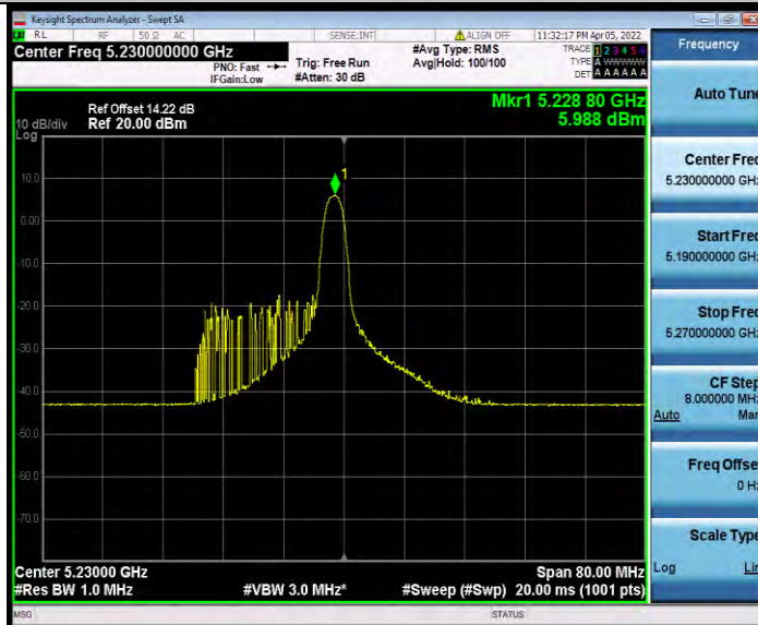
11AX40MIMO_Ant0_5230_26Tone_RU17
