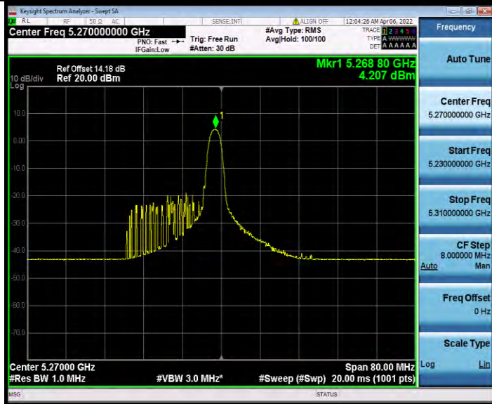
11AX40MIMO_Ant0_5270_26Tone_RU17
