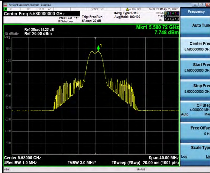
11AX20MIMO_Ant1_5580_26Tone_RU8
