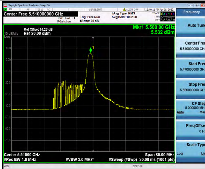
11AX40MIMO_Ant1_5510_26Tone_RU17
