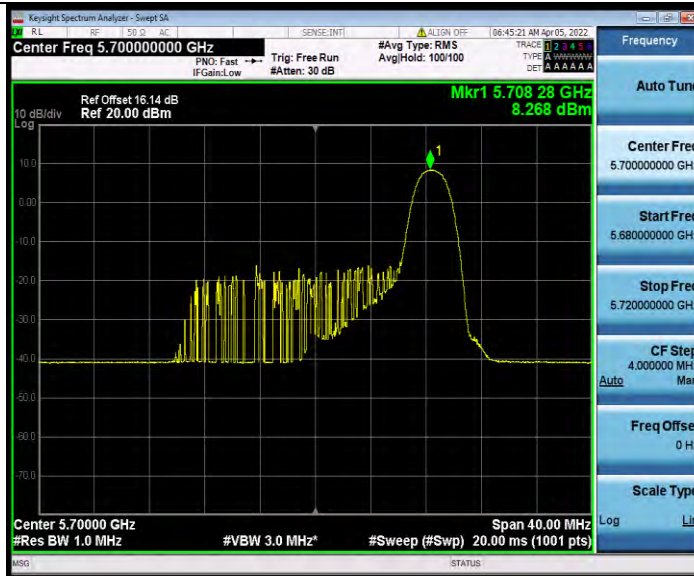
11AX20MIMO_Ant0_5700_242Tone_RU61
