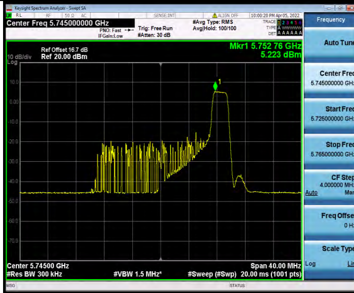
11AX20MIMO_Ant0_5745_242Tone_RU61
