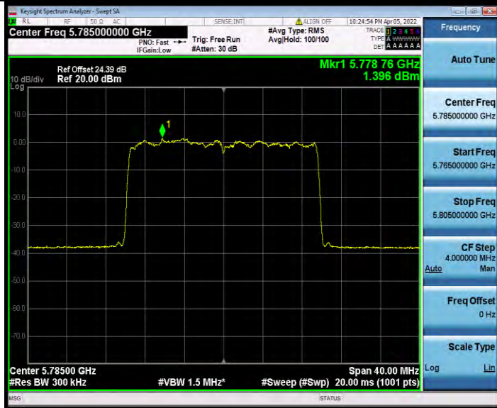
11AX20MIMO_Ant1_5785_26Tone_RU0
