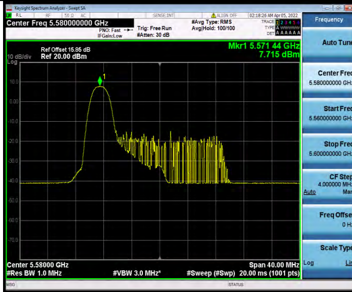
11AX20MIMO_Ant0_5580_26Tone_RU4
