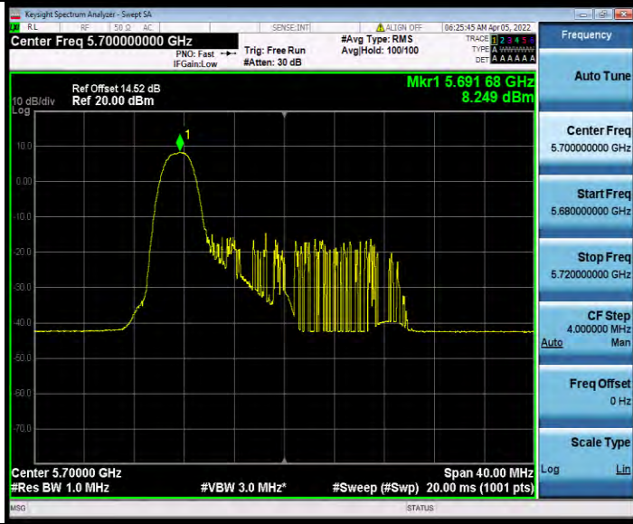
11AX20MIMO_Ant0_5700_26Tone_RU4
