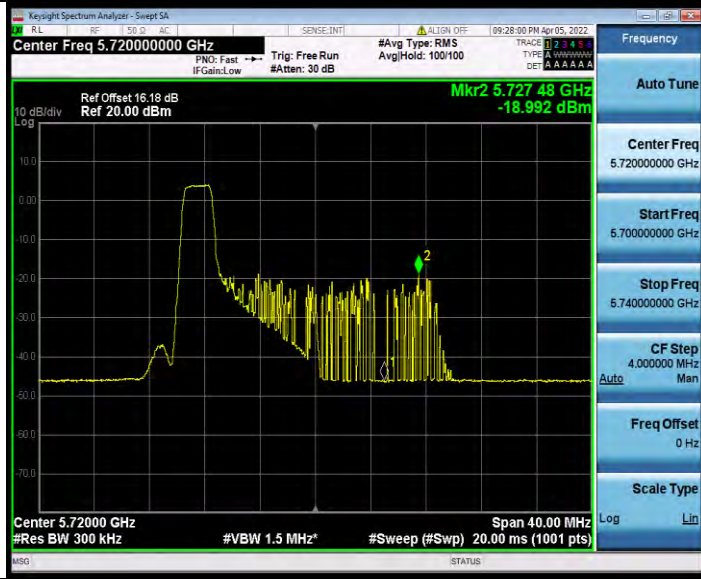
11AX20MIMO_Ant1_5720_UNII-3_26Tone_RU4
