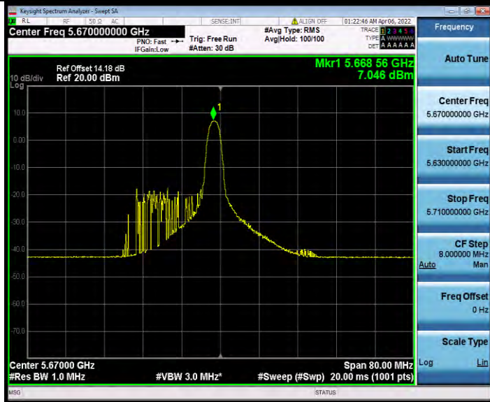
11AX40MIMO_Ant1_5670_26Tone_RU17
