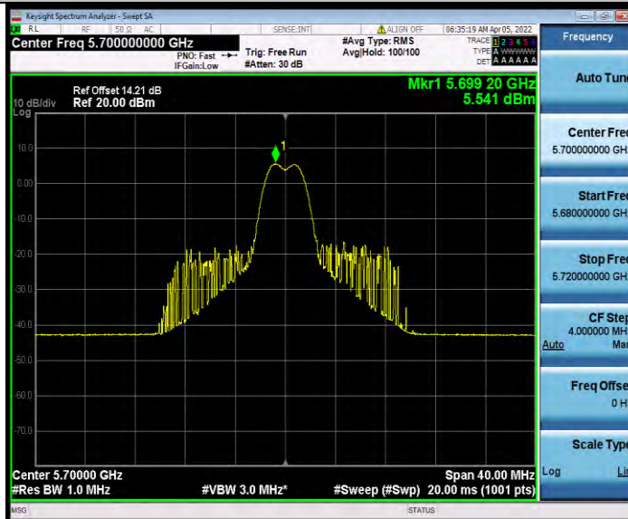
11AX20MIMO_Ant1_5700_26Tone_RU8
