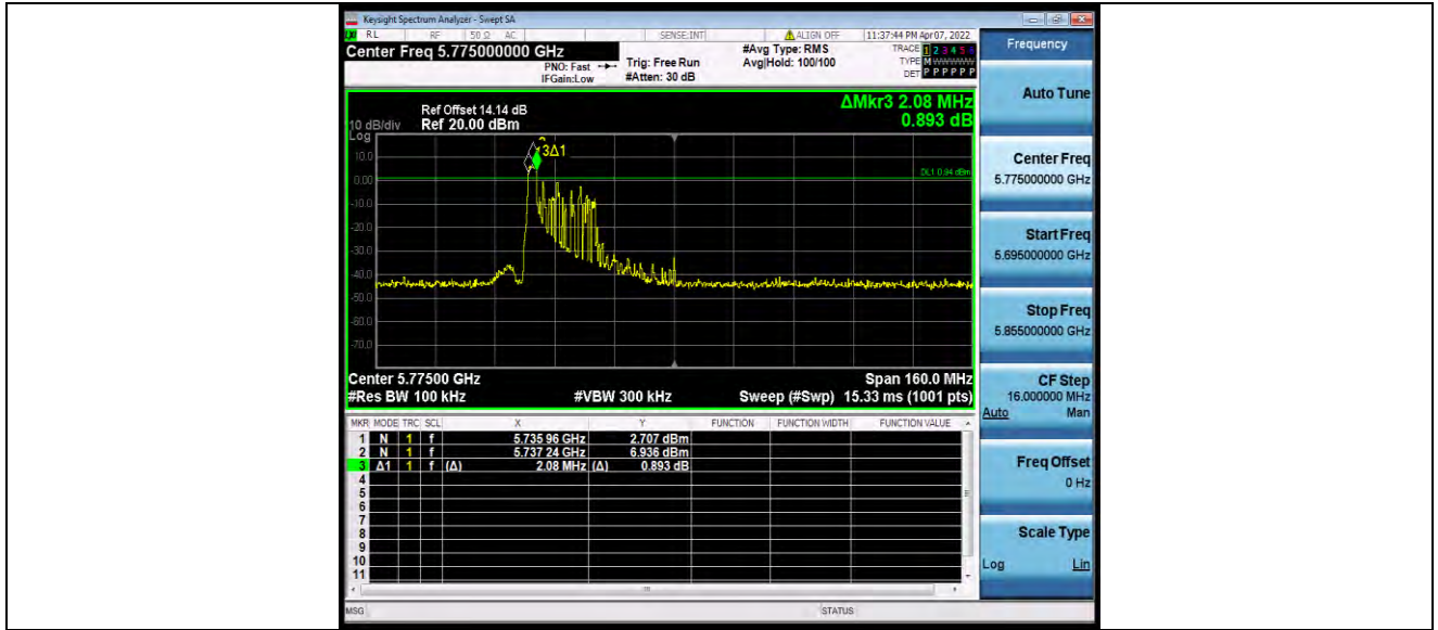
11AX80MIMO_Ant0_5775_26Tone_RU18
