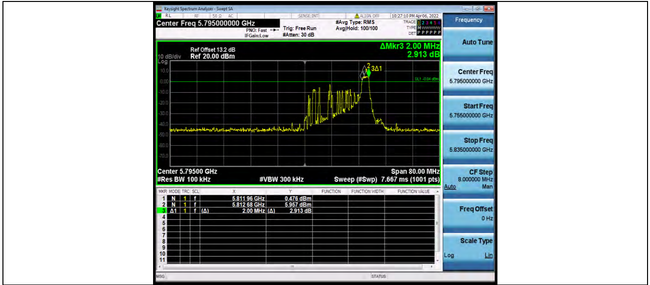
11AX40MIMO_Ant1_5795_484Tone_RU65
