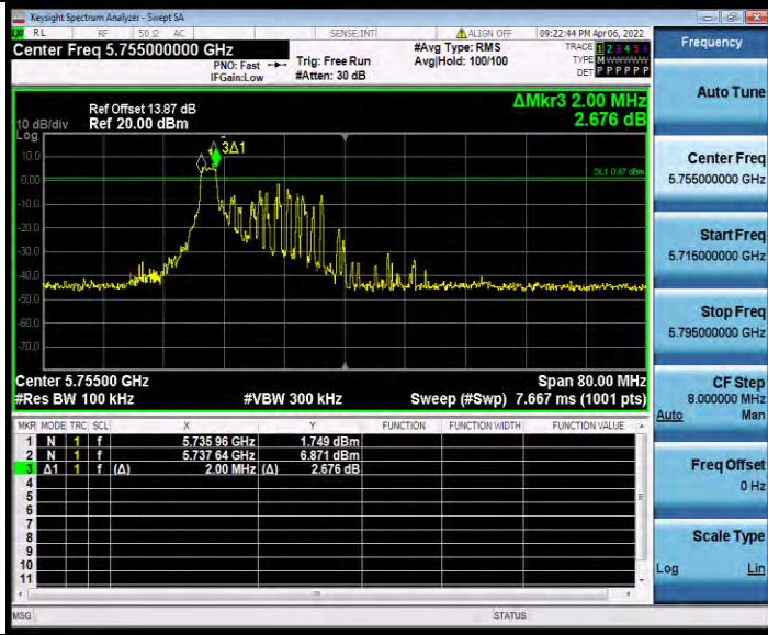
11AX40MIMO_Ant1_5755_26Tone_RU8
