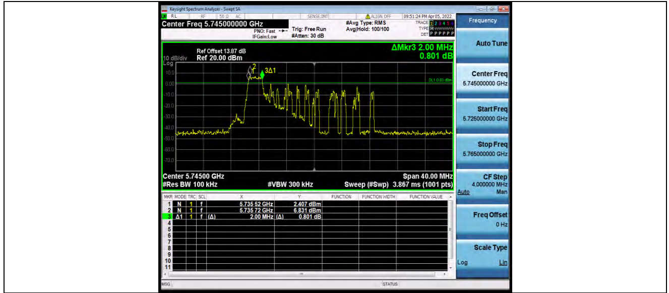
11AX20MIMO_Ant1_5745_26Tone_RU4
