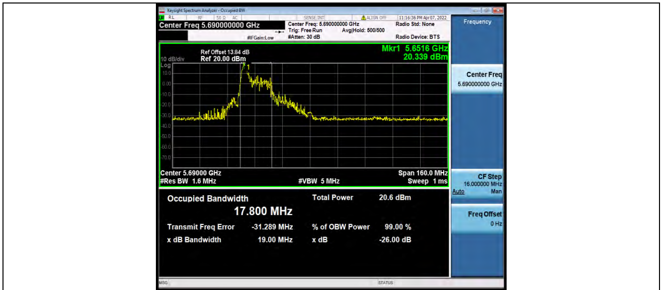
11AX80MIMO_Ant1_5690_26Tone_RU18
