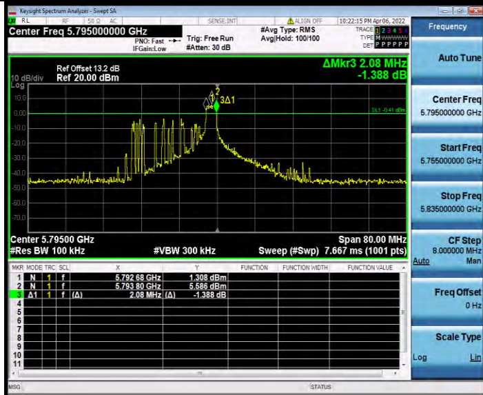
11AX40MIMO_Ant1_5795_26Tone_RU17
