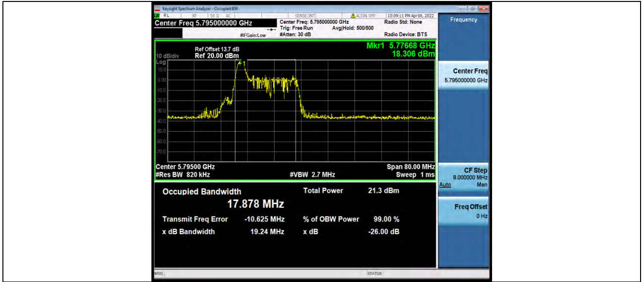
11AX40MIMO_Ant1_5795_26Tone_RU8
