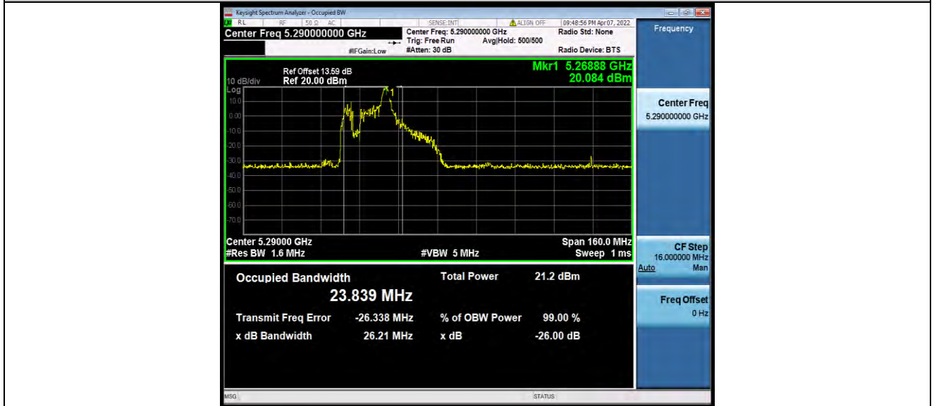
11AX80MIMO_Ant1_5290_26Tone_RU36
