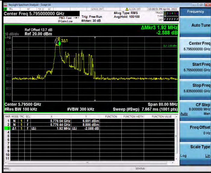
11AX40MIMO_Ant1_5795_26Tone_RU8
