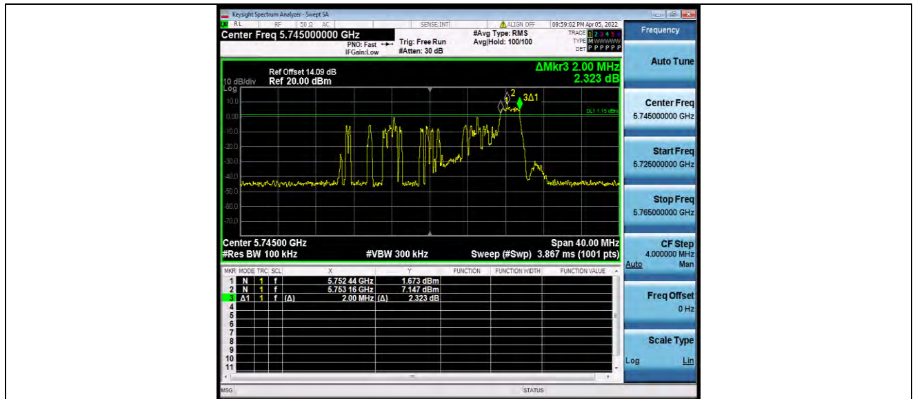
11AX20MIMO_Ant0_5745_242Tone_RU61
