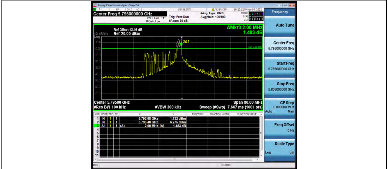
11AX40MIMO_Ant0_5795_26Tone_RU17
