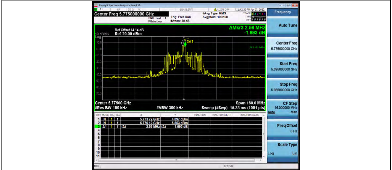
11AX80MIMO_Ant0_5775_26Tone_RU36
