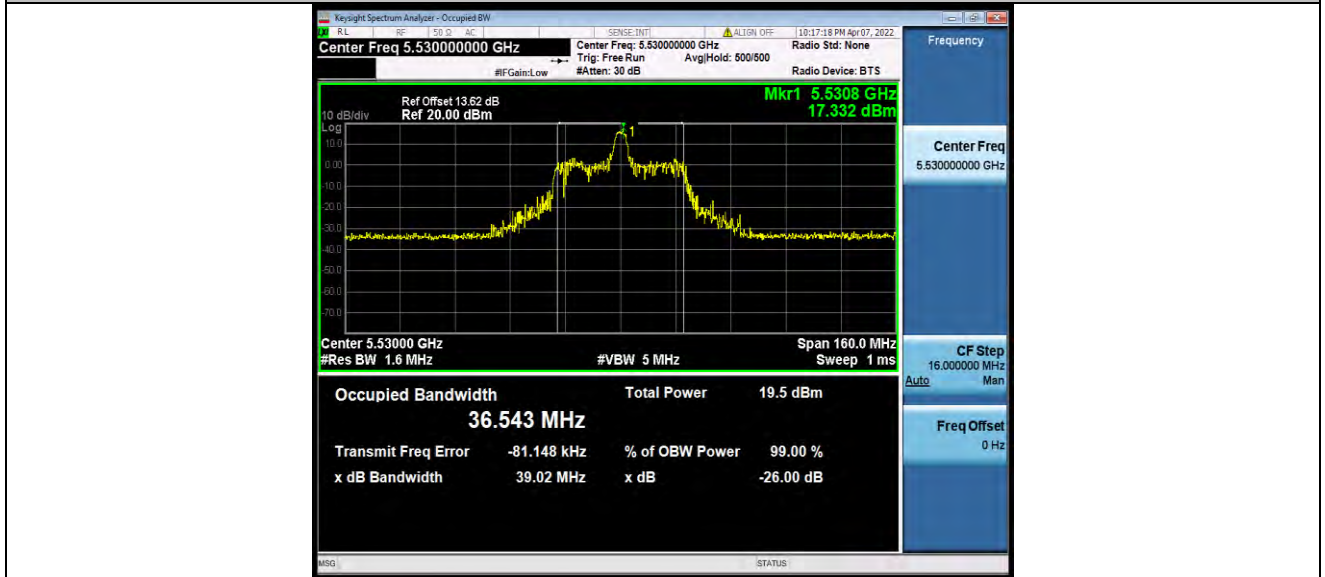
11AX80MIMO_Ant1_5530_26Tone_RU36
