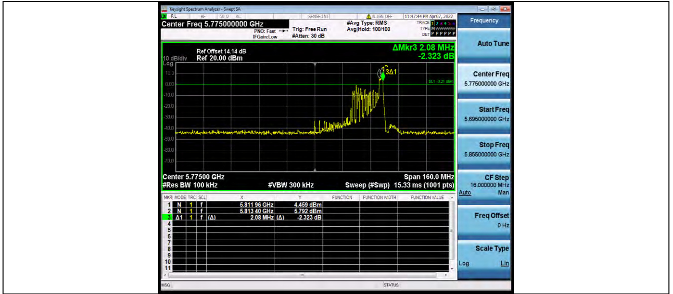
11AX80MIMO_Ant0_5775_996Tone_RU67
