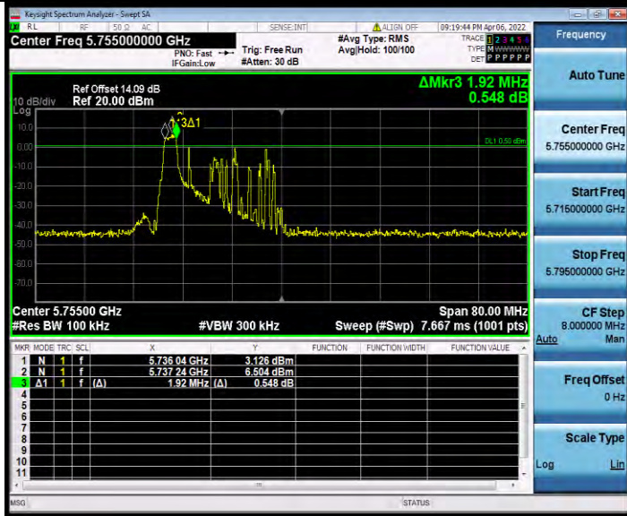
11AX40MIMO_Ant0_5755_26Tone_RU8
