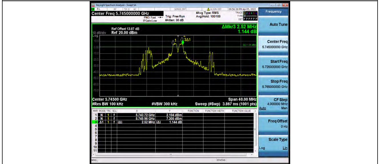
11AX20MIMO_Ant1_5745_26Tone_RU8
