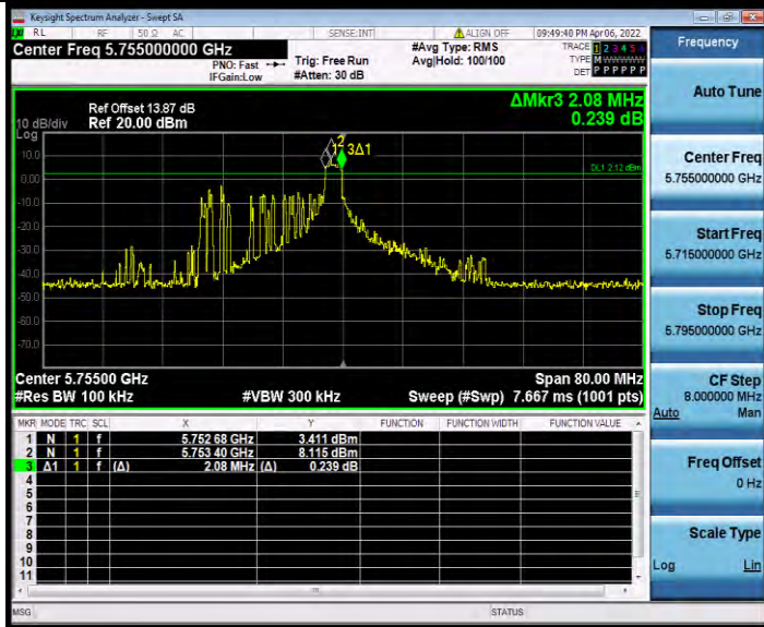
11AX40MIMO_Ant1_5755_26Tone_RU17
