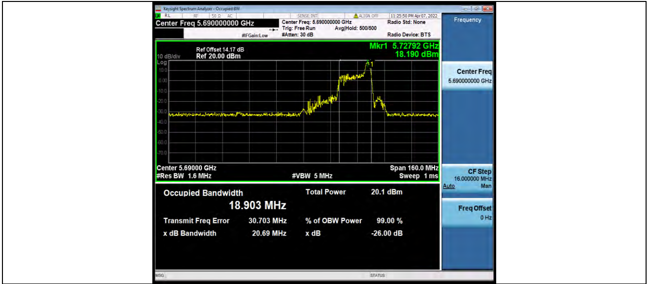
11AX80MIMO_Ant0_5690_996Tone_RU67
