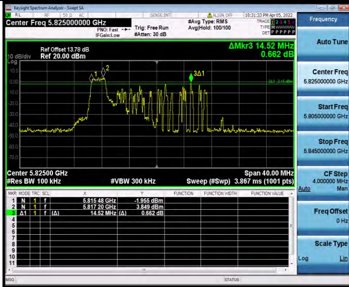
11AX20MIMO_Ant1_5825_26Tone_RU4
