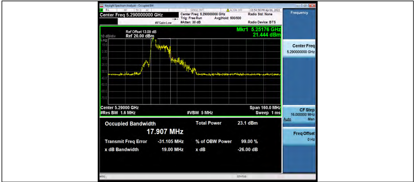
11AX80MIMO_Ant1_5290_26Tone_RU18
