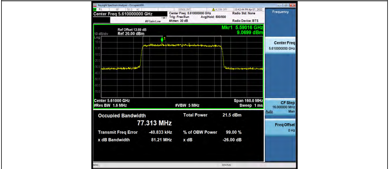
11AX80MIMO_Ant1_5610_26Tone_RU0
