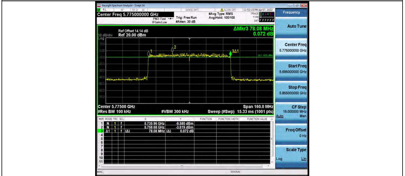
11AX80MIMO_Ant1_5775_26Tone_RU0
