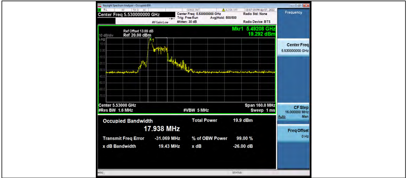
11AX80MIMO_Ant0_5530_26Tone_RU18
