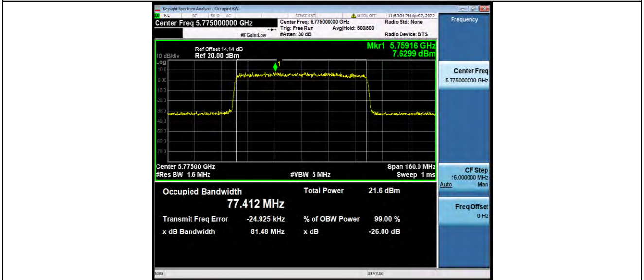
11AX80MIMO_Ant1_5775_26Tone_RU0
