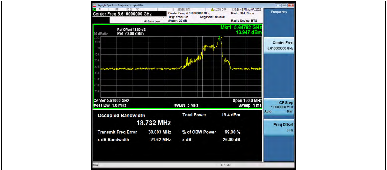
11AX80MIMO_Ant0_5610_996Tone_RU67
