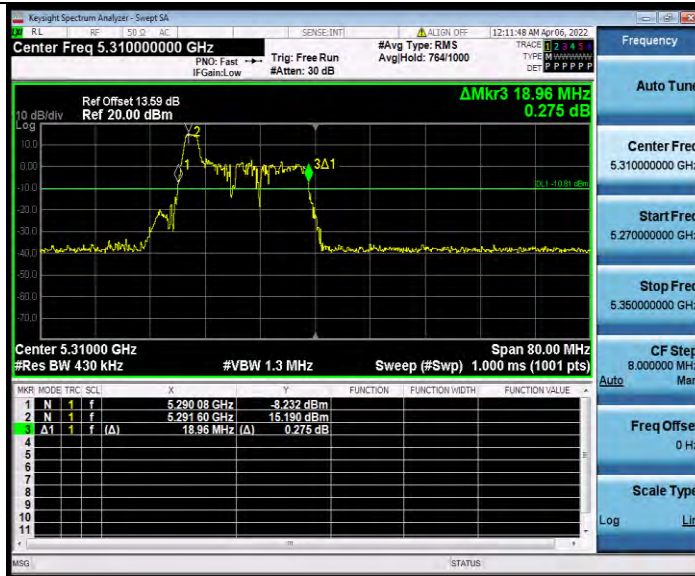
11AX40MIMO_Ant1_5310_26Tone_RU8
