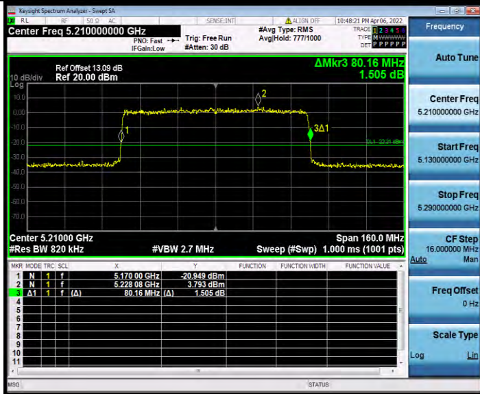
11AX80MIMO_Ant1_5210_26Tone_RU0
