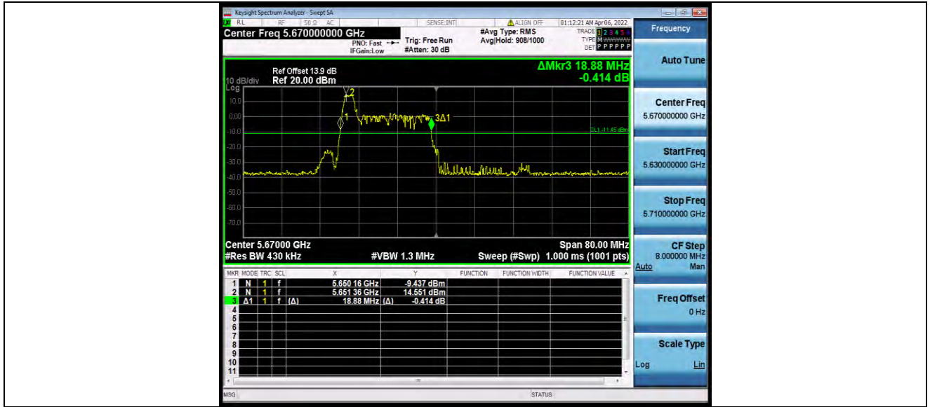
11AX40MIMO_Ant0_5670_26Tone_RU8
