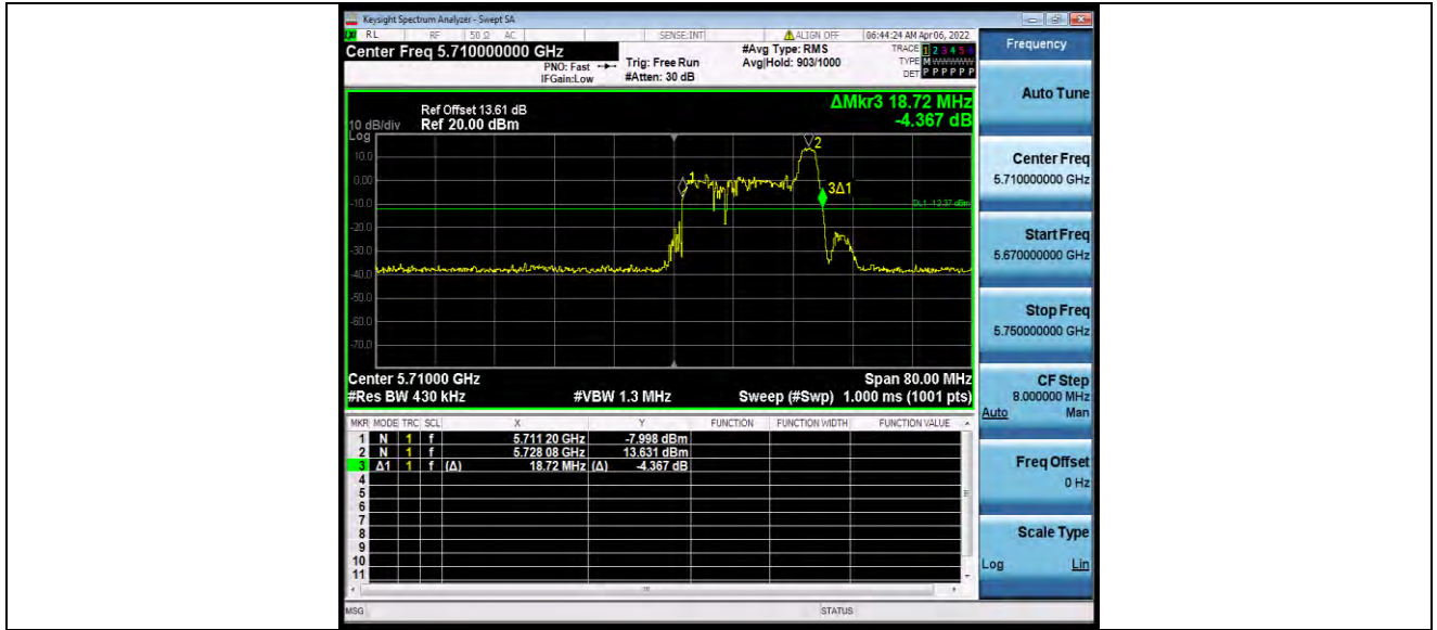
11AX40MIMO_Ant1_5710_484Tone_RU65
