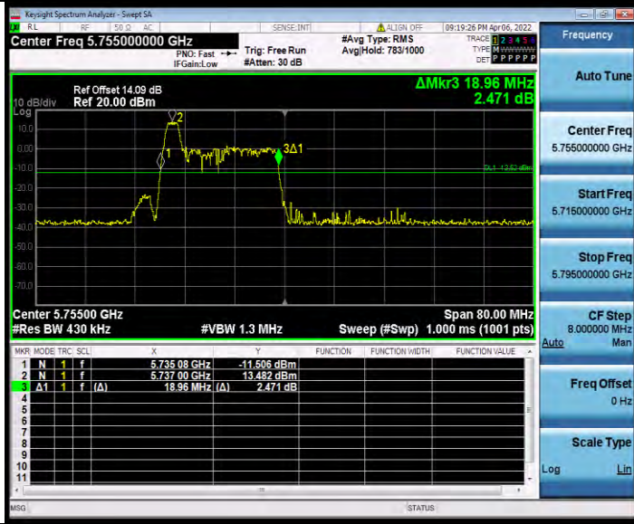
11AX40MIMO_Ant0_5755_26Tone_RU8
