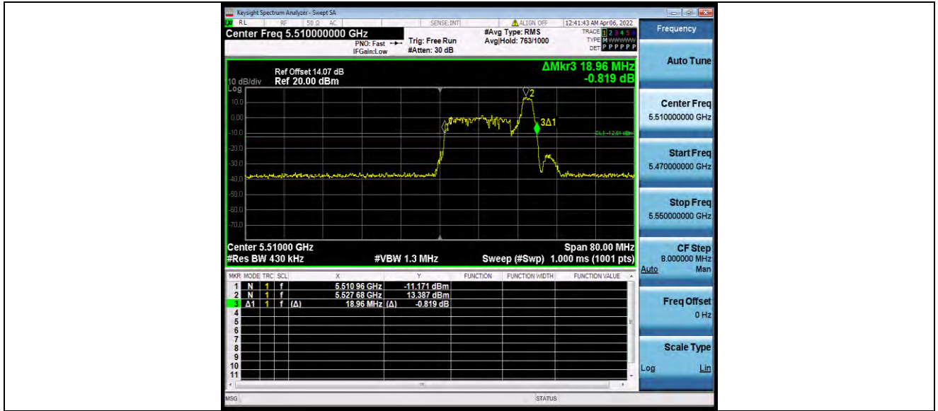
11AX40MIMO_Ant0_5510_484Tone_RU65
