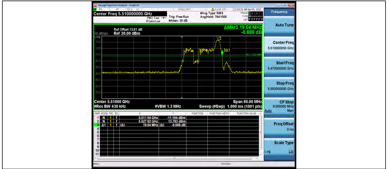
11AX40MIMO_Ant1_5510_484Tone_RU65
