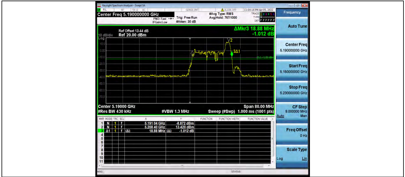
11AX40MIMO_Ant1_5190_484Tone_RU65
