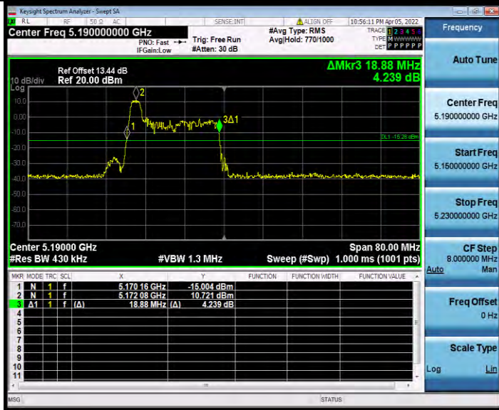
11AX40MIMO_Ant1_5190_26Tone_RU8
