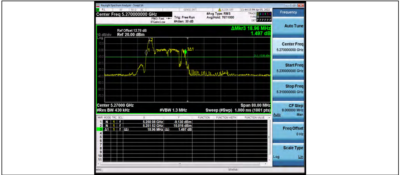
11AX40MIMO_Ant0_5270_26Tone_RU8
