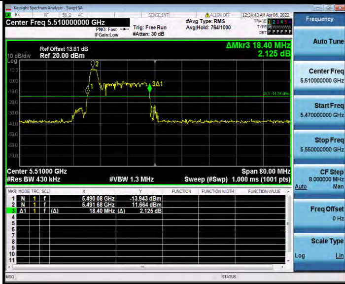
11AX40MIMO_Ant1_5510_26Tone_RU8
