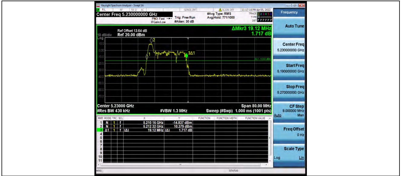
11AX40MIMO_Ant1_5230_26Tone_RU8
