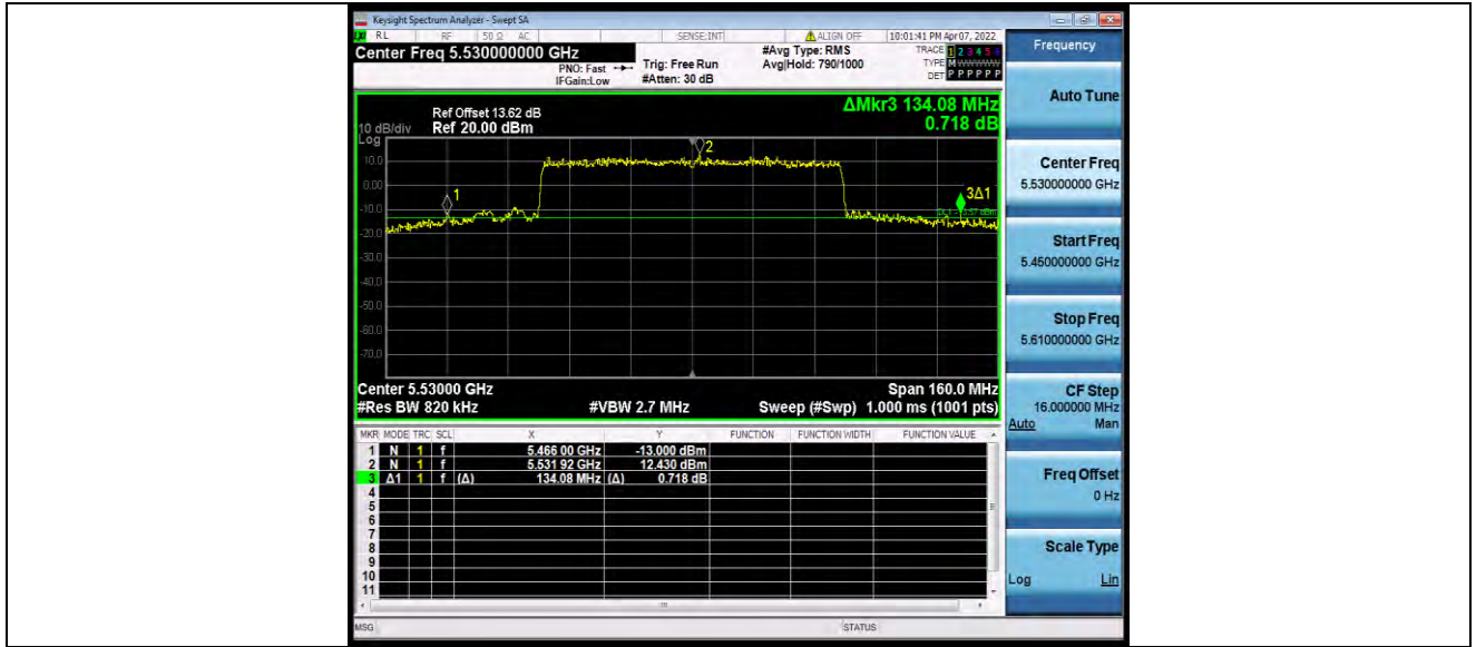
11AX80MIMO_Ant1_5530_26Tone_RU18
