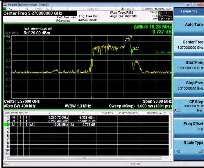
11AX40MIMO_Ant1_5270_484Tone_RU65
