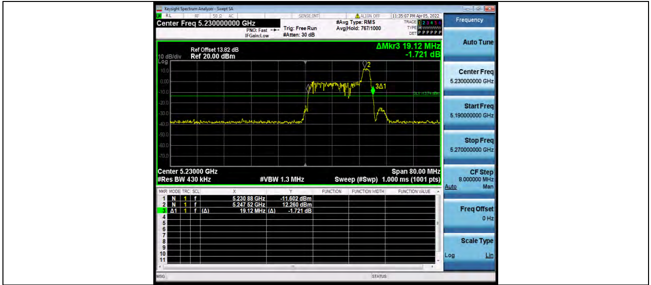
11AX40MIMO_Ant0_5230_484Tone_RU65
