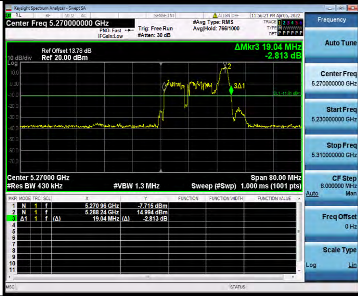
11AX40MIMO_Ant0_5270_484Tone_RU65
