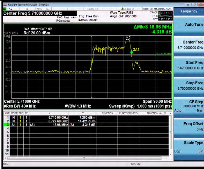
11AX40MIMO_Ant0_5710_484Tone_RU65
