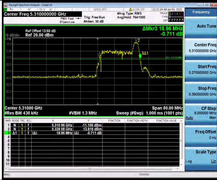
11AX40MIMO_Ant1_5310_484Tone_RU65
