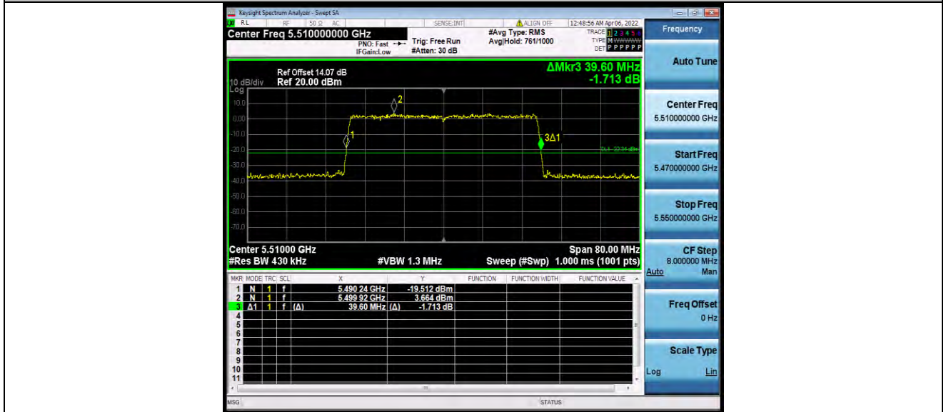
11AX40MIMO_Ant1_5510_26Tone_RU0
