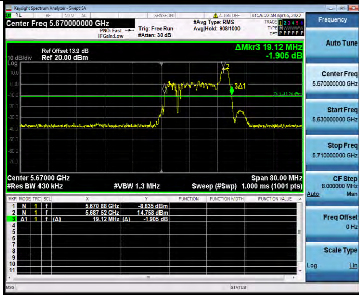
11AX40MIMO_Ant0_5670_484Tone_RU65
