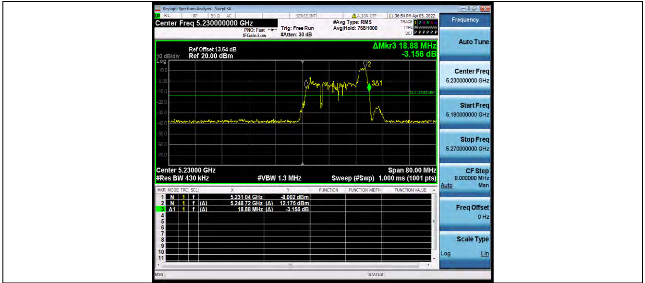
11AX40MIMO_Ant1_5230_484Tone_RU65
