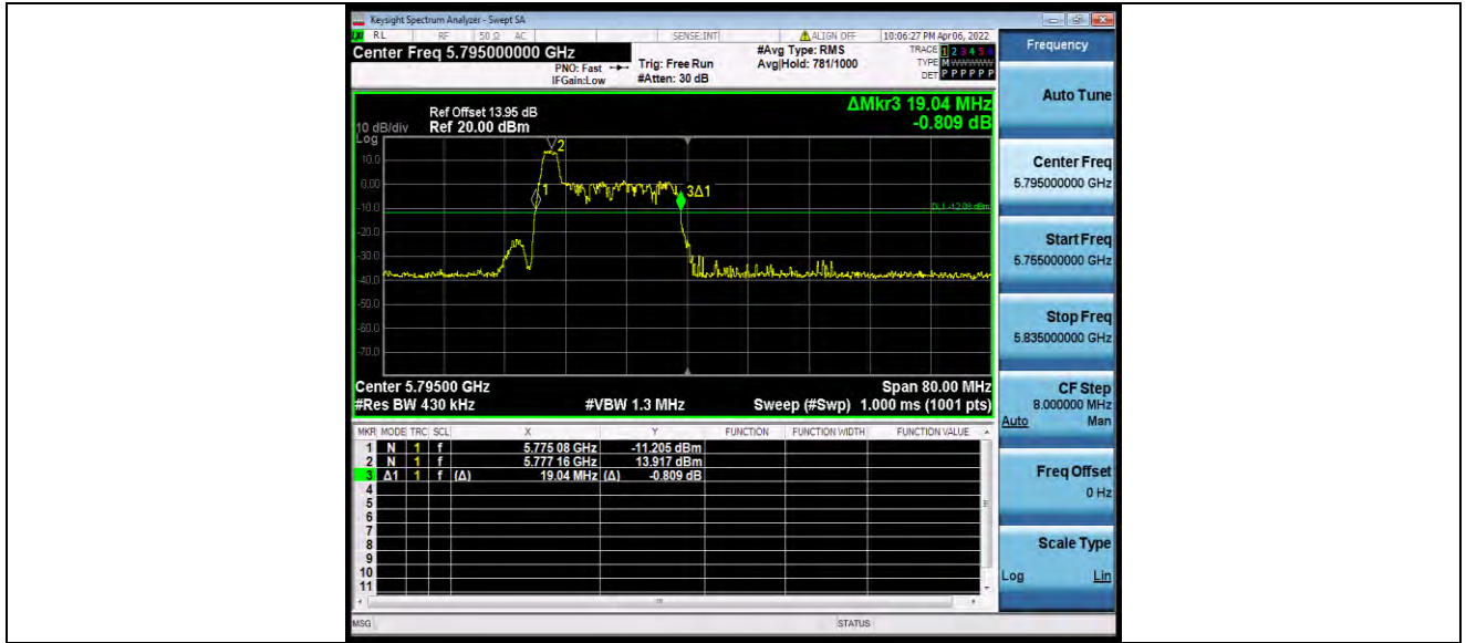
11AX40MIMO_Ant0_5795_26Tone_RU8
