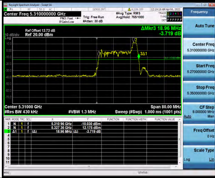
11AX40MIMO_Ant0_5310_484Tone_RU65
