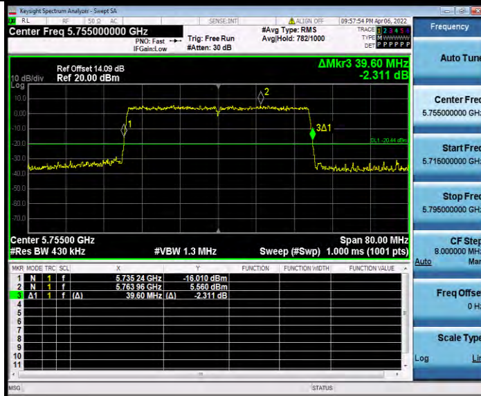
11AX40MIMO_Ant1_5755_26Tone_RU0
