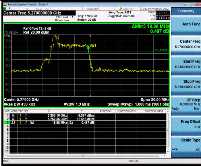
11AX40MIMO_Ant1_5270_26Tone_RU8
