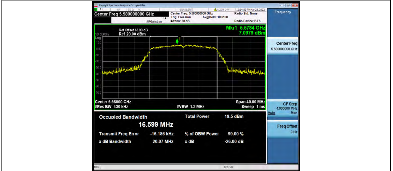
11A-CDD_Ant1_5580
