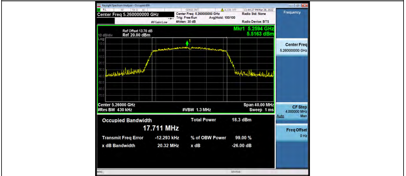
11N20MIMO_Ant1_5260
