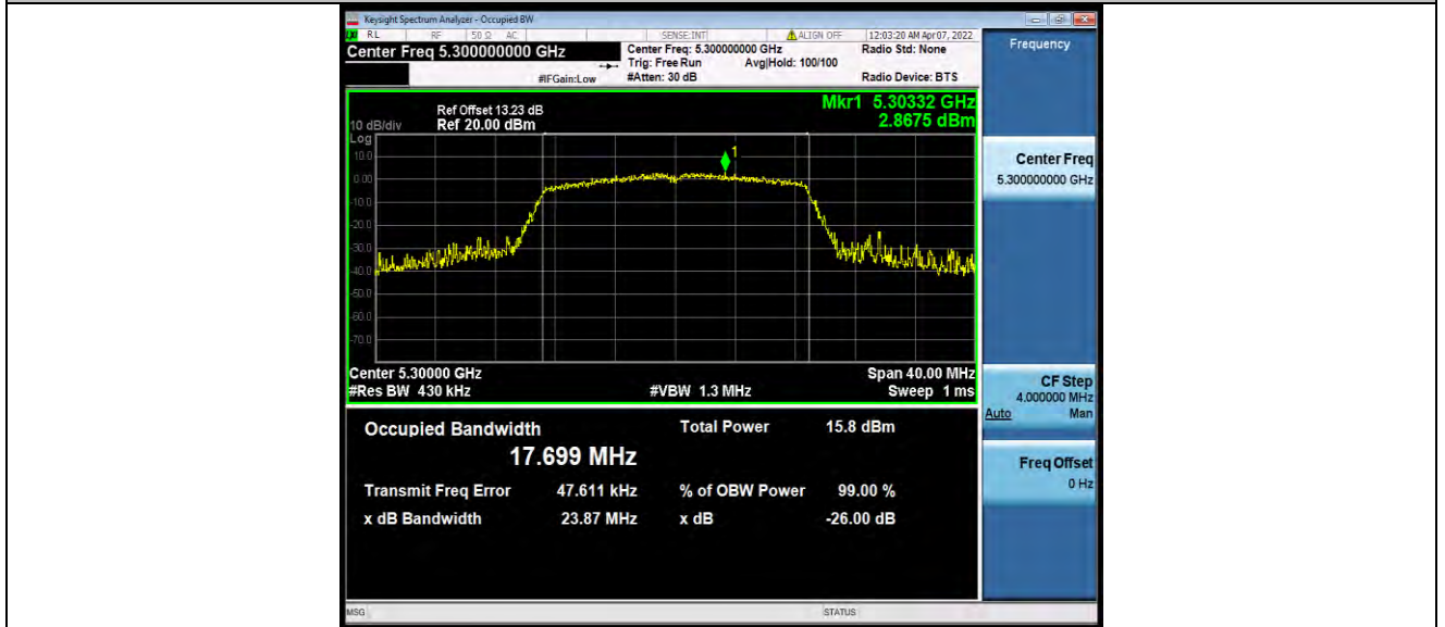
11N20MIMO_Ant1_5300
