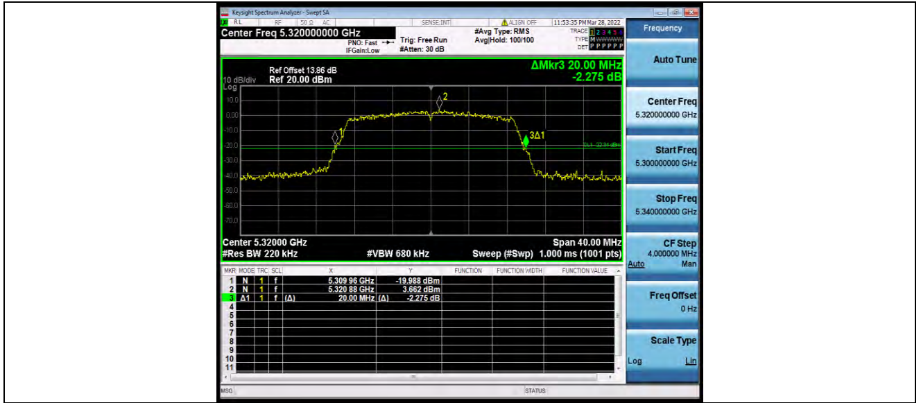
11N20MIMO_Ant1_5320
