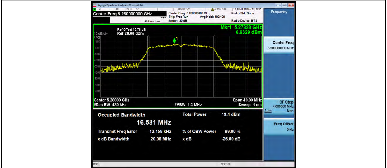
11A-CDD_Ant1_5280
