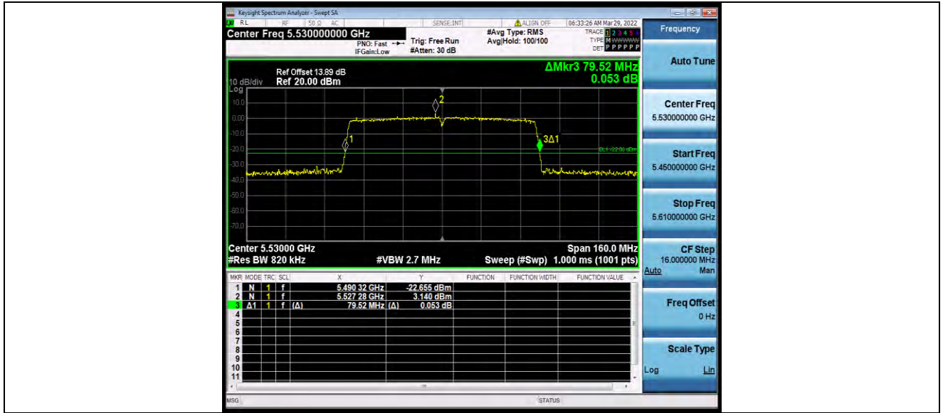
11AC80MIMO_Ant1_5530
