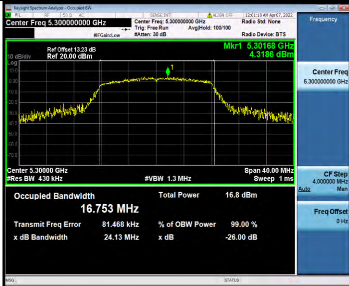
11A-CDD_Ant1_5300
