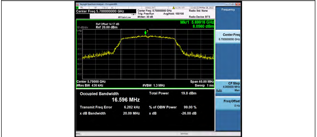
11A-CDD_Ant1_5700
