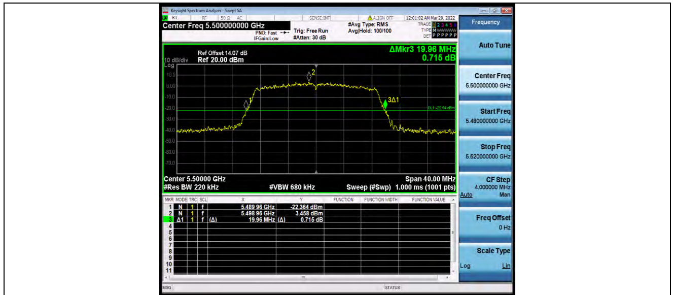
11N20MIMO_Ant1_5500
