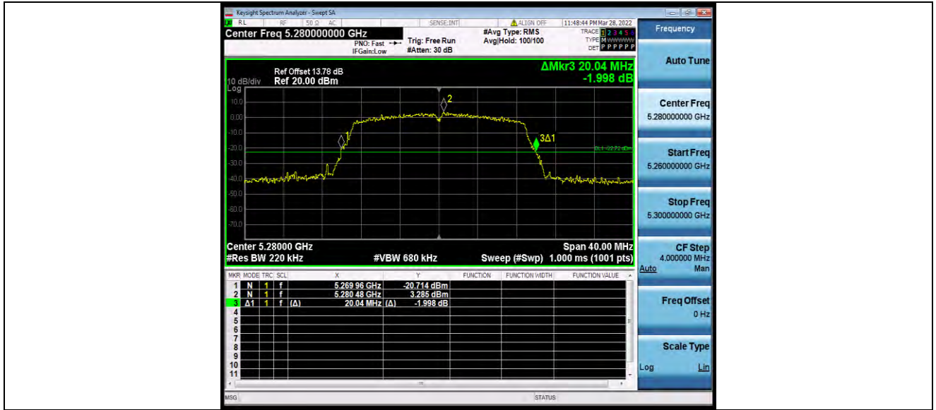
11N20MIMO_Ant1_5280
