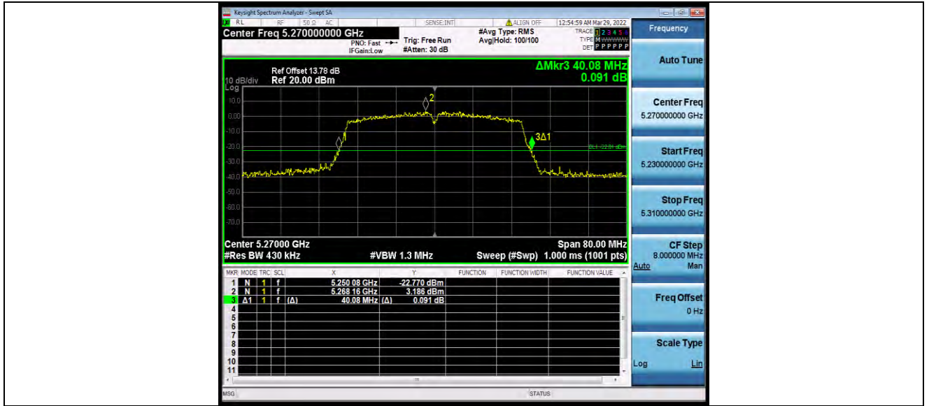
11N40MIMO_Ant1_5270
