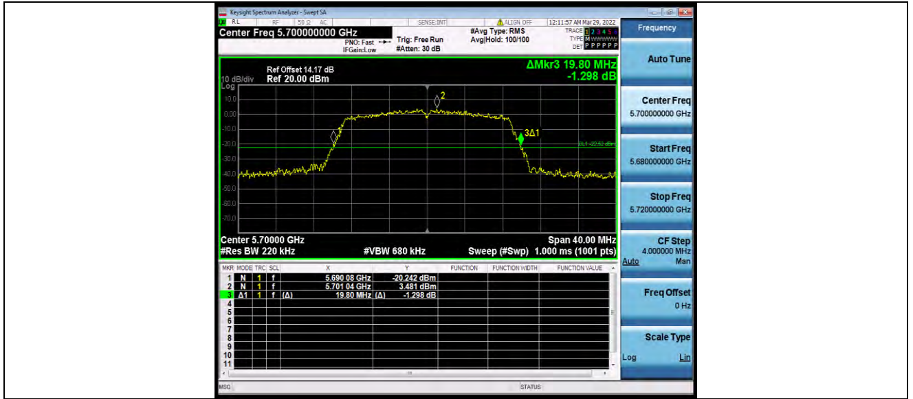
11N20MIMO_Ant1_5700
