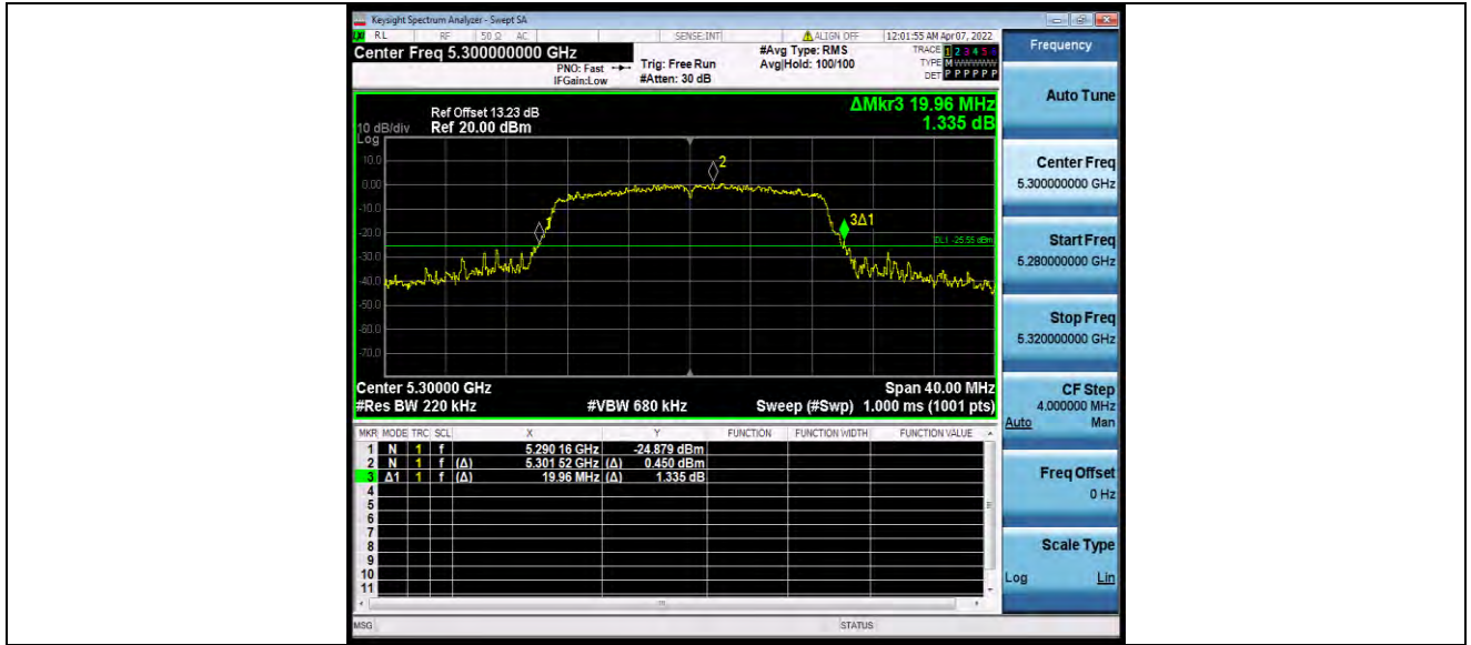
11N20MIMO_Ant1_5300
