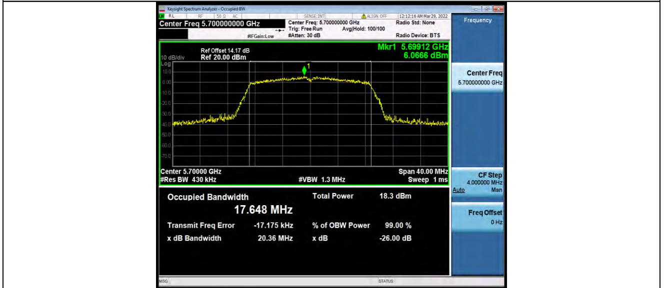
11N20MIMO_Ant1_5700
