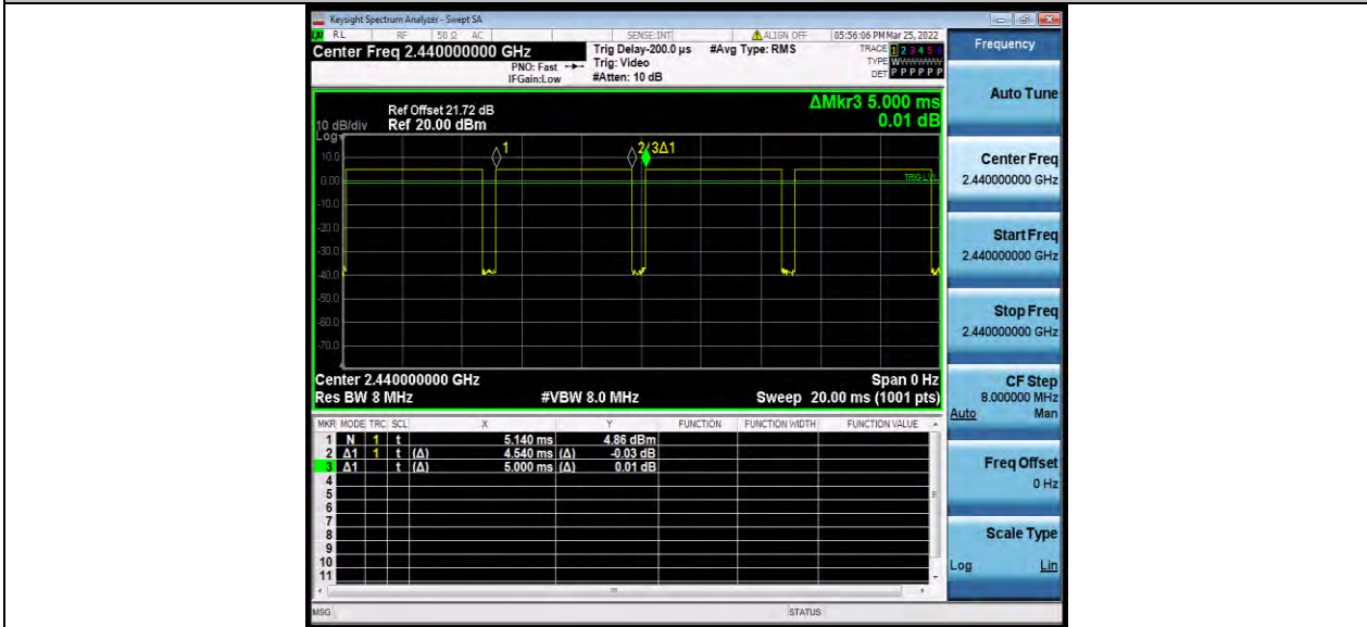
BLE_500K_ant1_2440
