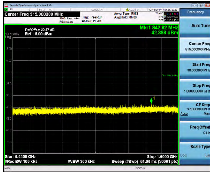
11N40MIMO_Ant0_2422_1000~26500
