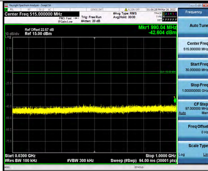
11N20MIMO_Ant0_2412_1000~26500
