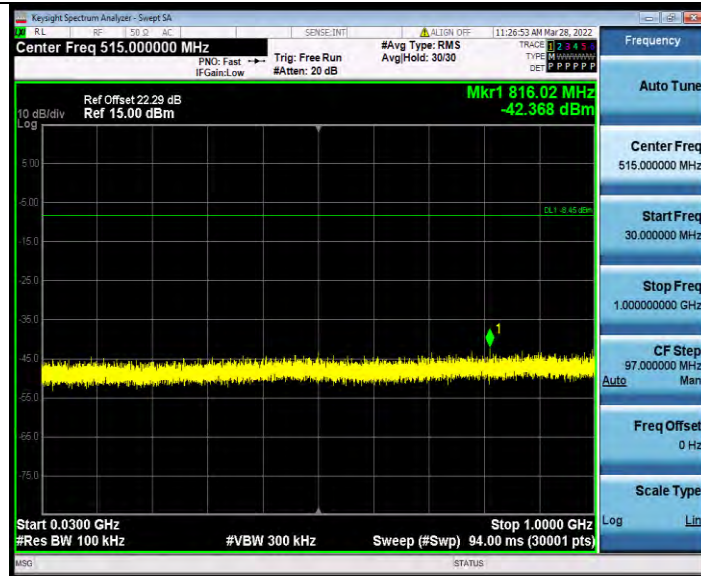
11B-CDD_Ant1_2462_1000~26500
