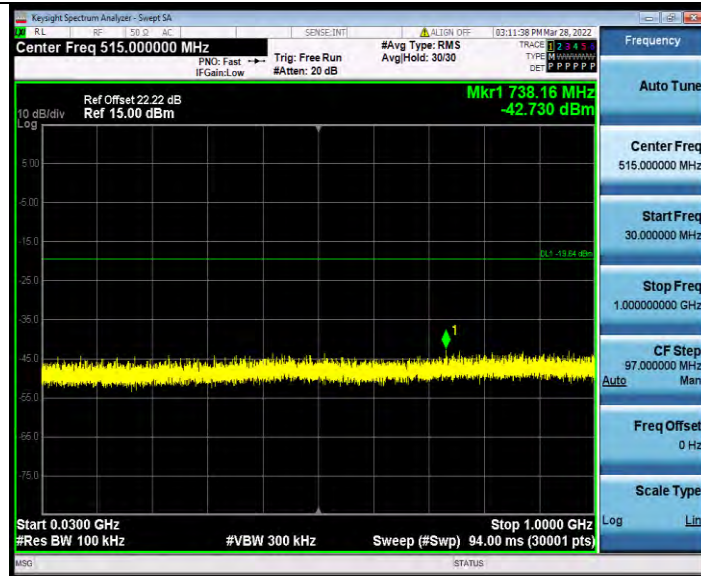
11N40MIMO_Ant0_2437_1000~26500
