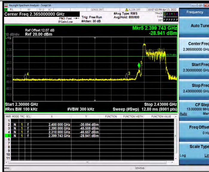
11AX40MIMO_Ant0_Low_2422_26Tone_RU8
