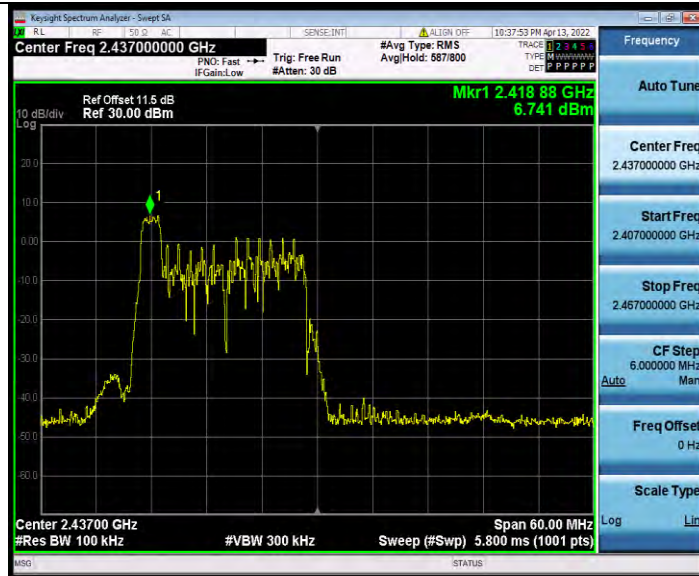
11AX40MIMO_Ant1_2437_26Tone_RU8
