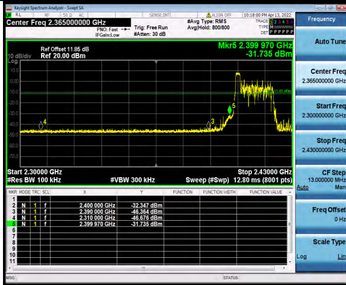
11AX40MIMO_Ant1_Low_2422_26Tone_RU8
