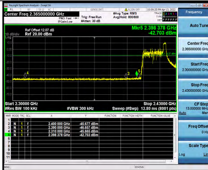
11AX40MIMO_Ant0_Low_2422_26Tone_RU17
