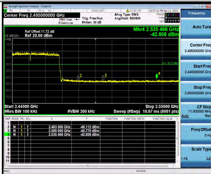
11AX40MIMO_Ant1_High_2452_26Tone_RU0
