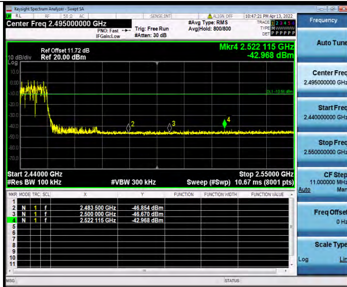
11AX40MIMO_Ant0_High_2452_26Tone_RU8
