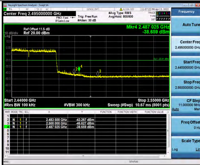
11AX40MIMO_Ant1_High_2452_484Tone_RU65
