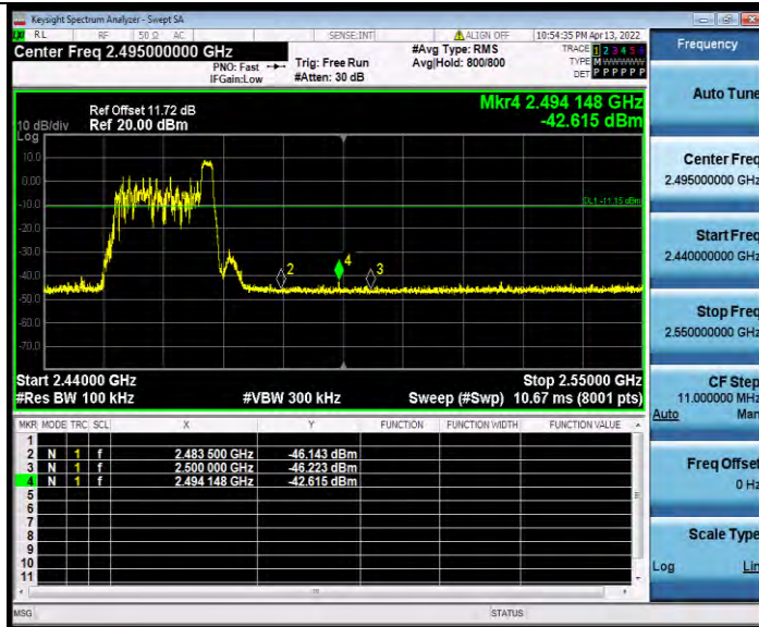
11AX40MIMO_Ant0_High_2452_484Tone_RU65
