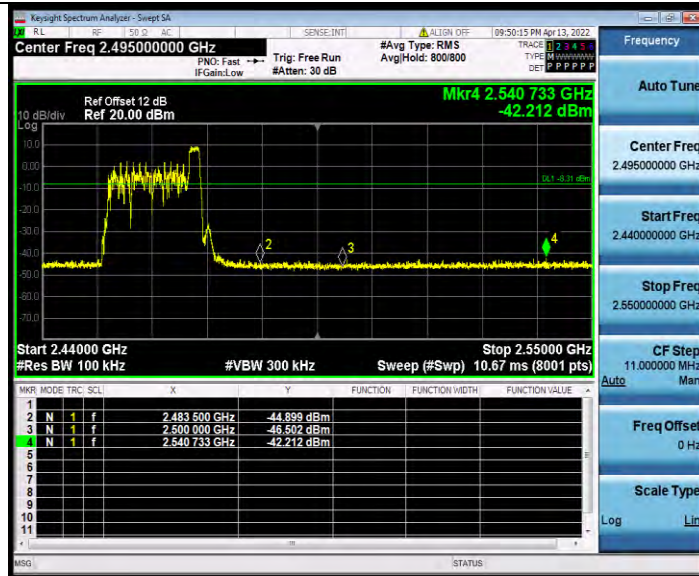
11AX20MIMO_Ant0_High_2462_242Tone_RU61
