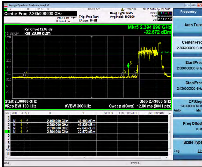
11AX20MIMO_Ant0_Low_2412_242Tone_RU61
