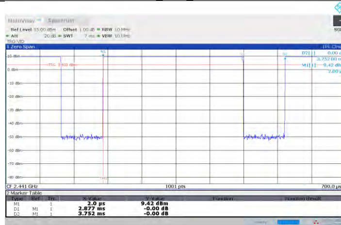
DH5_Ant1_2441
