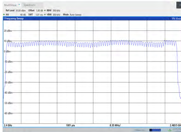
2DH5_Ant1_Hop
