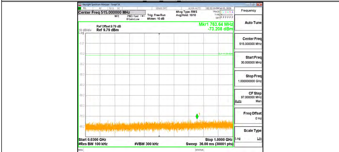
LE Ant2 2440 30~1000
