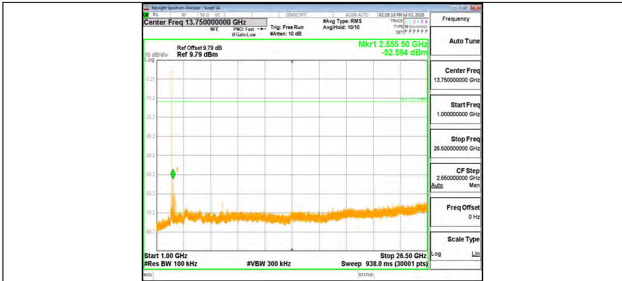
LE Ant2 2440 0~Reference
