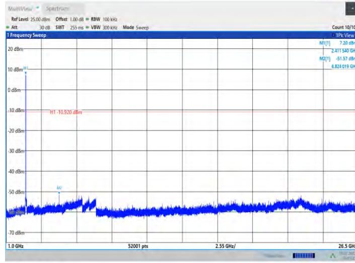
11B_Ant7_2412_1000~26500
