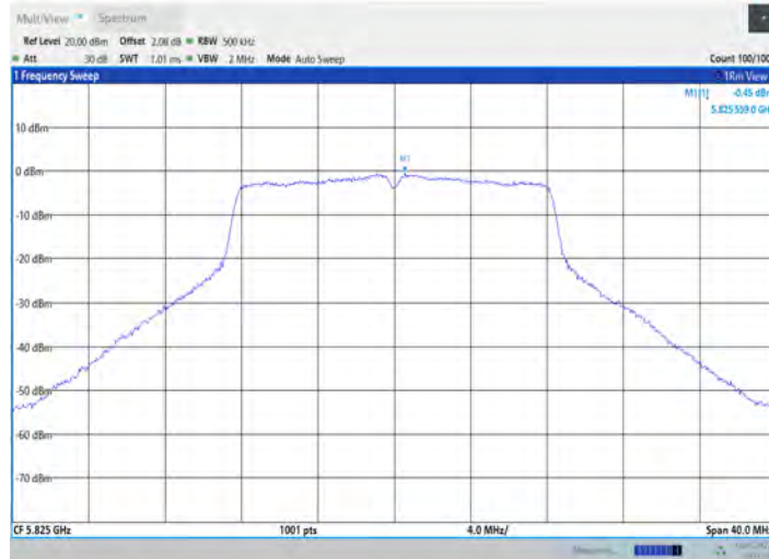
11A_Ant7_5825
