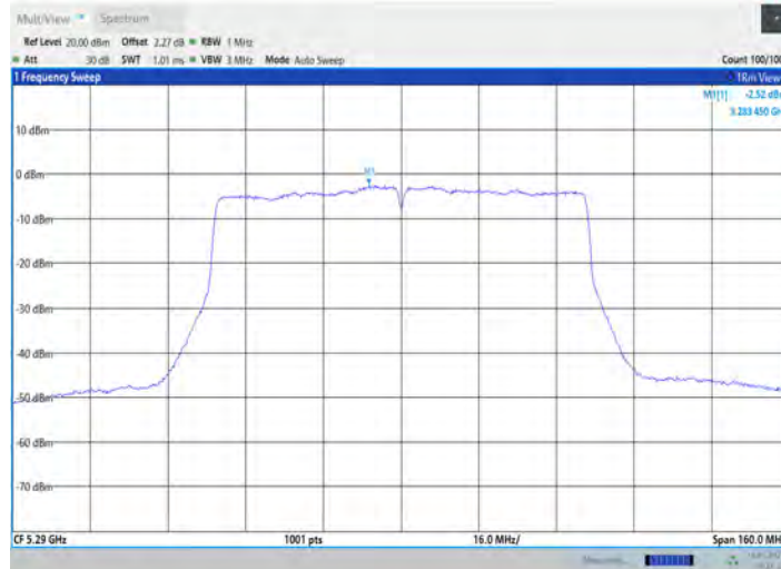
11AC80SISO_Ant7_5290
