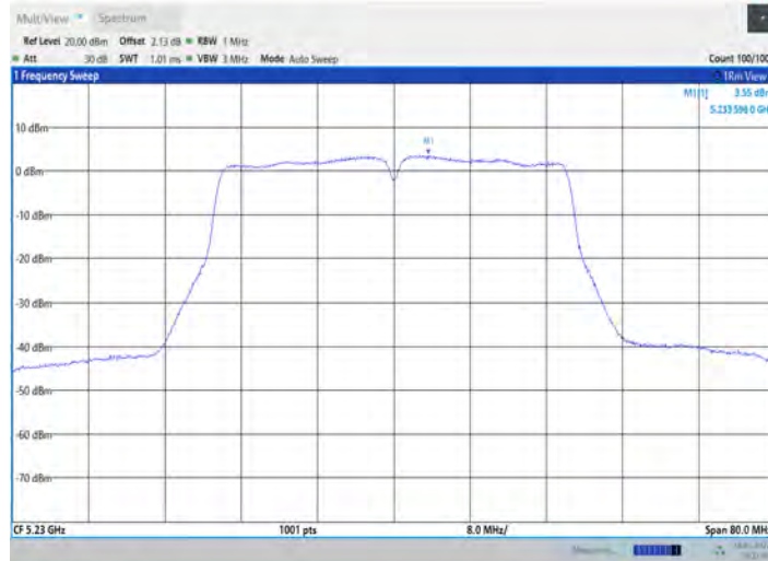
11N40SISO_Ant7_5230
