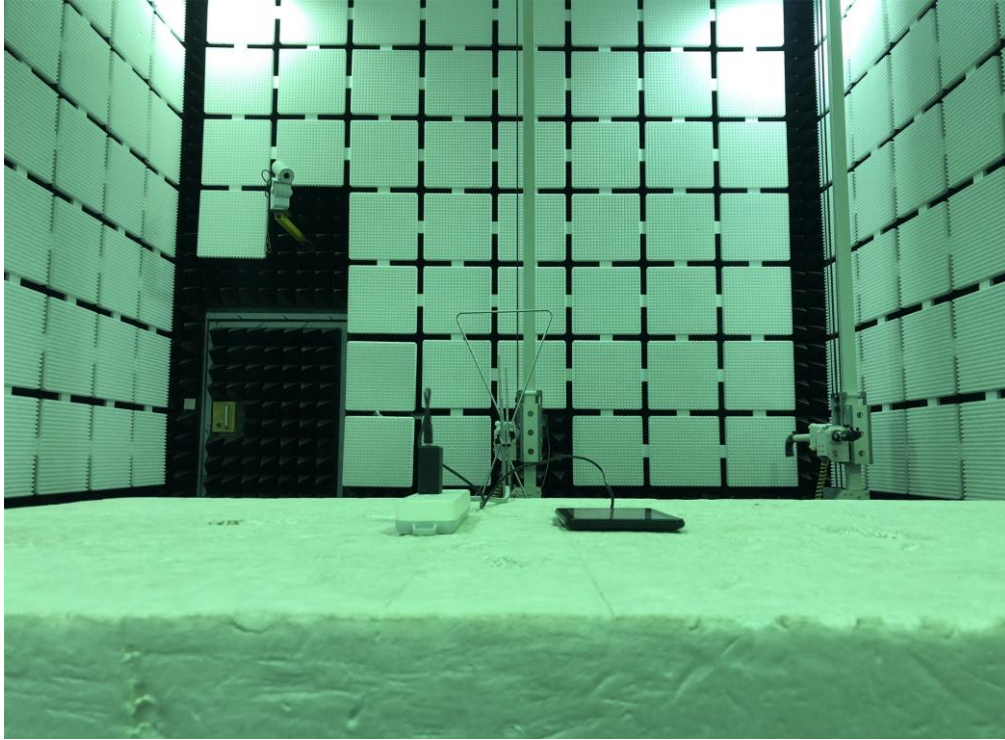
Fig. 1 (Below 1GHz)
