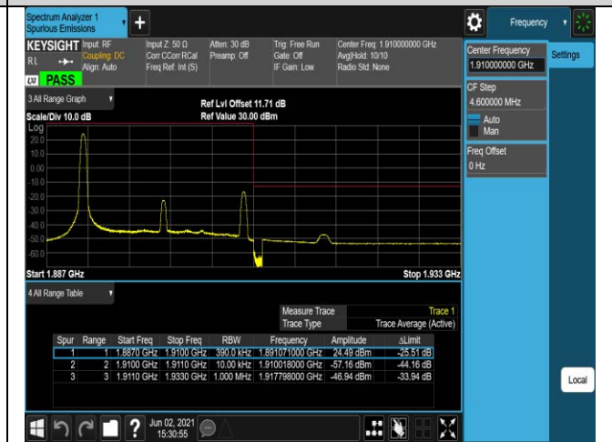
Band2-20MHz-QPSK-19100-100RB#0
