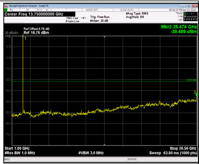
Band7-5MHz-QPSK-21425-1RB#0-Range2:1000~26500MHz
