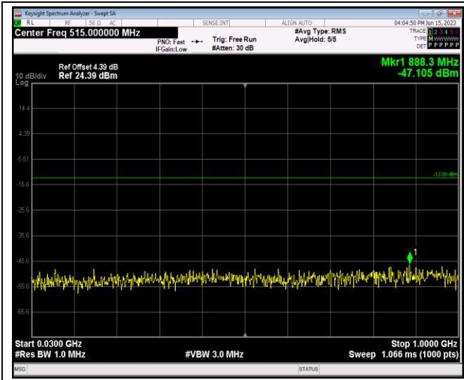
Band4-20MHz-QPSK-20050-1RB#0-Range1:30~100 OMHz
