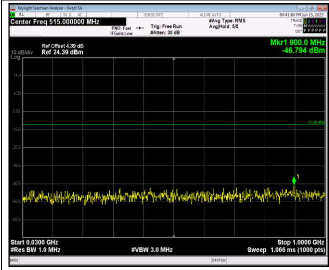
Band4-20MHz-QPSK-20175-1RB#0-Range1:30~100 OMHz
