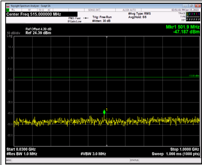
Band2-20MHz-QPSK-19100-1RB#0-Range1:30~100 0MHz
