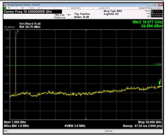
Band4-20MHz-QPSK-20050-1RB#0-Range2:1000~20000MHz
