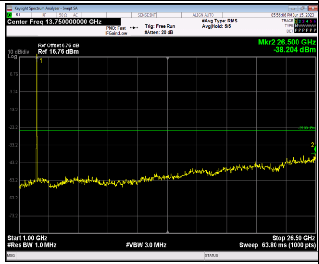
Band7-20MHz-QPSK-21350-1RB#0-Range2:1000~26500MHz
