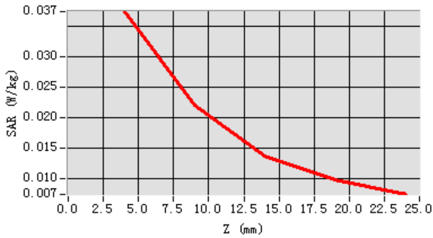
SAR, Z Axis Scan (X = -3, Y = -44)
