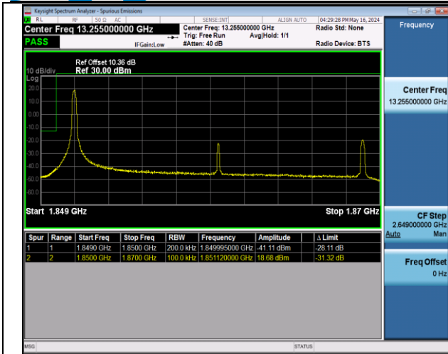
Band2_20MHz_QPSK_18700_1RB#0
