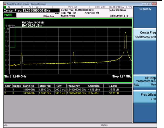
Band2_20MHz_QPSK_18700_1RB#99
