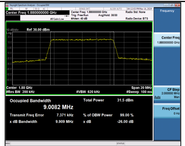
Band2-10MHz-QPSK-18900-50RB#0-PASS
