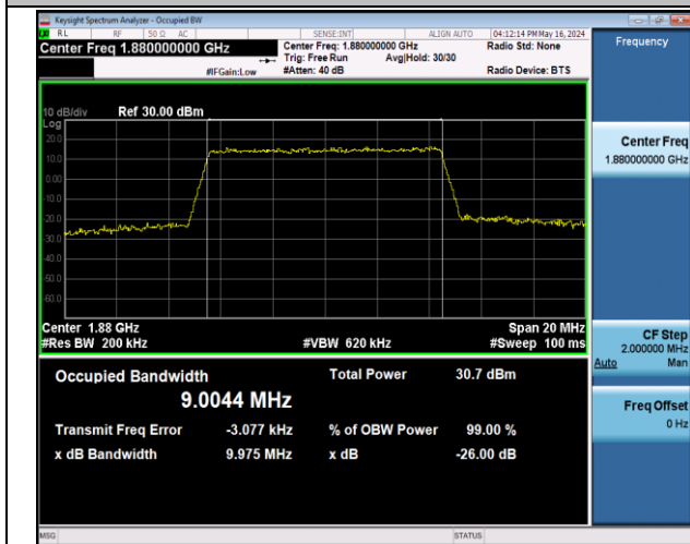
Band2-10MHz-16QAM-18900-50RB#0-PASS
