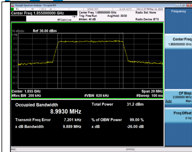
Band2-10MHz-QPSK-18650-50RB#0-PASS
