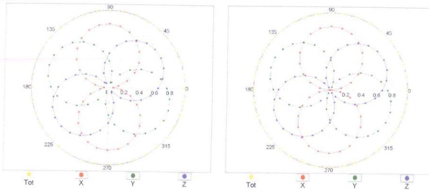
f=1800 MHz,R22
