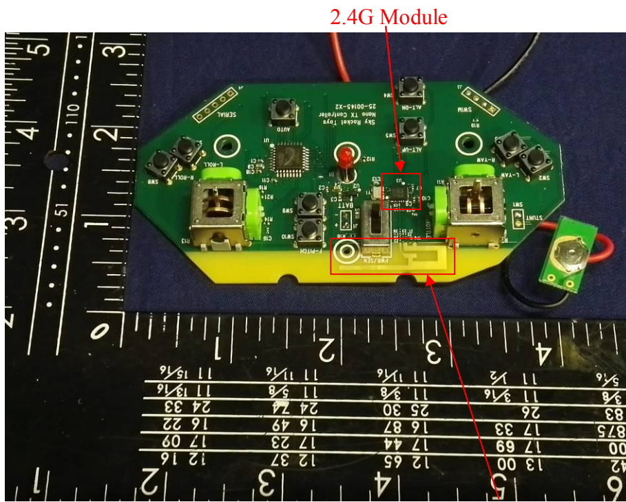
2.4G Antenna
