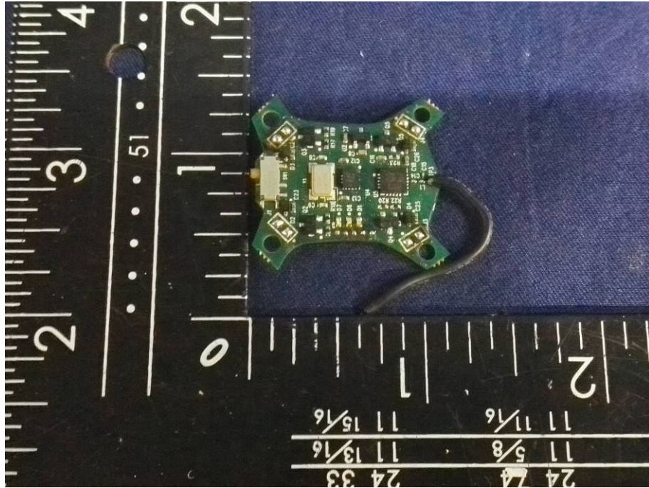
2.4G Module
