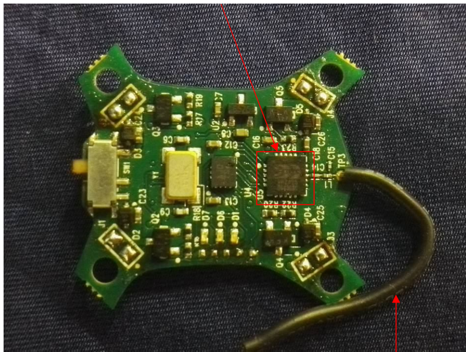
2.4G Antenna
