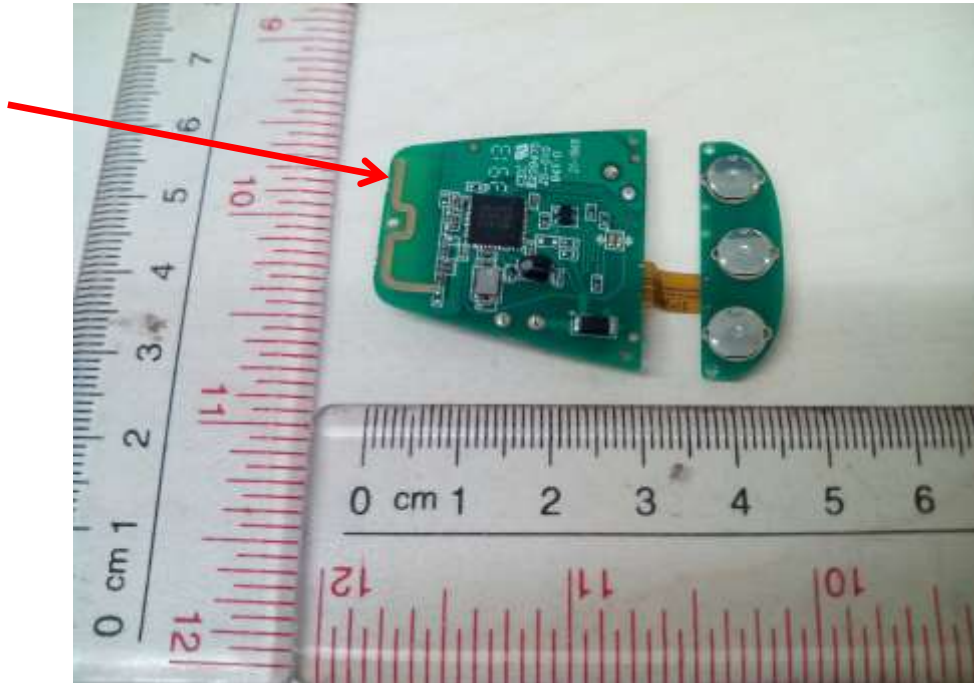
2.4G Antenna
