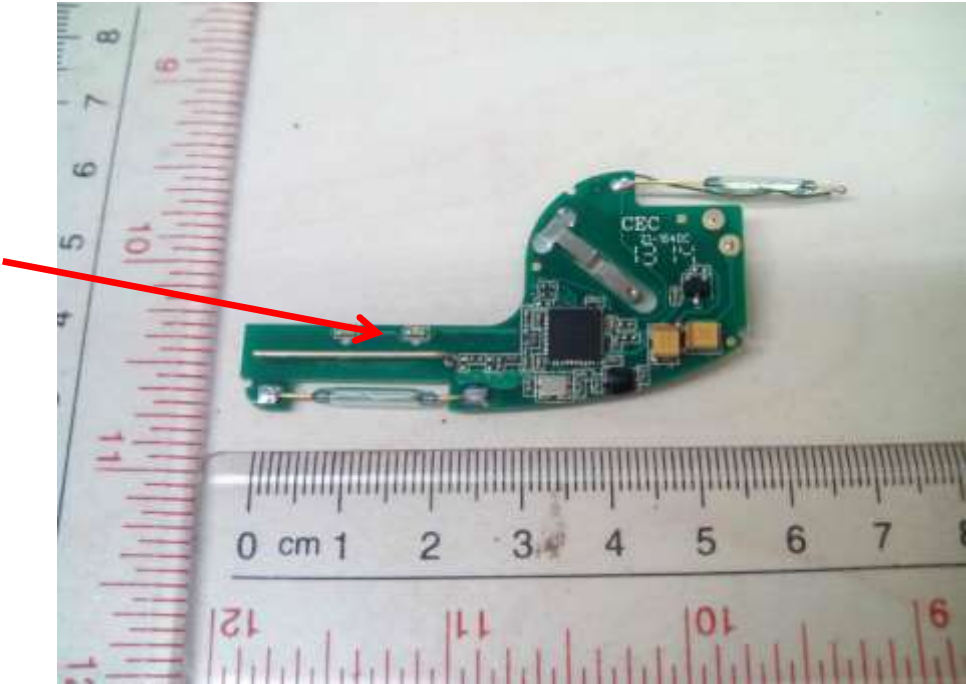
2.4G Antenna
