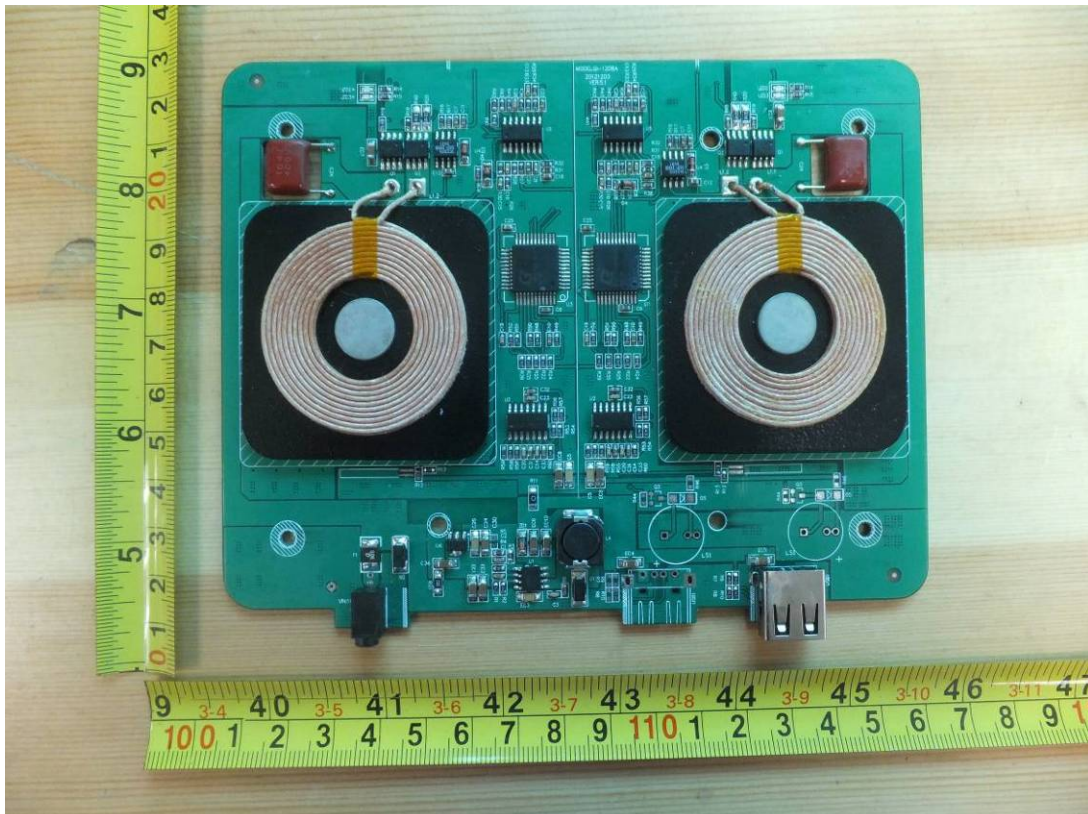
(2) EUT Photo
