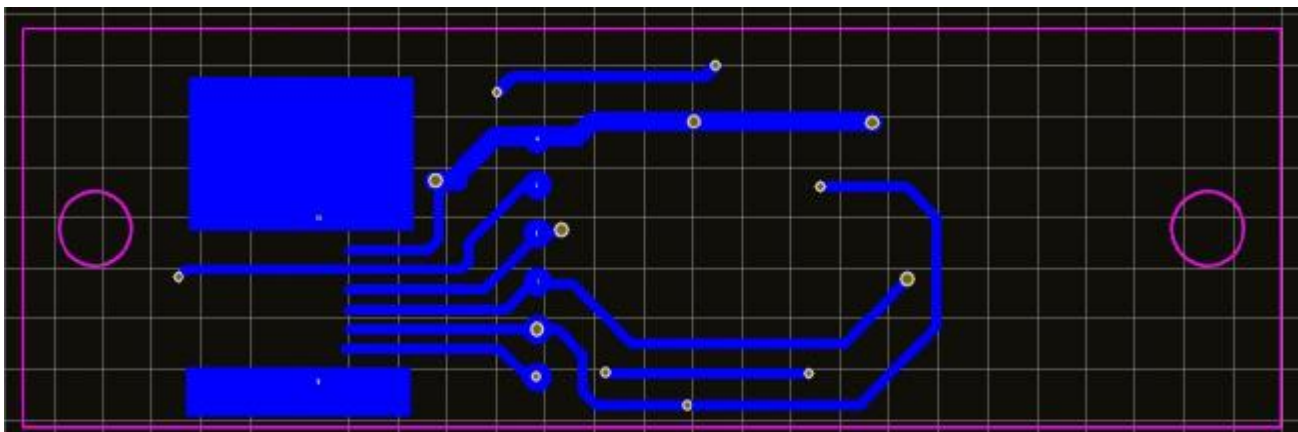
BH-1301A Bottom layer
