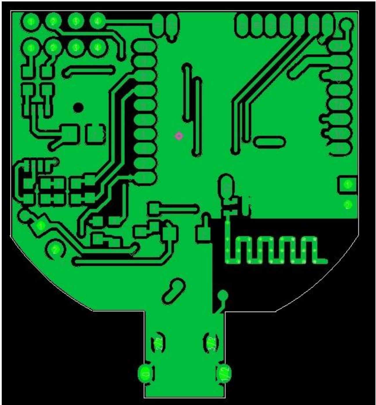
BH-1301A Bottom layer
