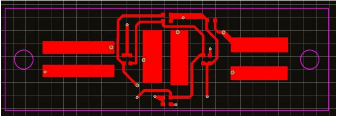
BH-1301A key TOP layer
