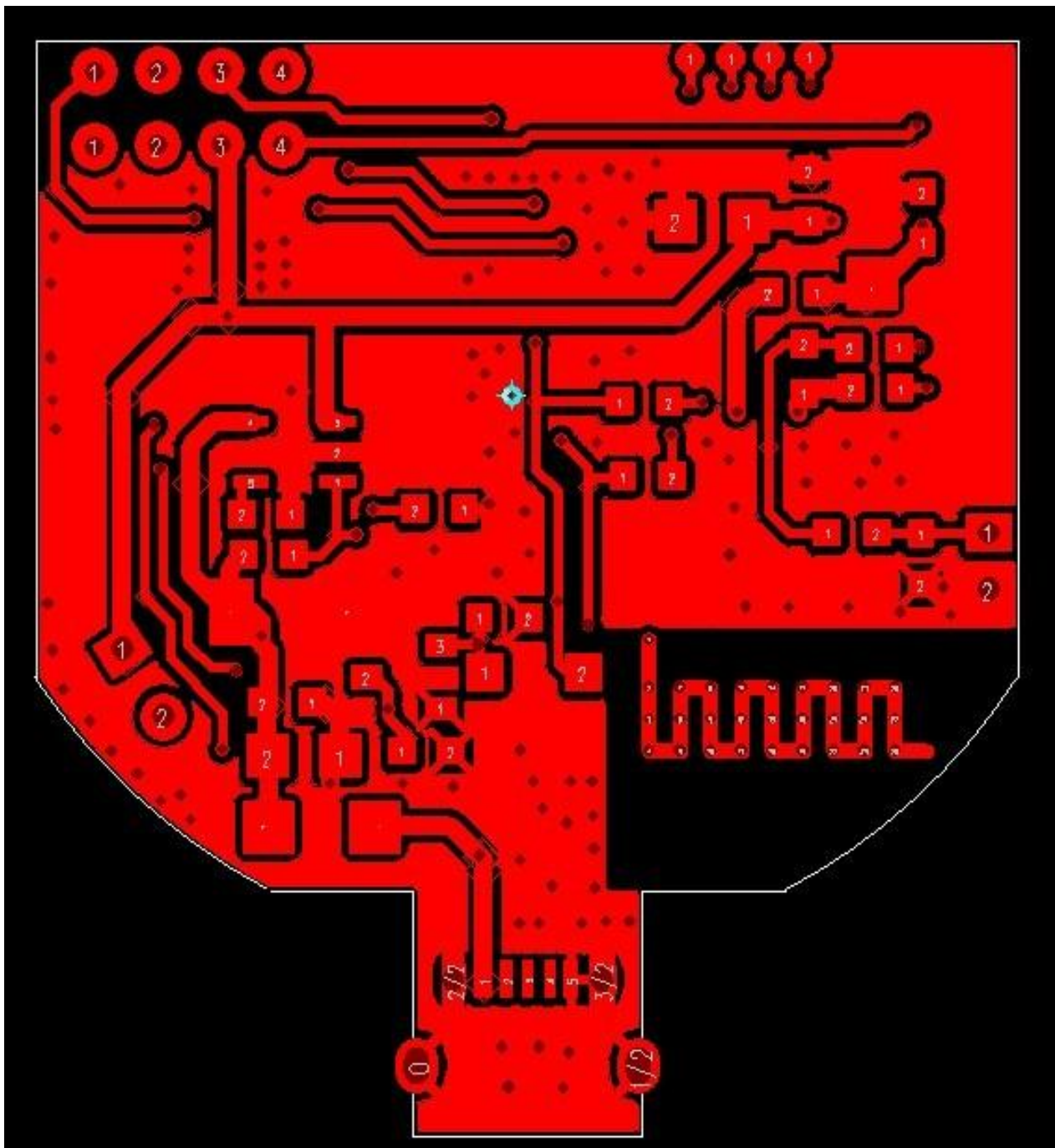
BH-1301A TOP layer
