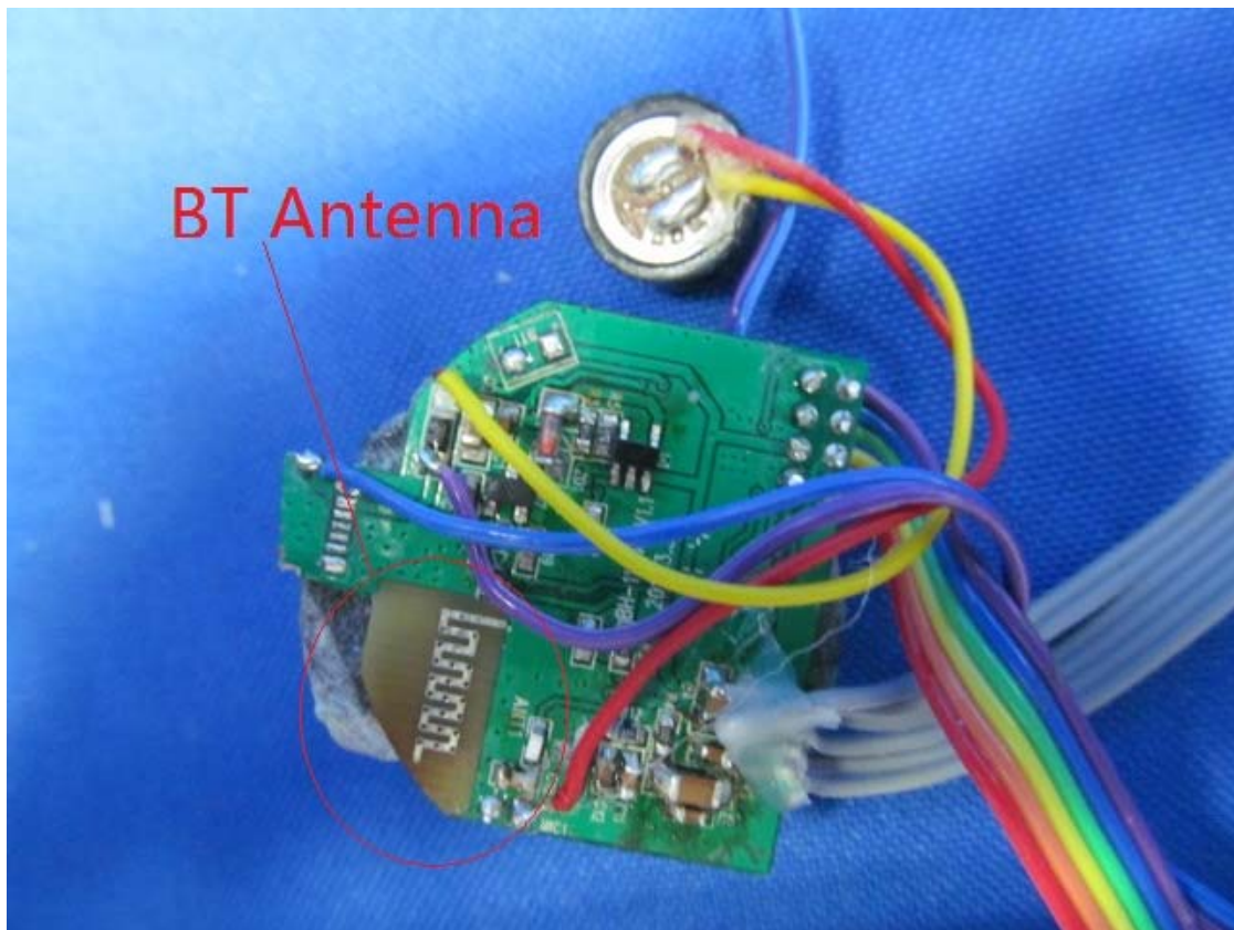
(3) EUT Photo
