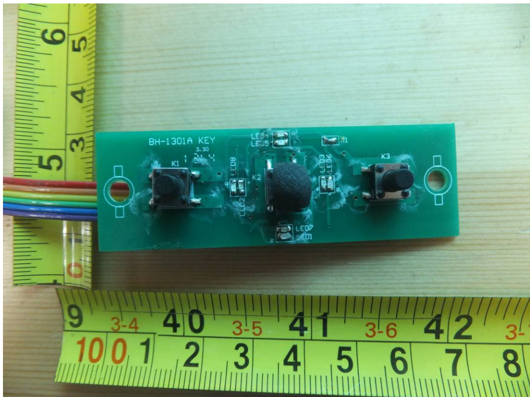
(6) EUT Photo
