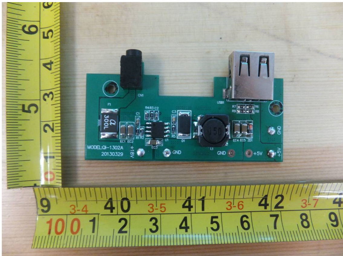
(8) EUT Photo
