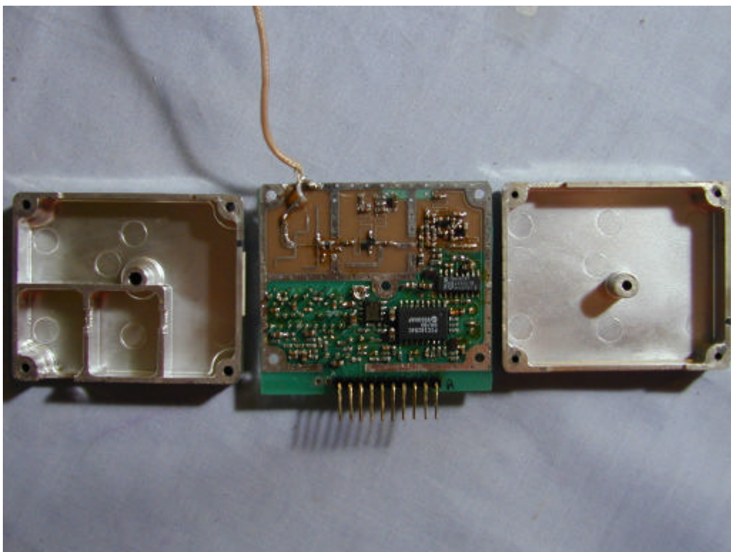
(10) EUT Photo
