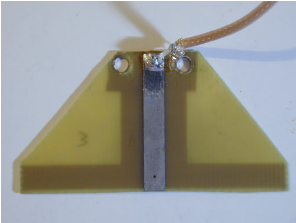
(19) EUT Photo
