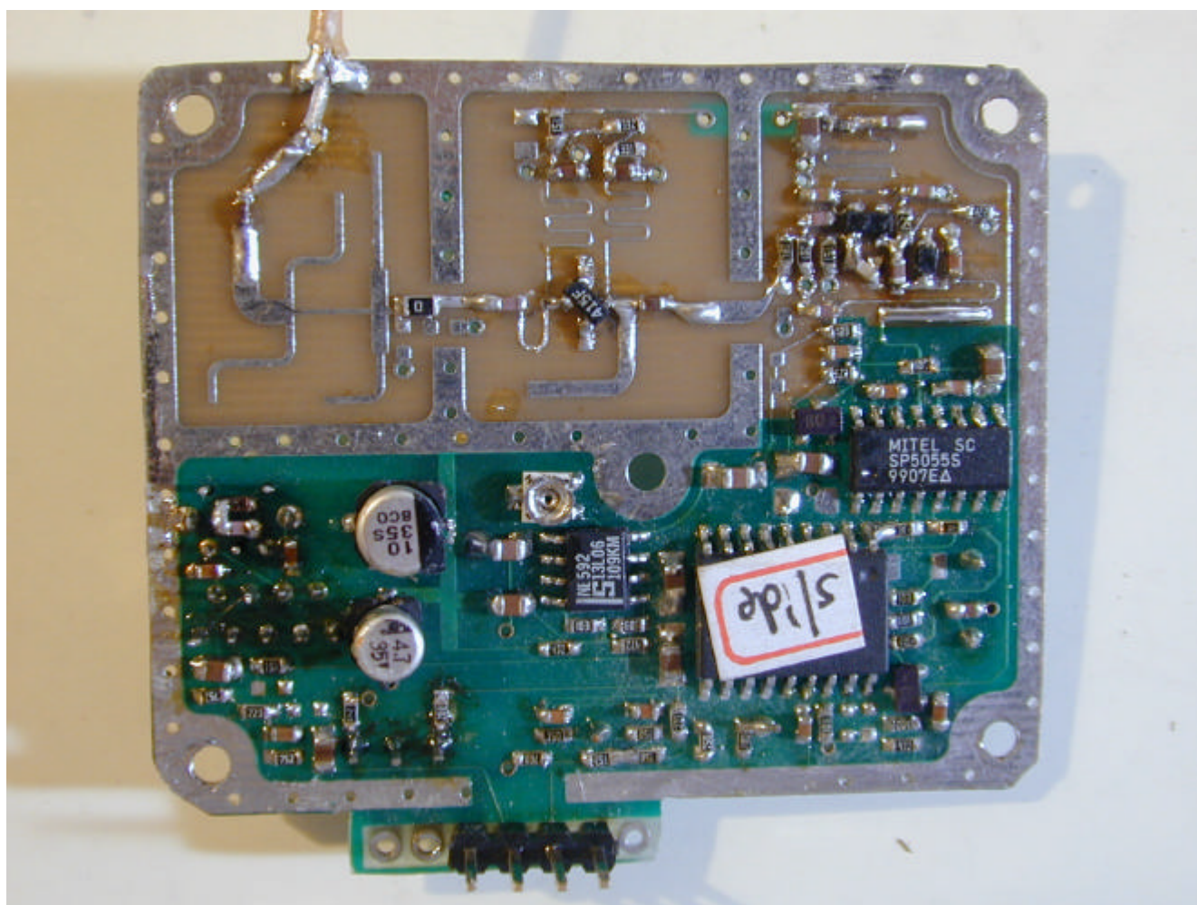
(15) EUT Photo
