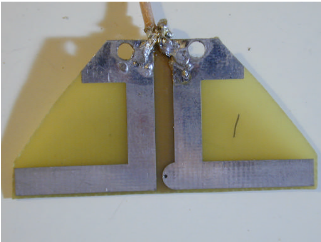
(5) EUT Photo
