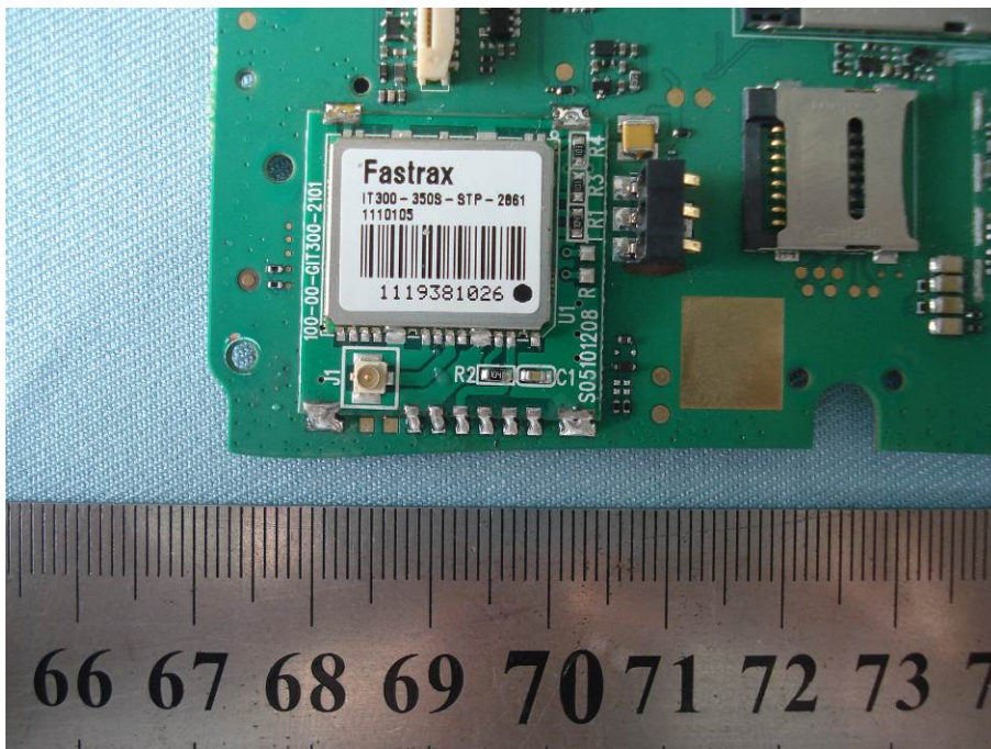
---GPS Module
