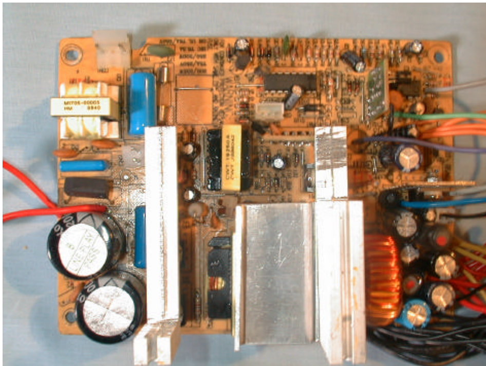
(18) EUT Photo
