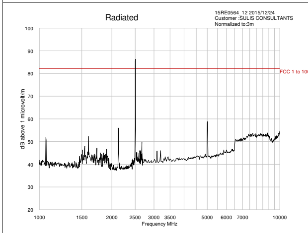
1 – 10 GHz: Low band; bottom
