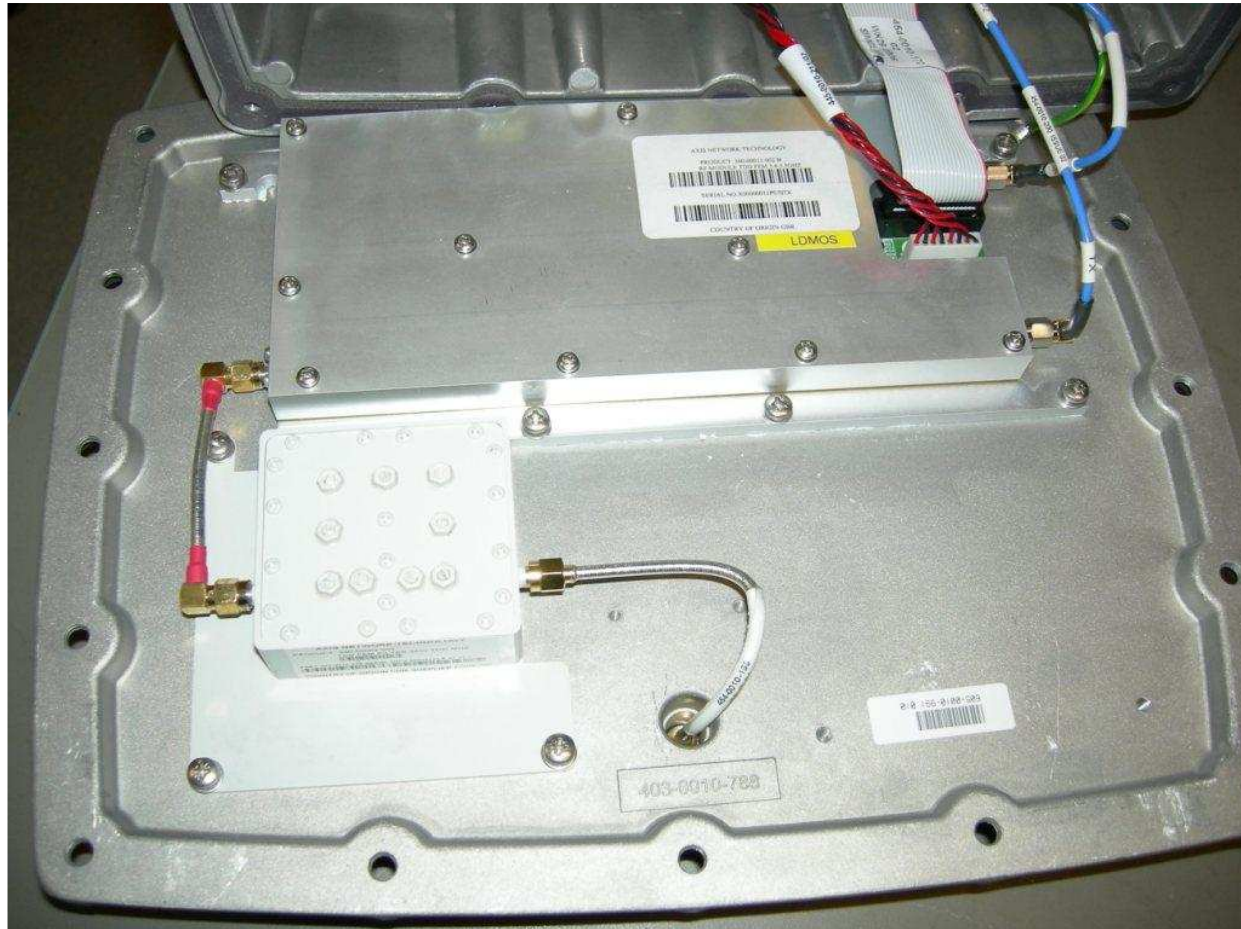
SCRT Front-end module
