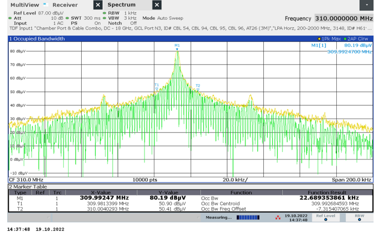
99% BW
