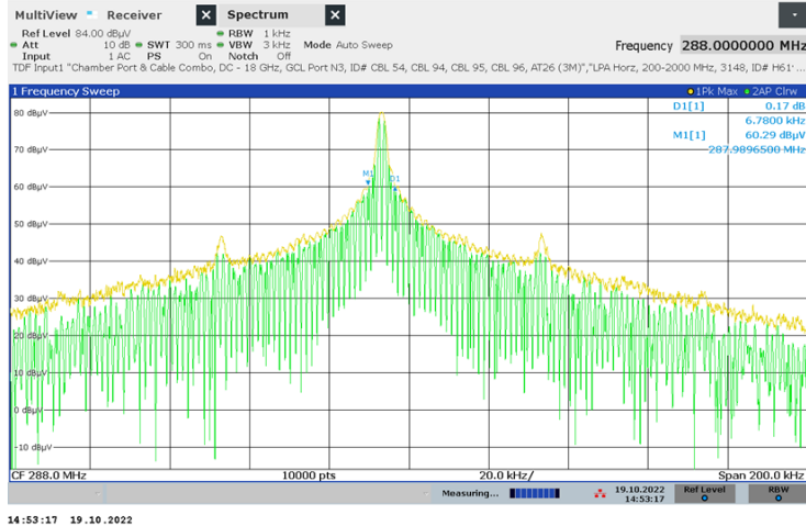
20dB BW
