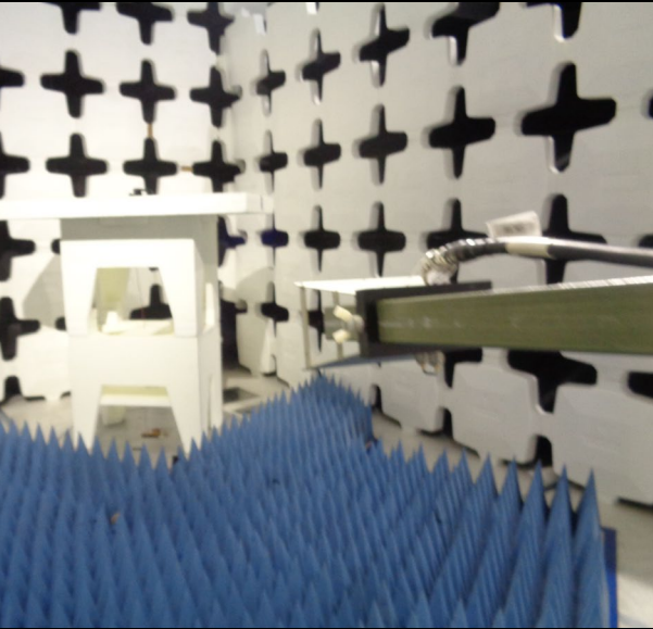
DRWG Horn (1-18GHz) Setup Overview
