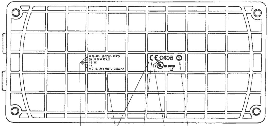
Frontansicht
