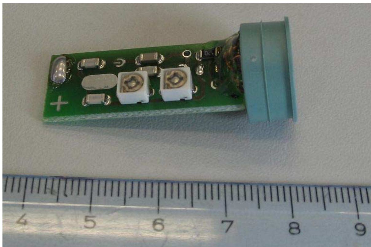
Antenna MOBY E ANT 18
