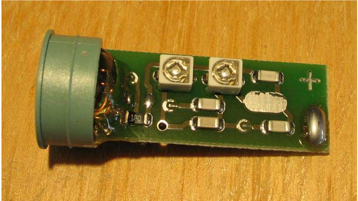
Antenna MOBY E ANT 18
