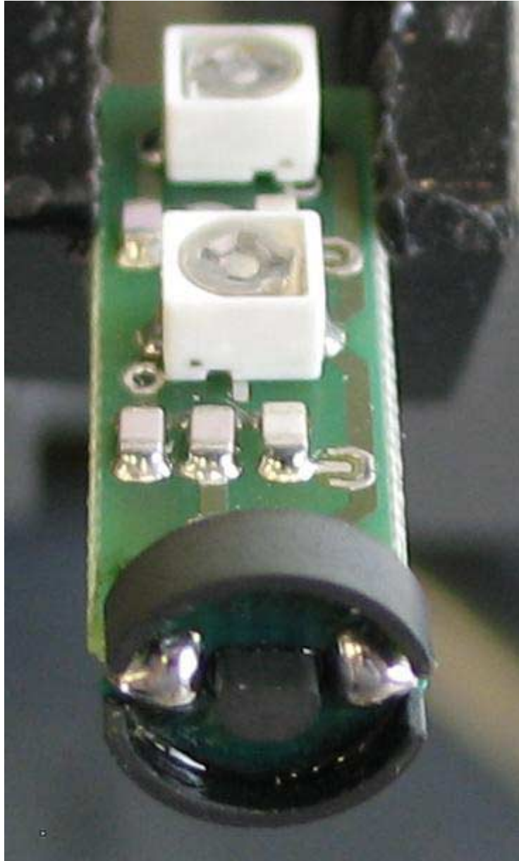
Antenna MOBY E ANT 12
