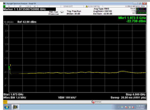
20 MHz QPSK
