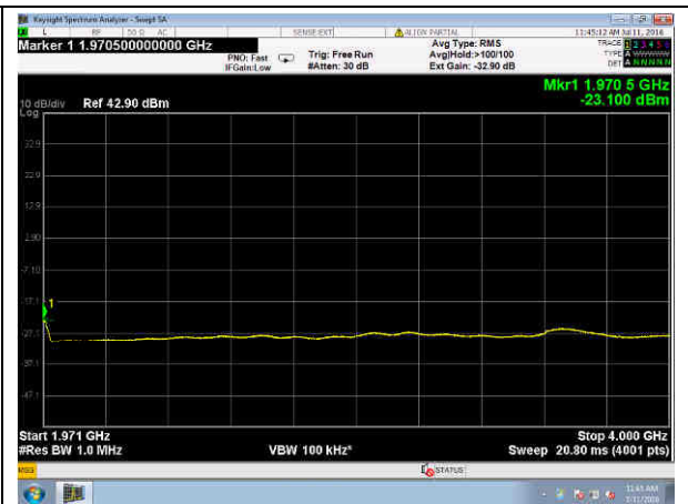
15 MHz QPSK
