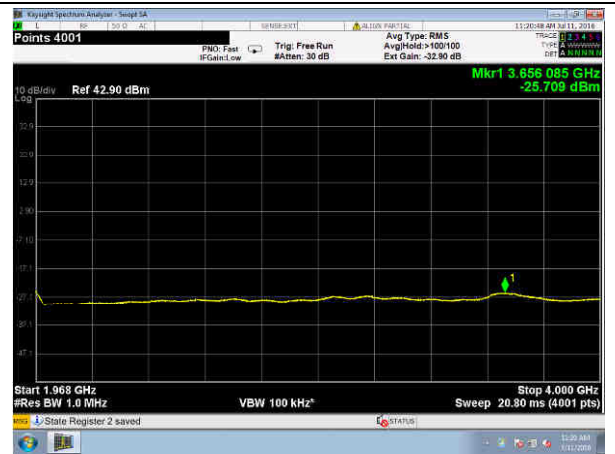
10 MHz QPSK
