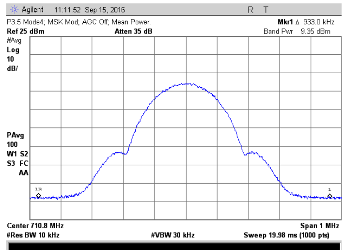
710.8 MHz; MSK; AGC off
