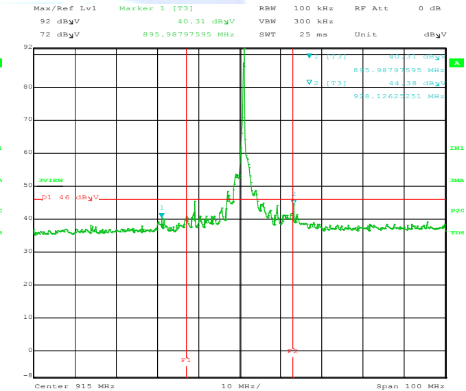
Comment A: Band Edge 916MHz Vertical
