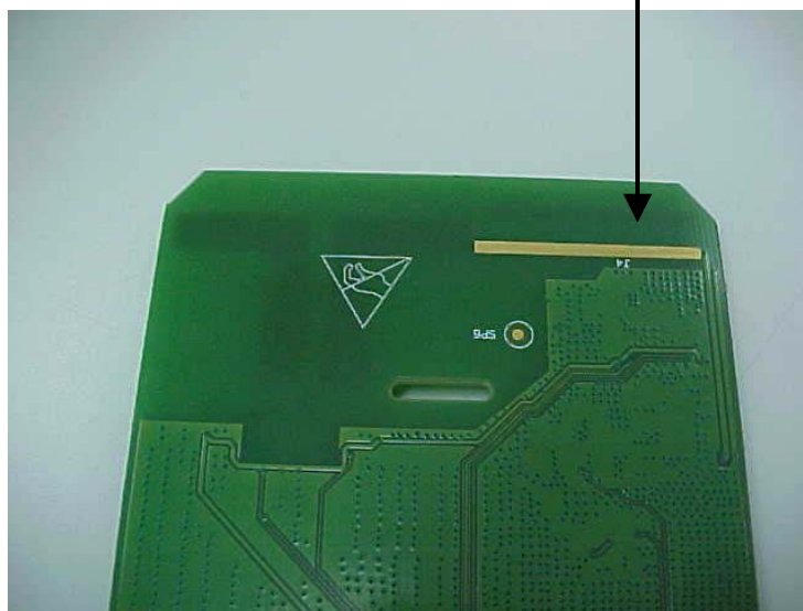
ANT 2.4GHZ
