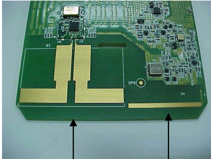
ANT 2.4GHZ
