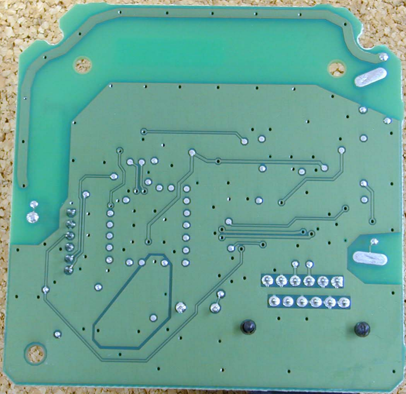
Mini RKE 1126, PCB, Bottom
