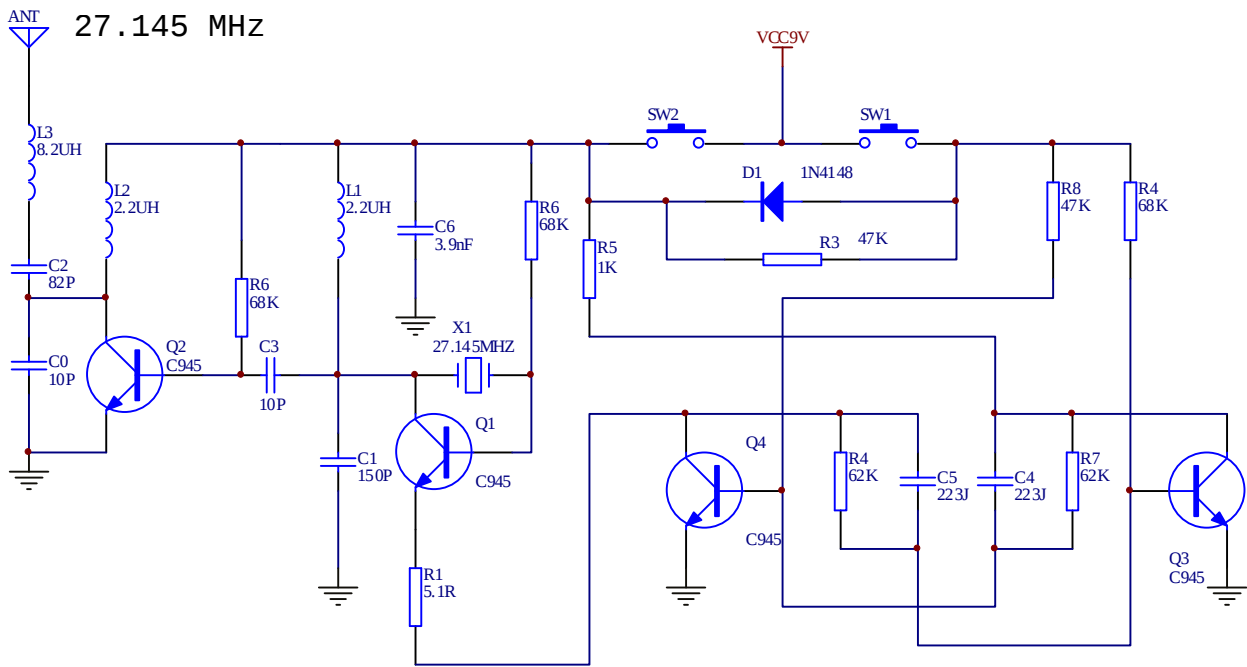
1018T 27M原理图
