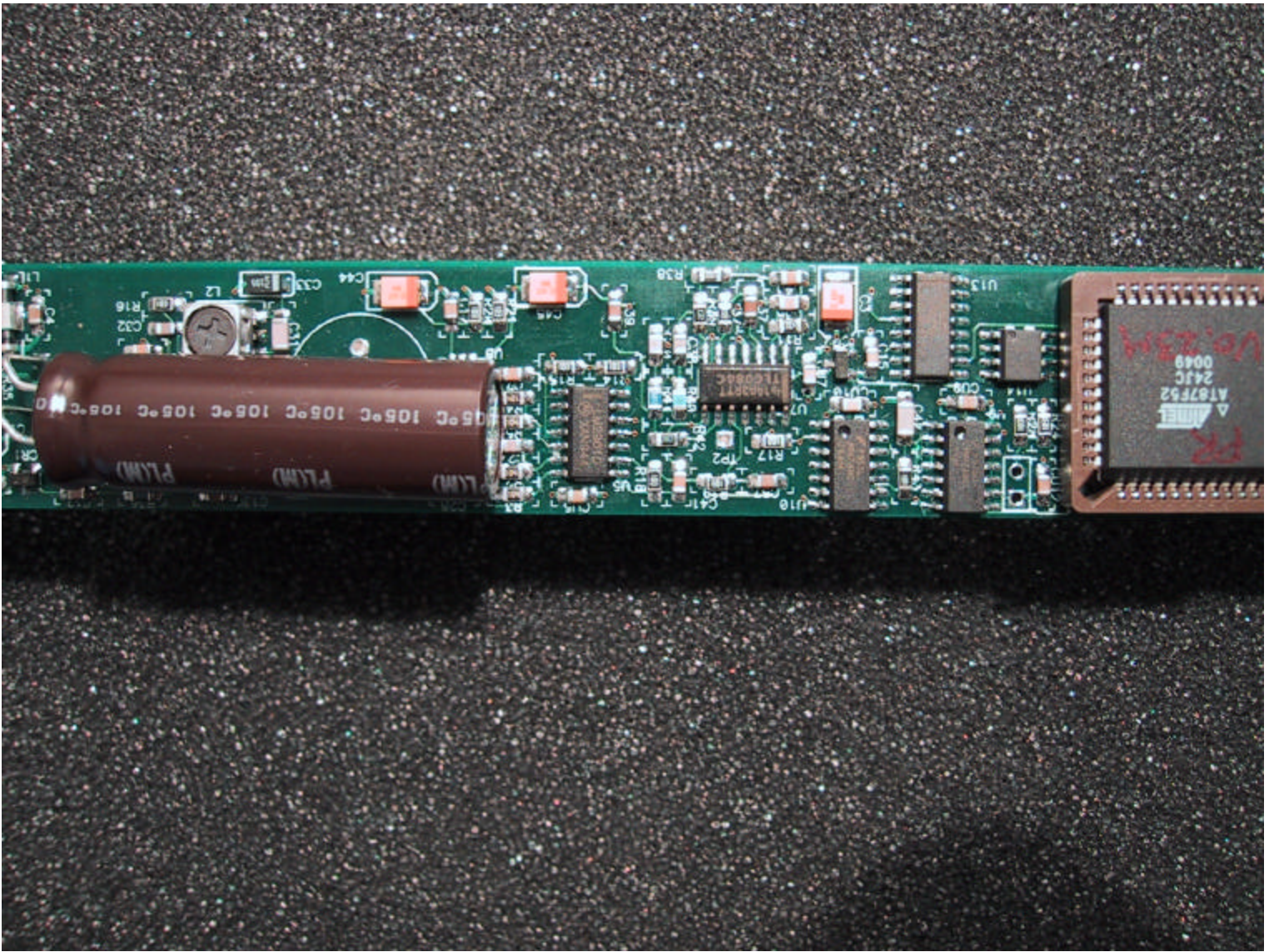
PCB TOP B
